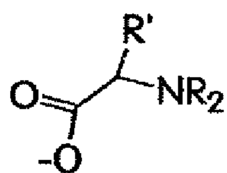
aminoacids
