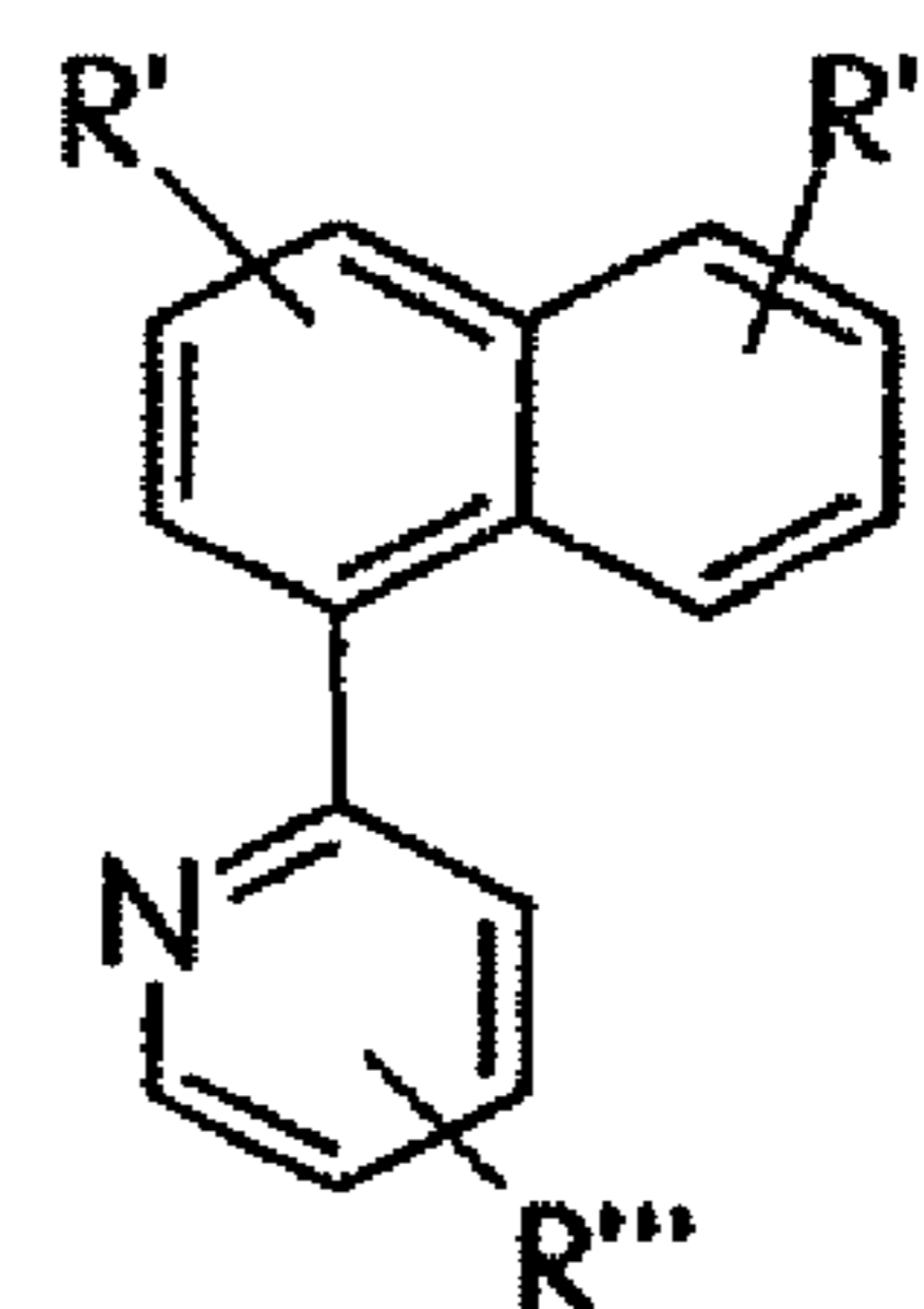
pyridylnaphthalenes
