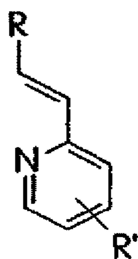
vinylpyridines
