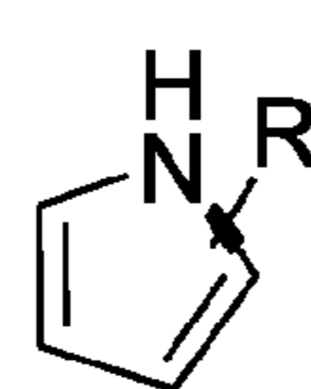
pyrroles
