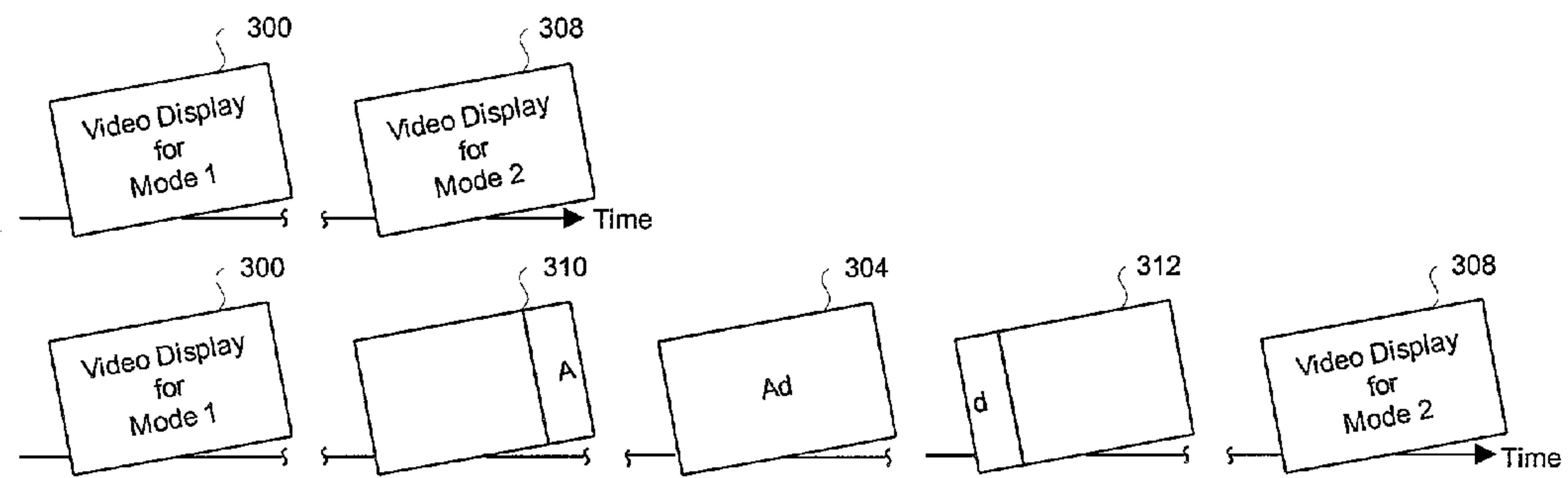
Fig. 3(d) - Transition Ad Placement
