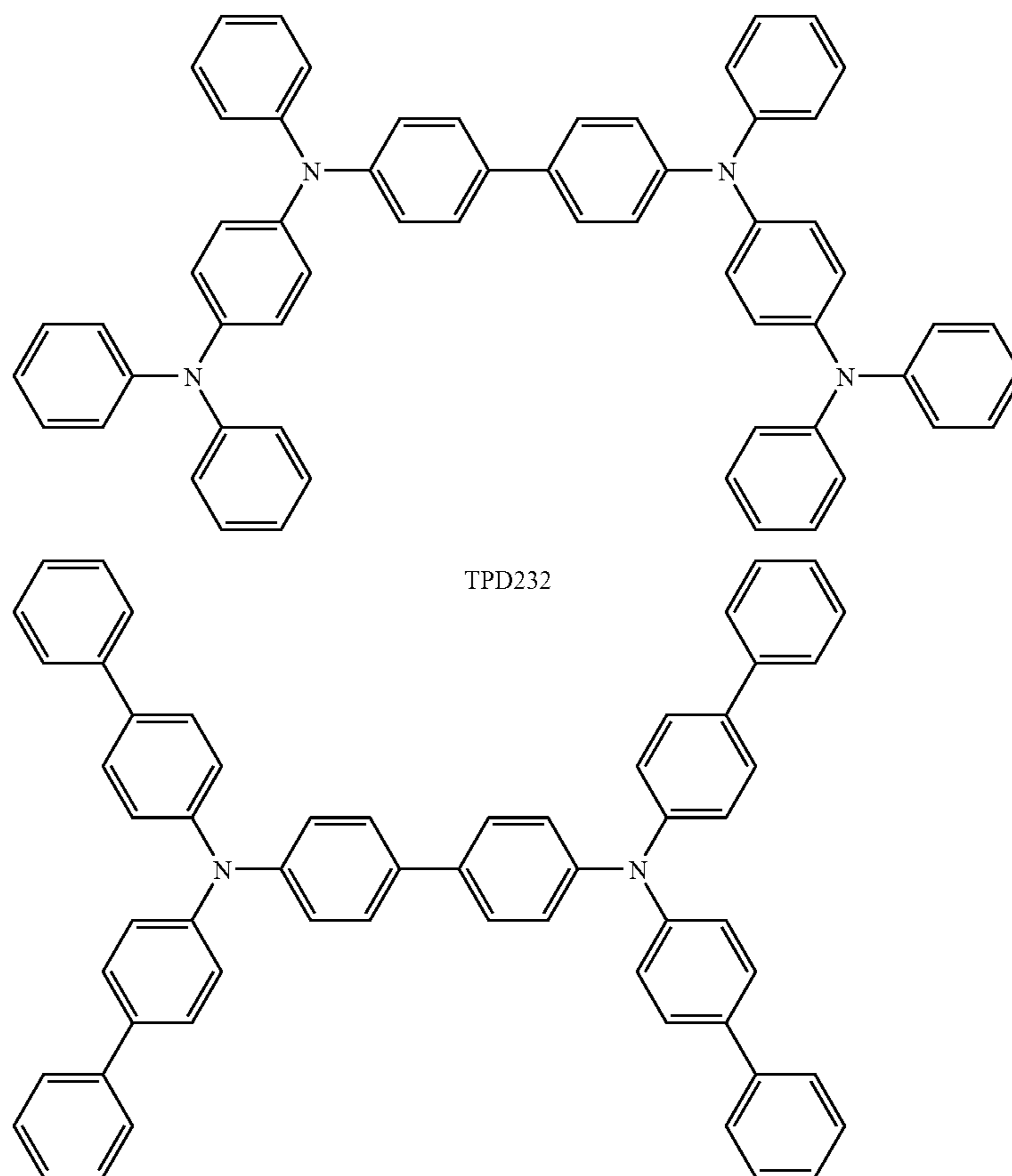
TBDB
