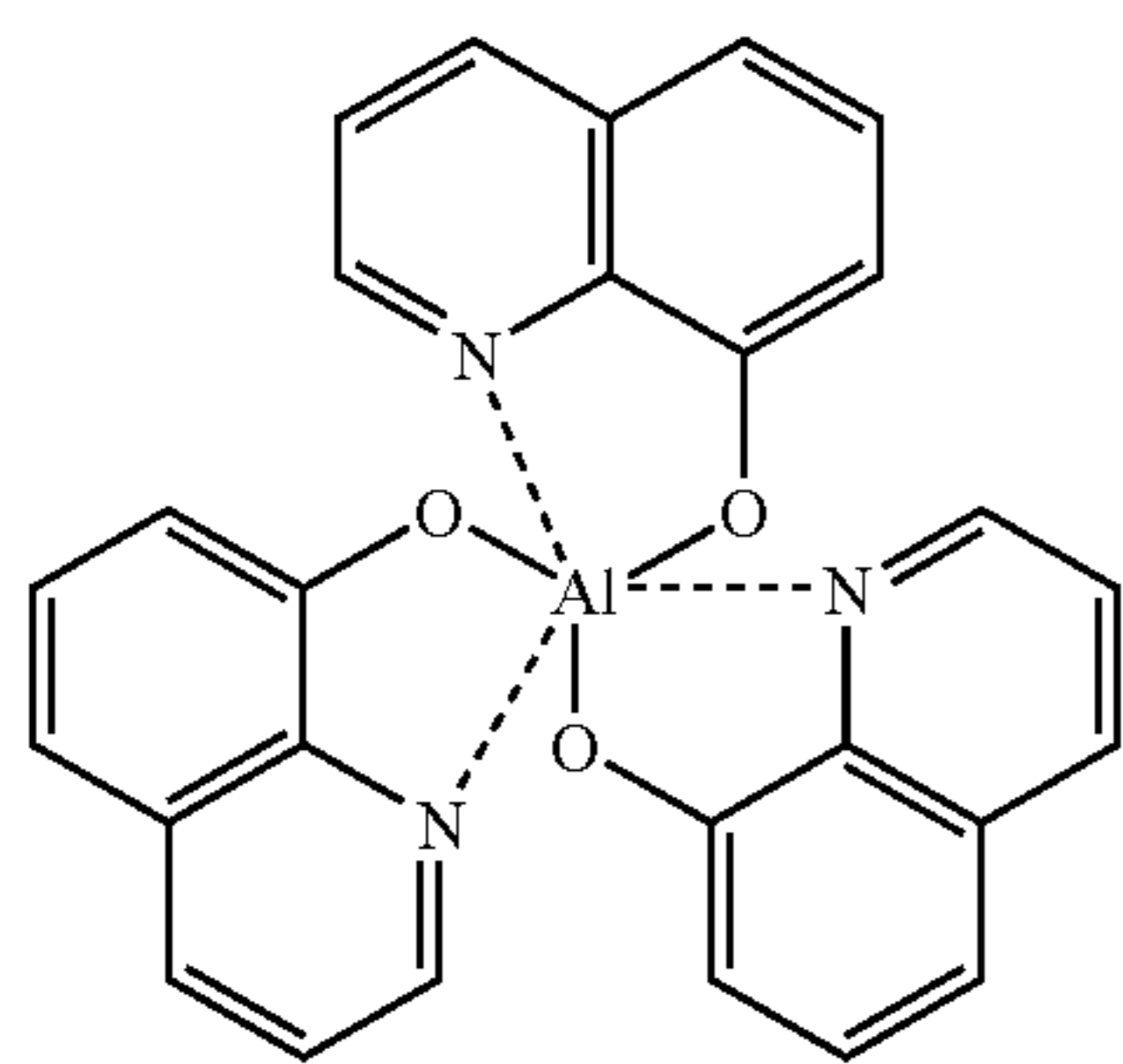
Alq
