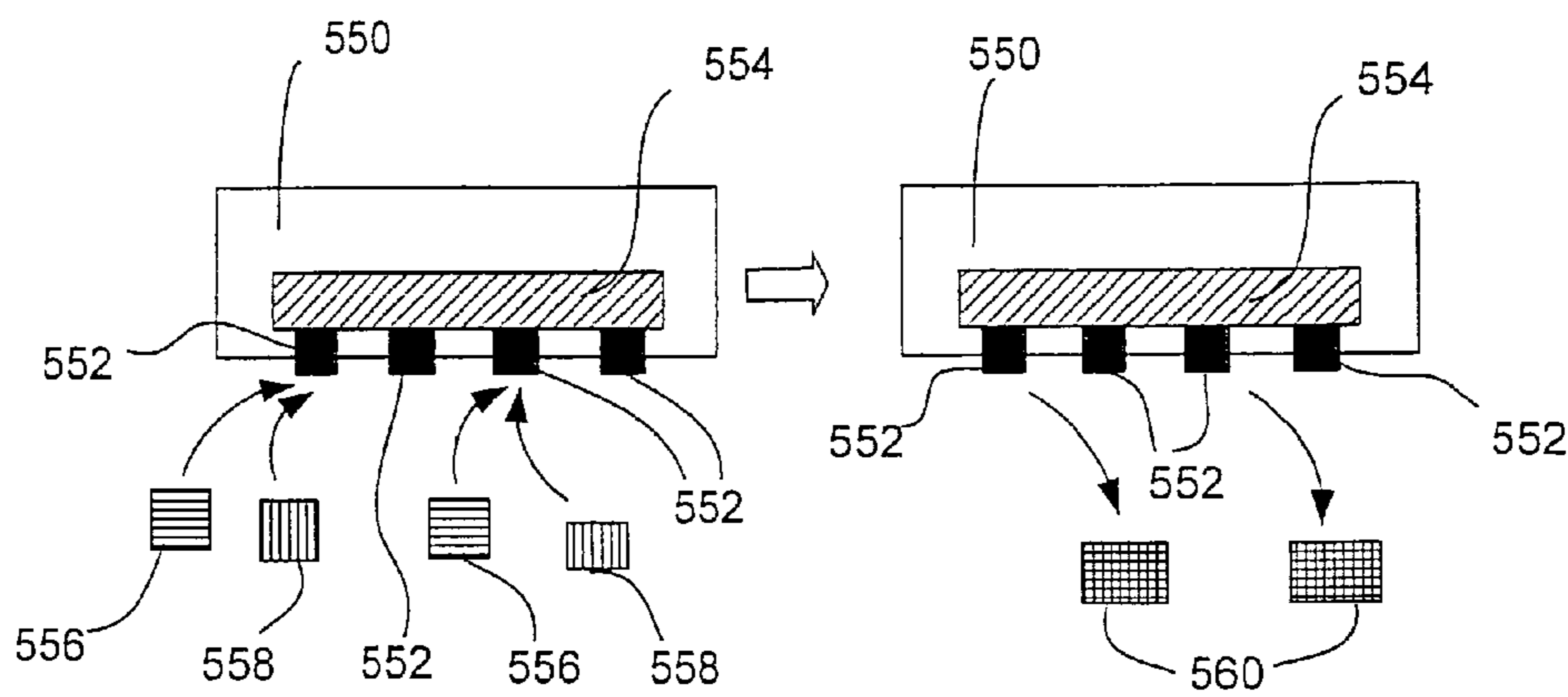
FIG. 17A
