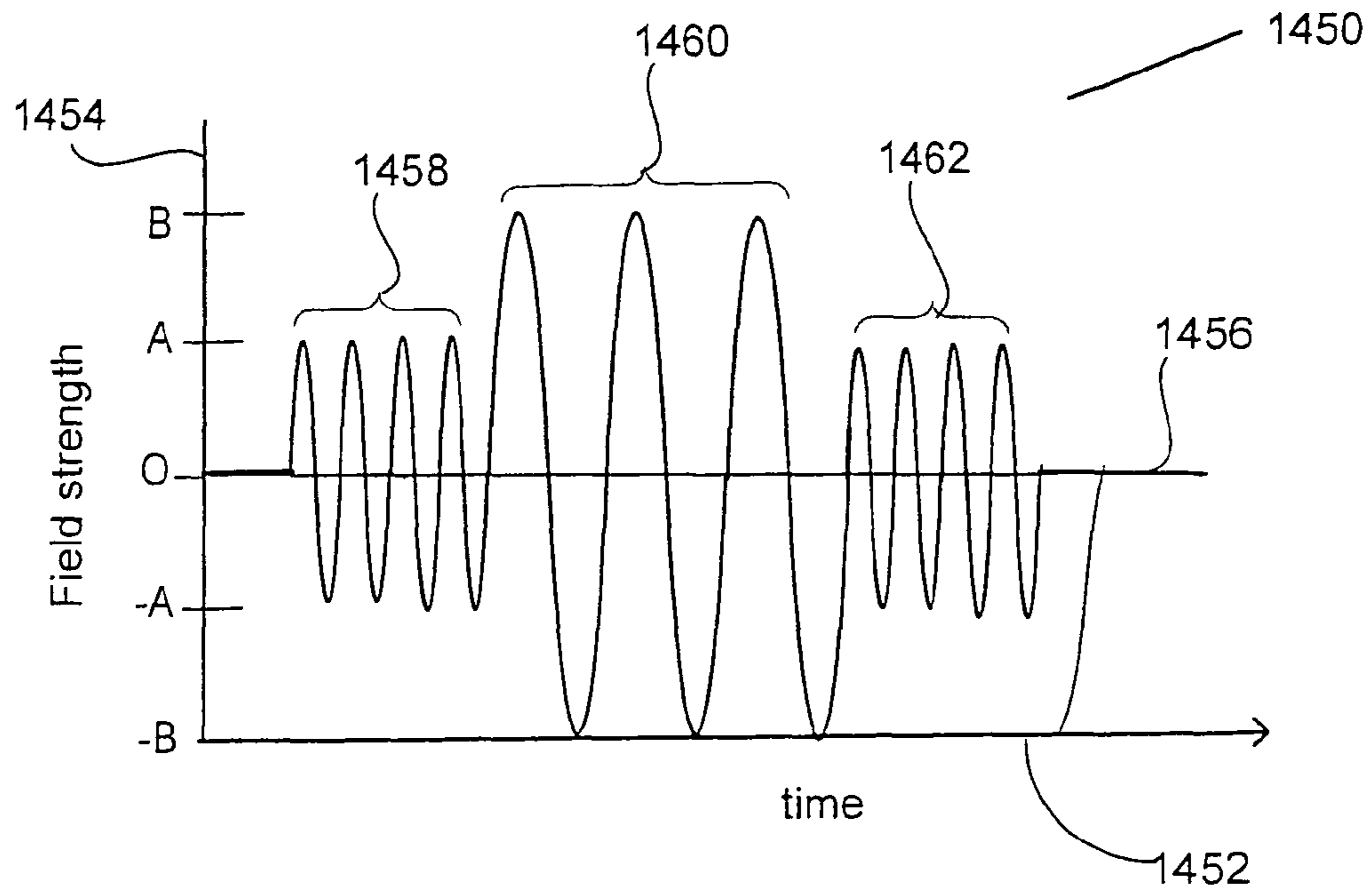
FIG. 40
