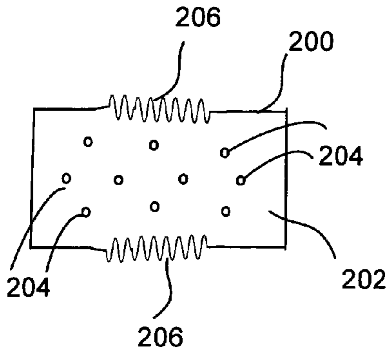
FIG. 9A
