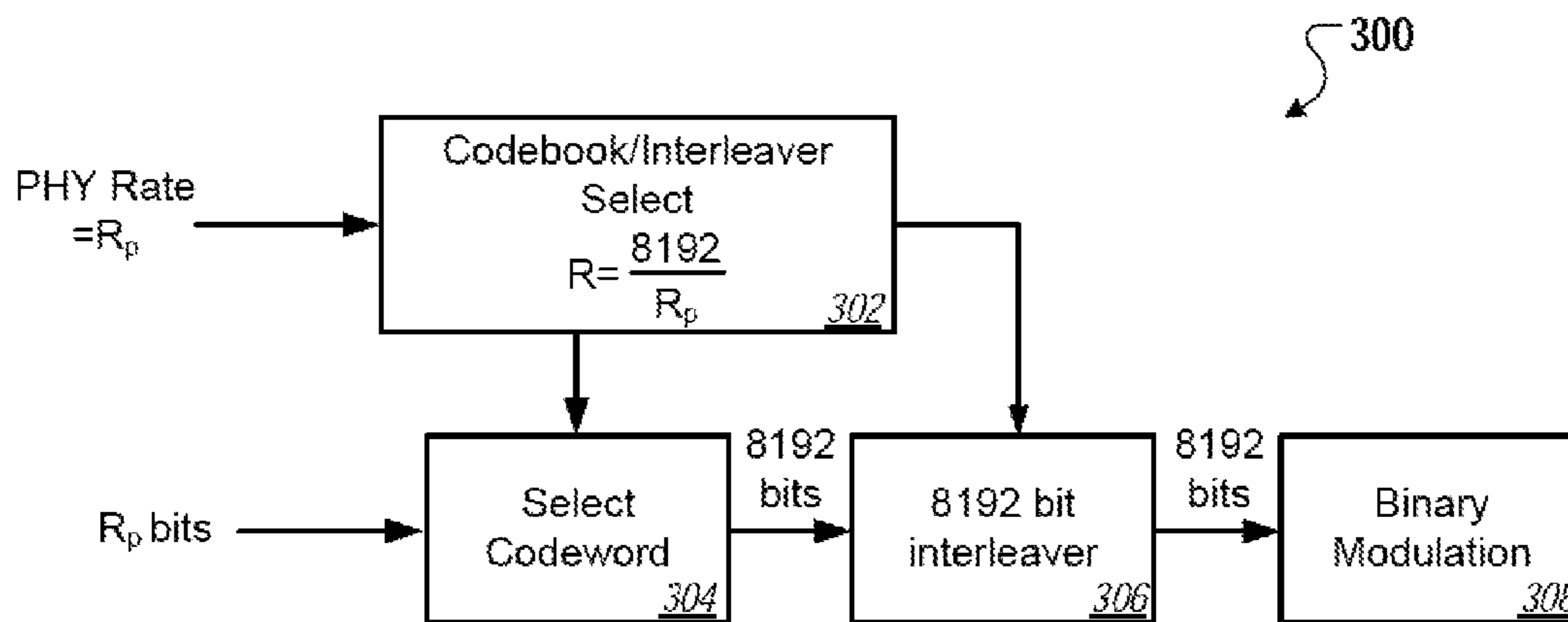
FIG. 3A
