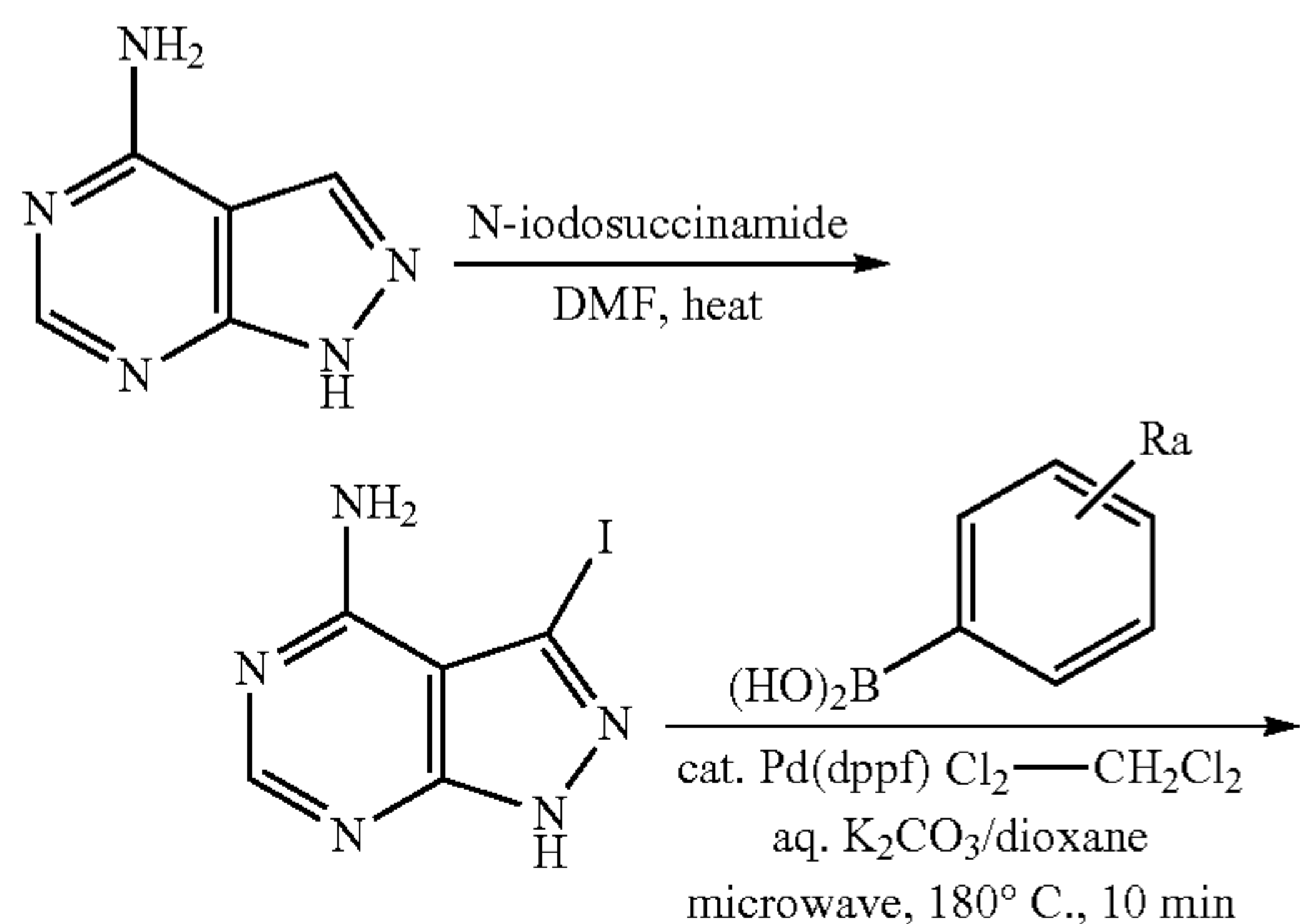
Scheme I.
