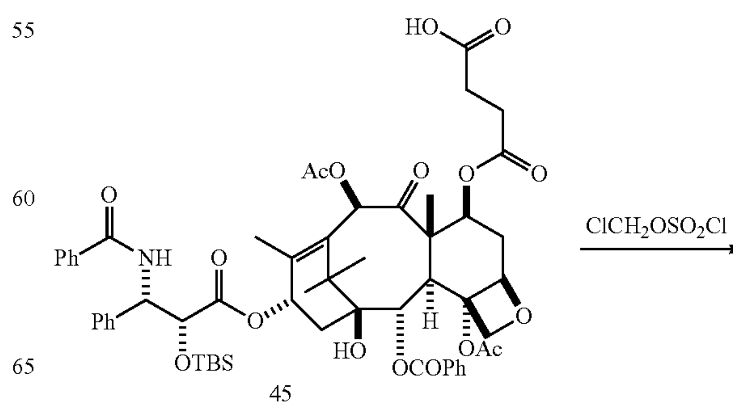
Scheme 10.1
