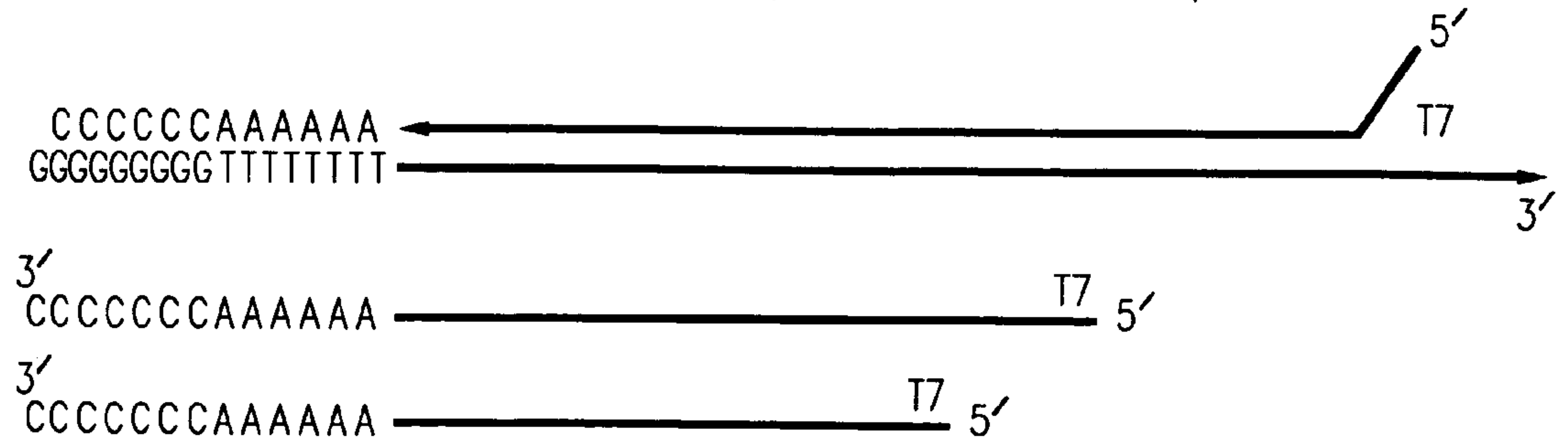
(D) Extension of primers and strand displacement of extended primers
