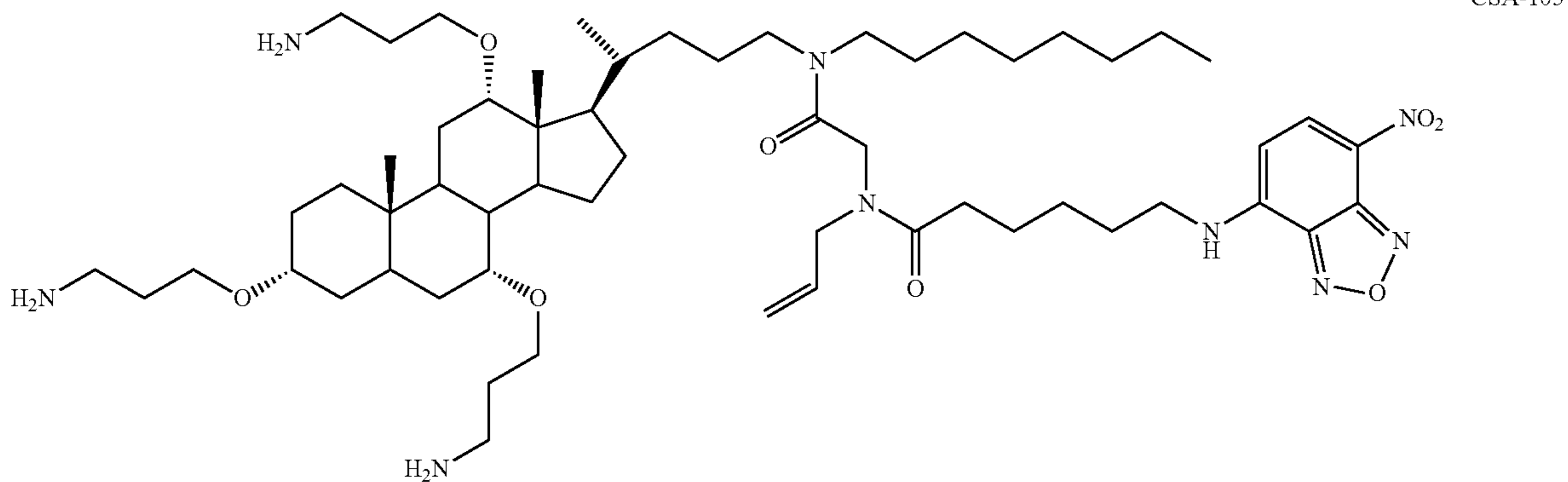
CSA-105 (polymerizable, fluorophore-labeled ceragenin)
