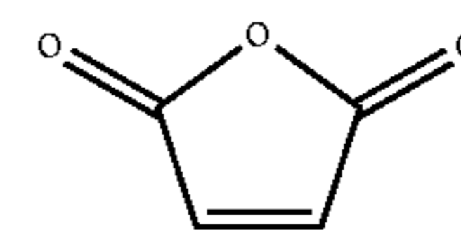
maleic anhydride
