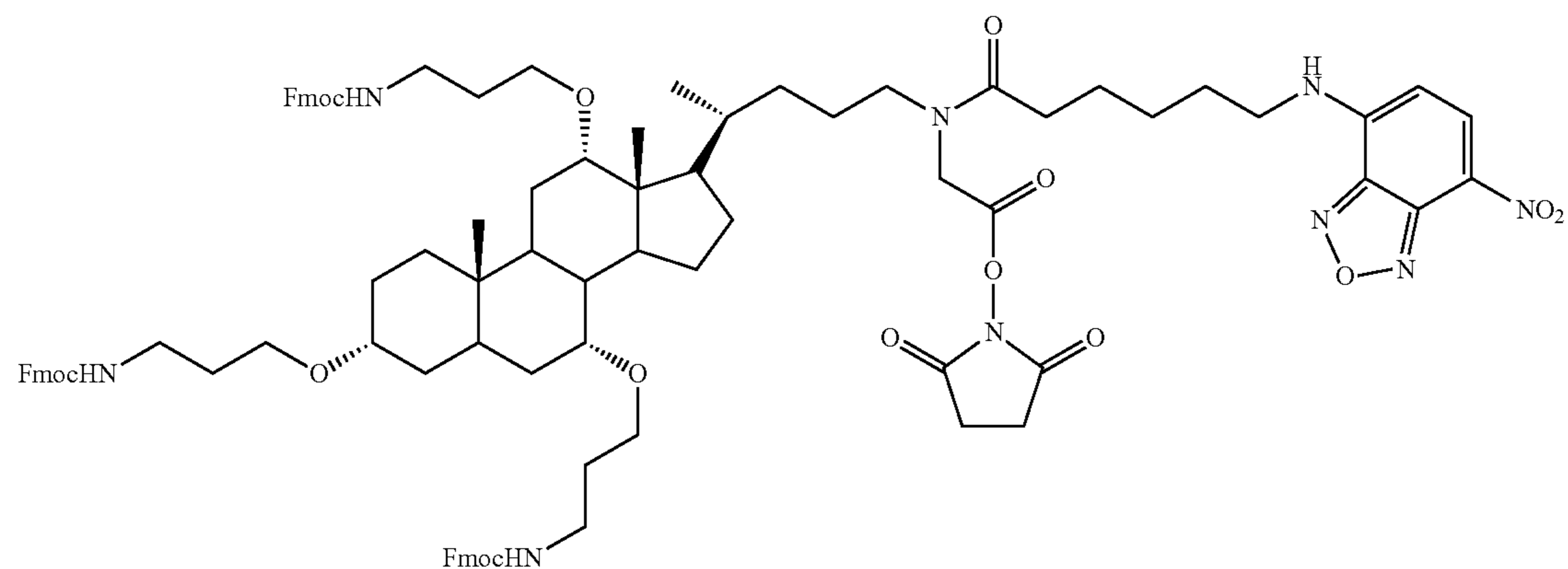
CSA-108
