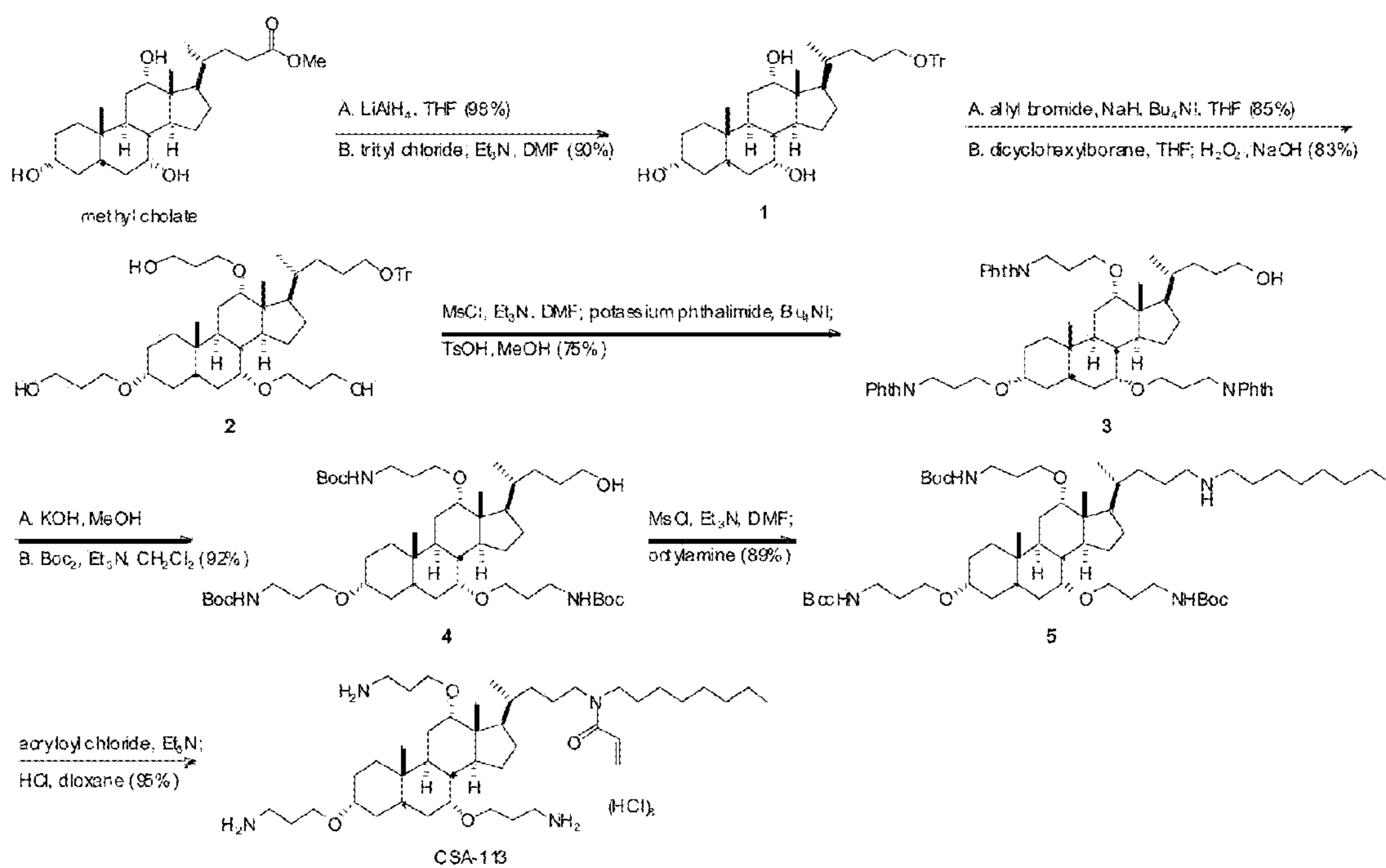
CSA-113 Synthesis Scheme
