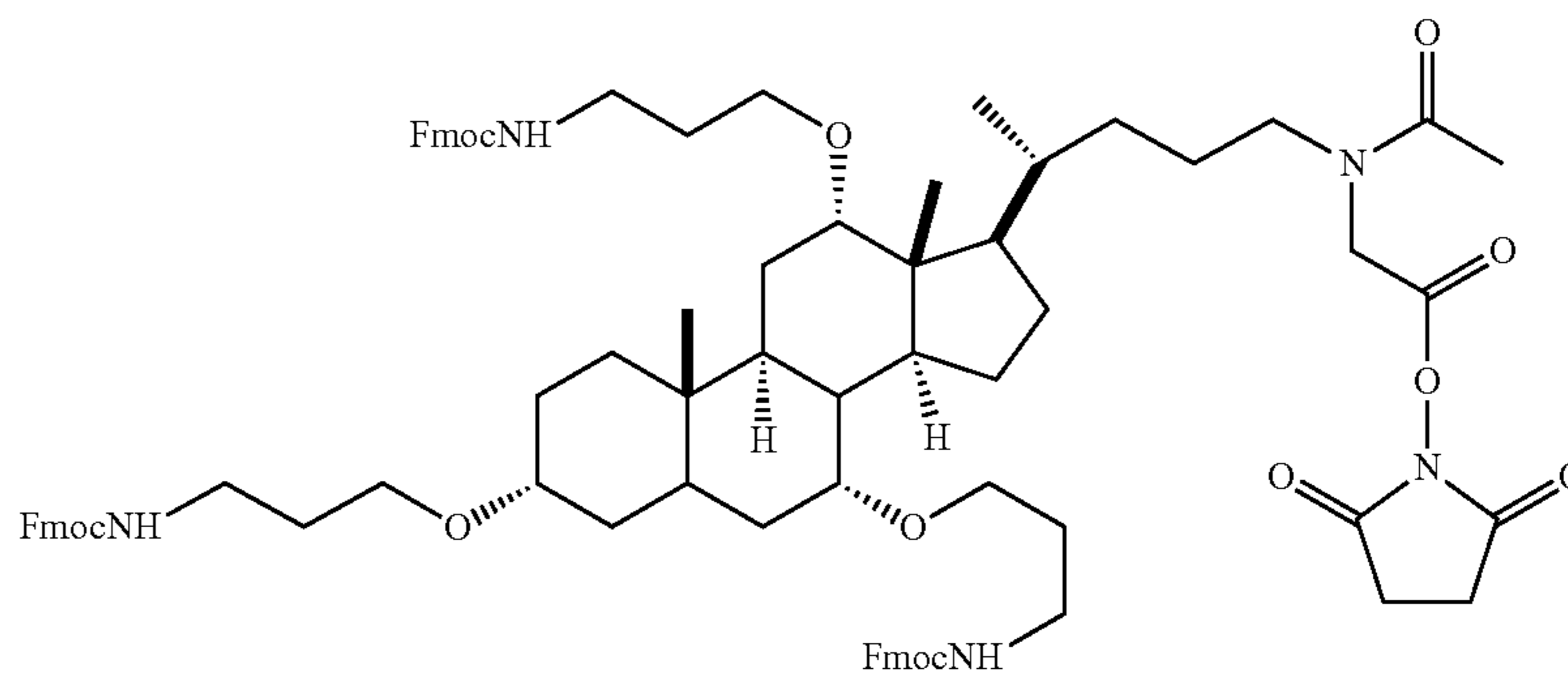
CSA-111
