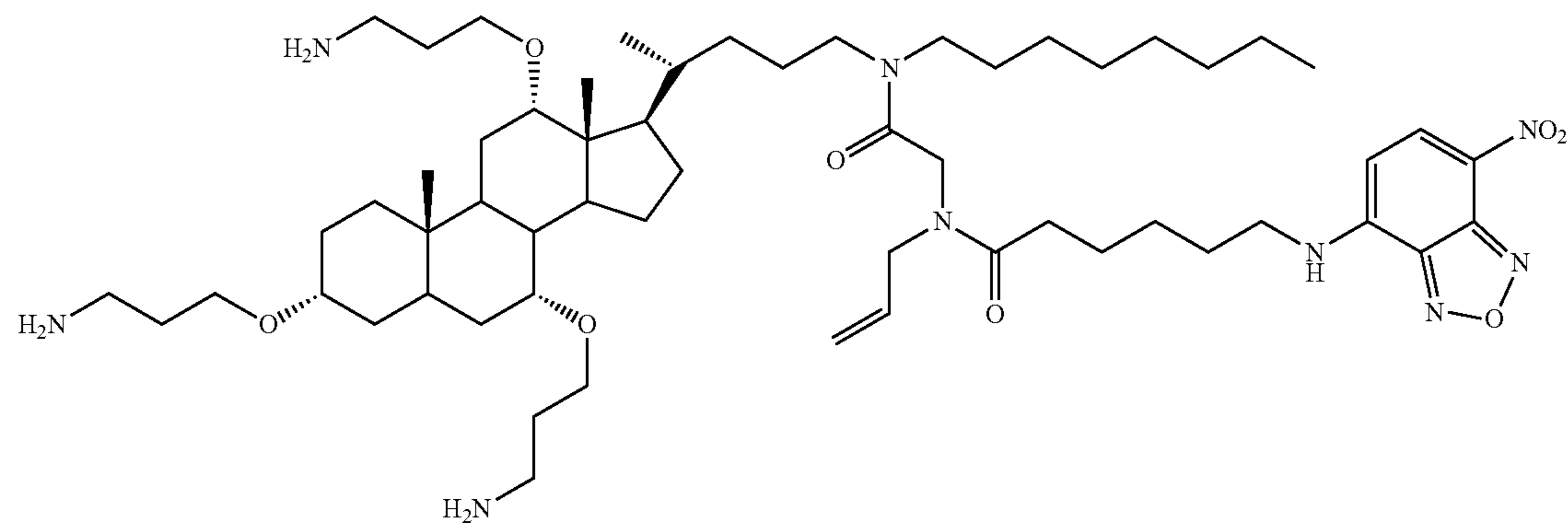
CSA-105
