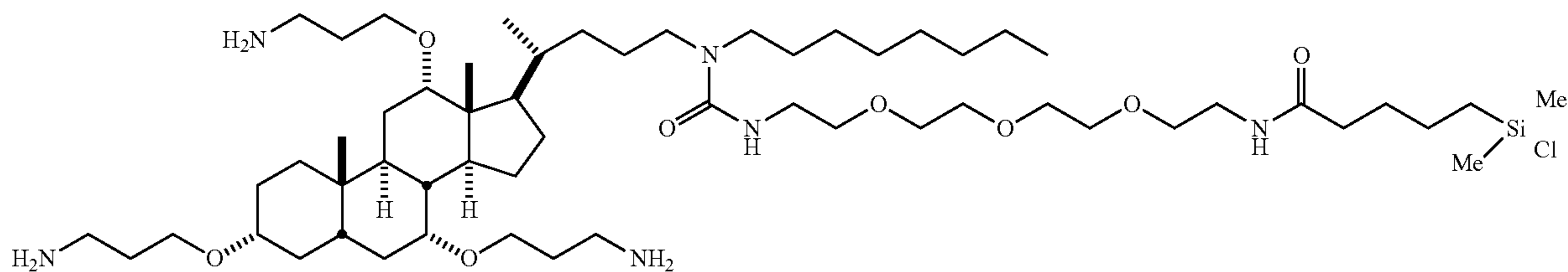
CSA-122
