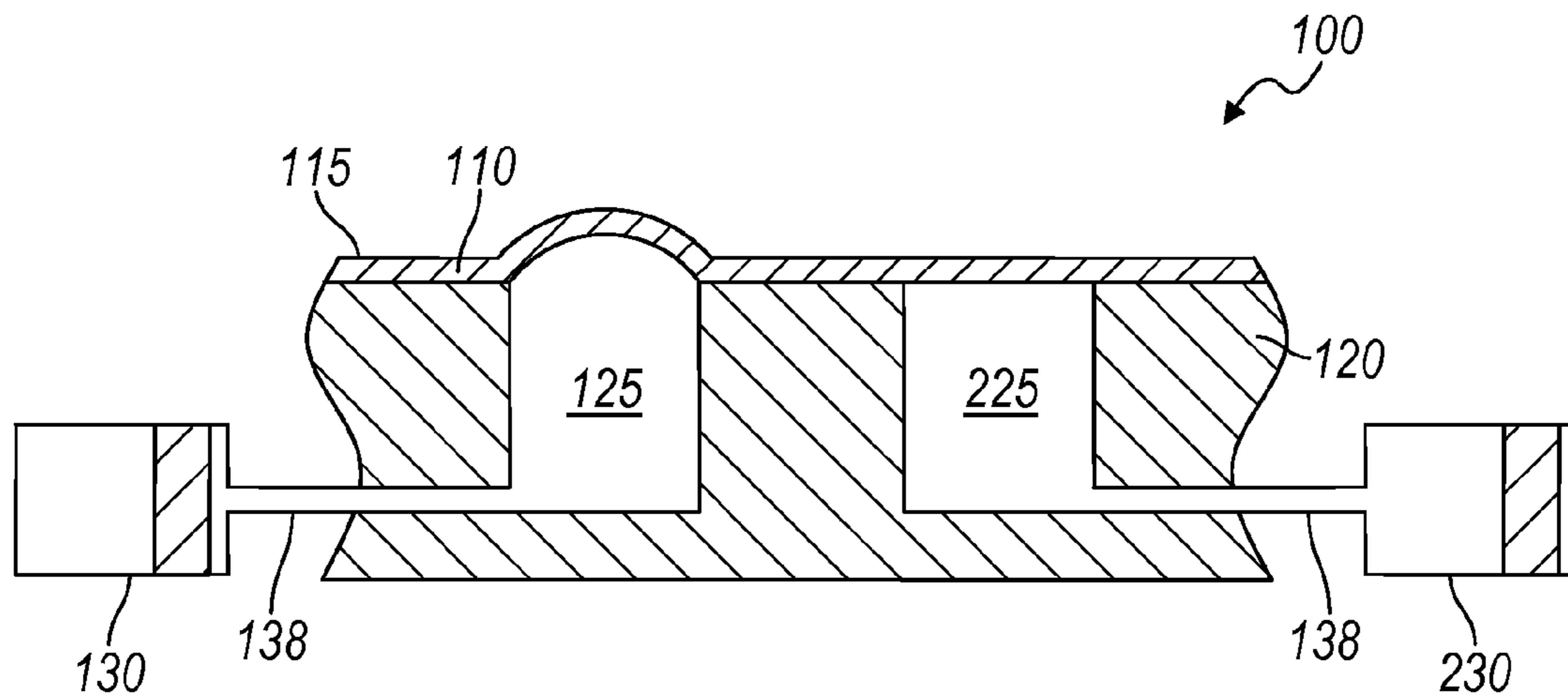
FIG. 19A
