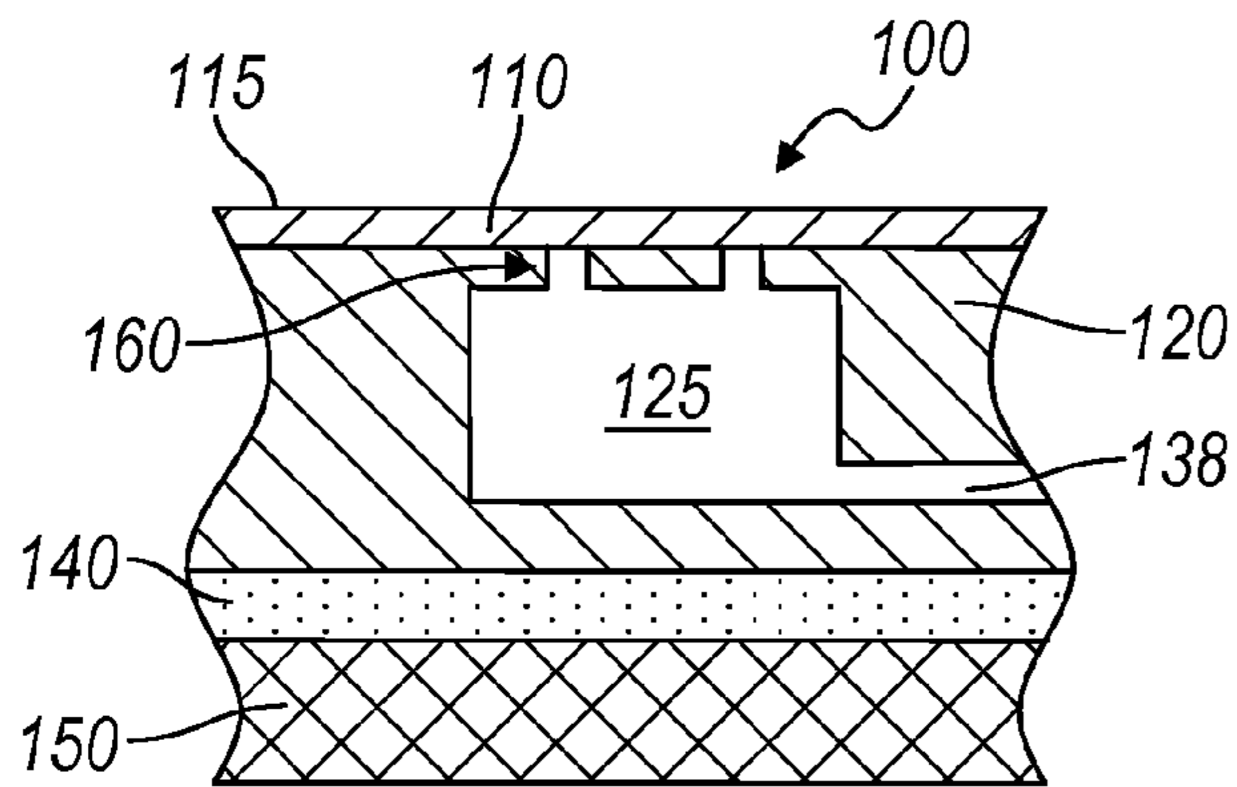
FIG. 6A
