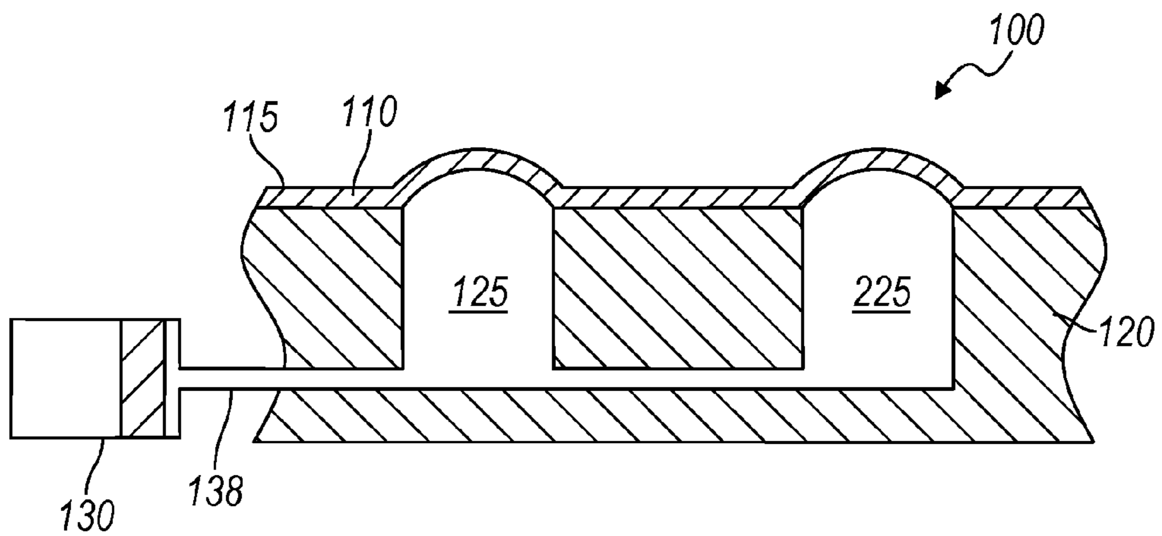
FIG. 18B
