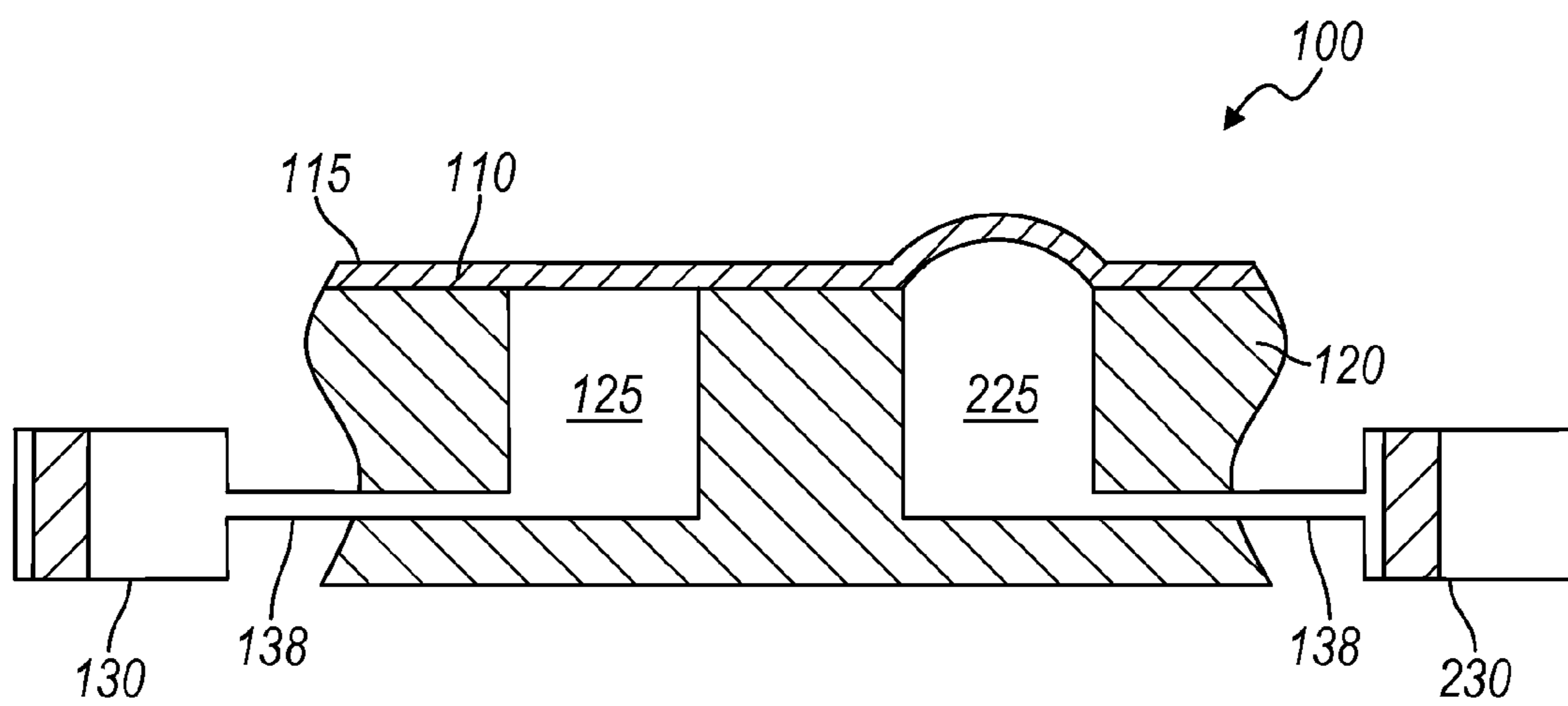
FIG. 19B
