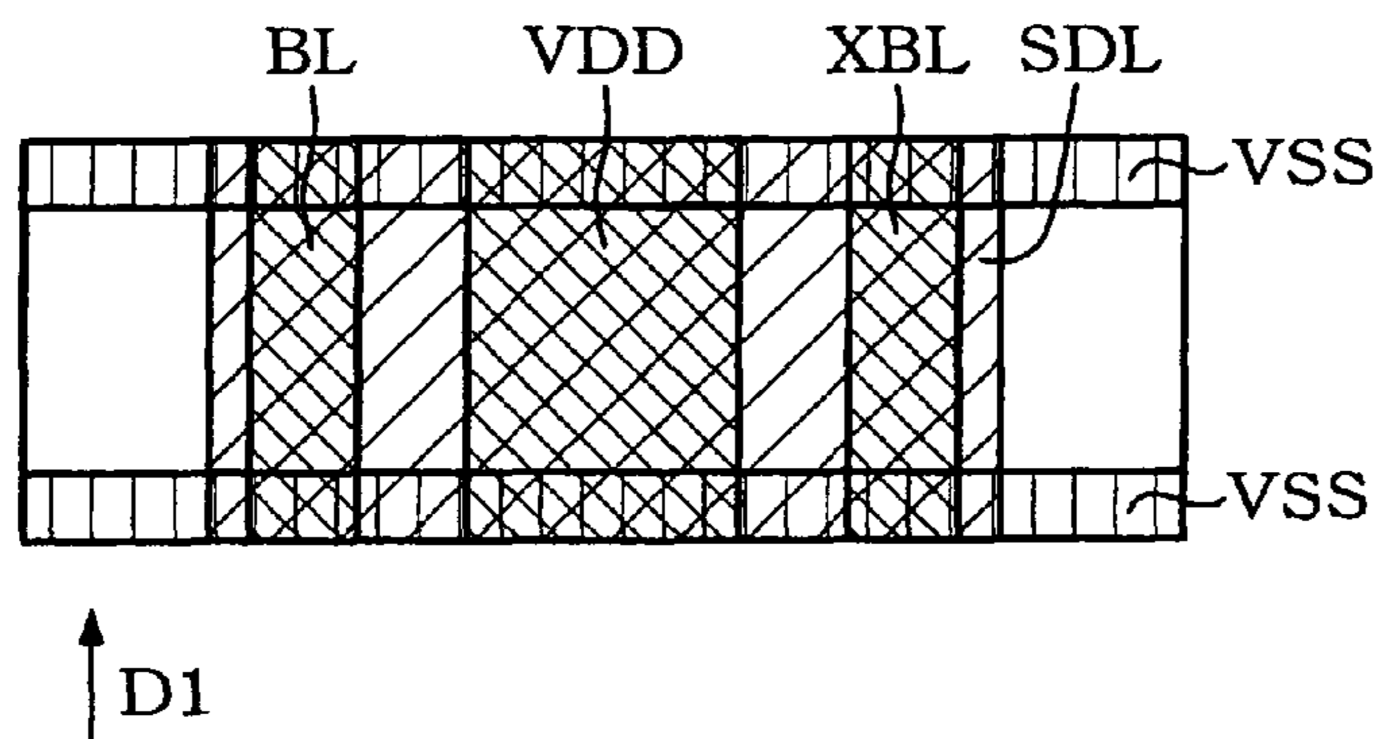
FIG. 20A HORIZONTAL CELL
