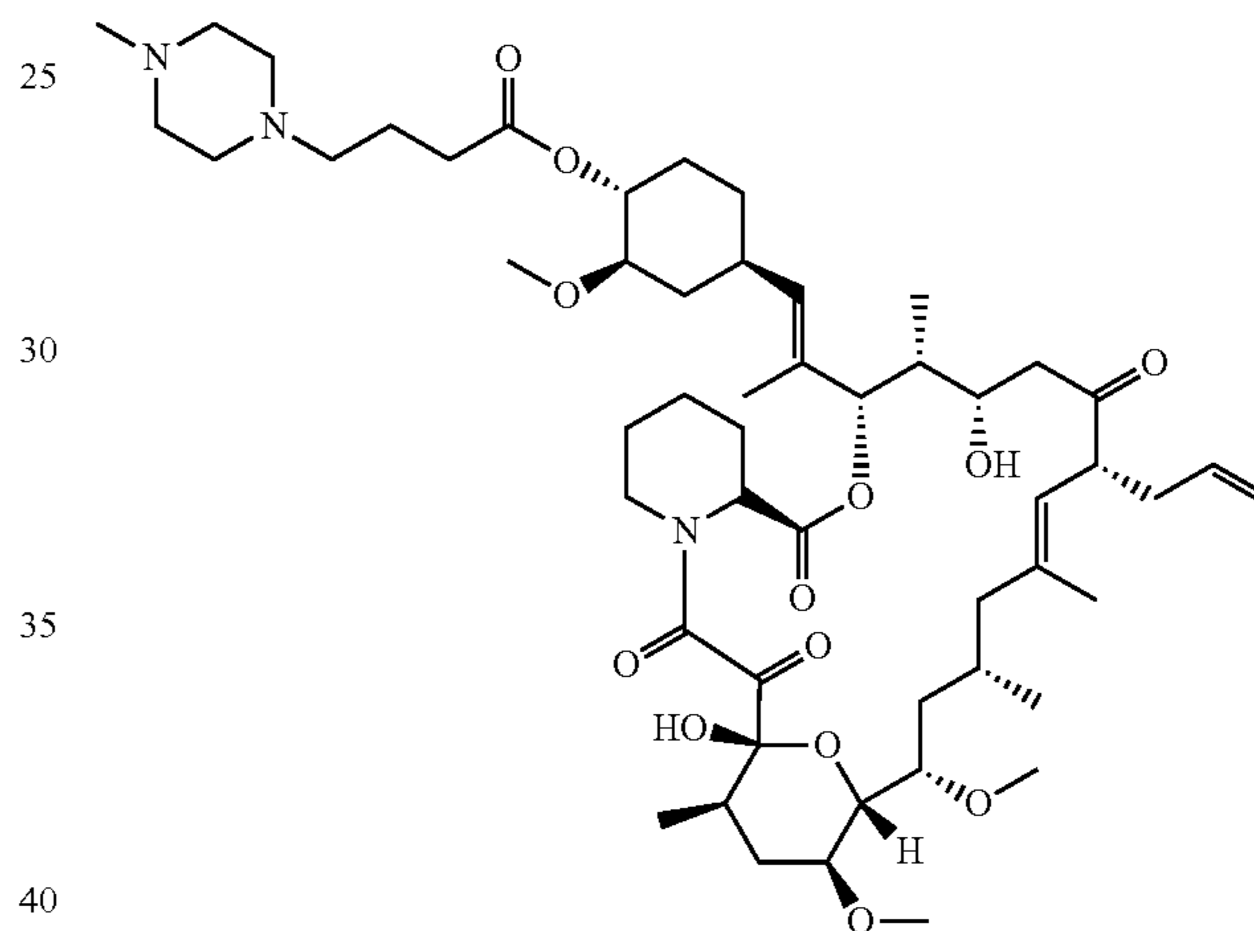
Tacrolimus-liner
