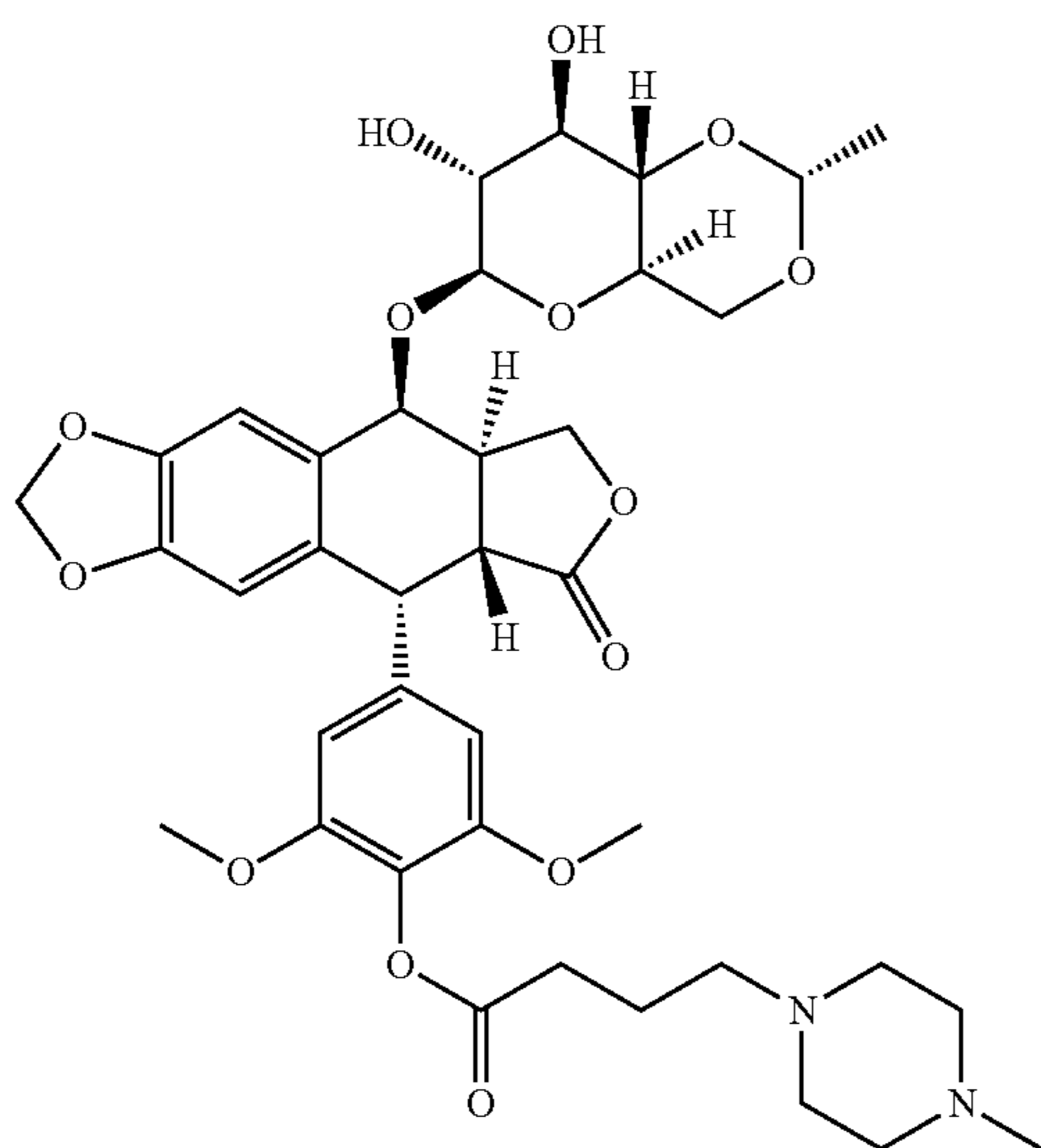
Etoposide-linker 7
