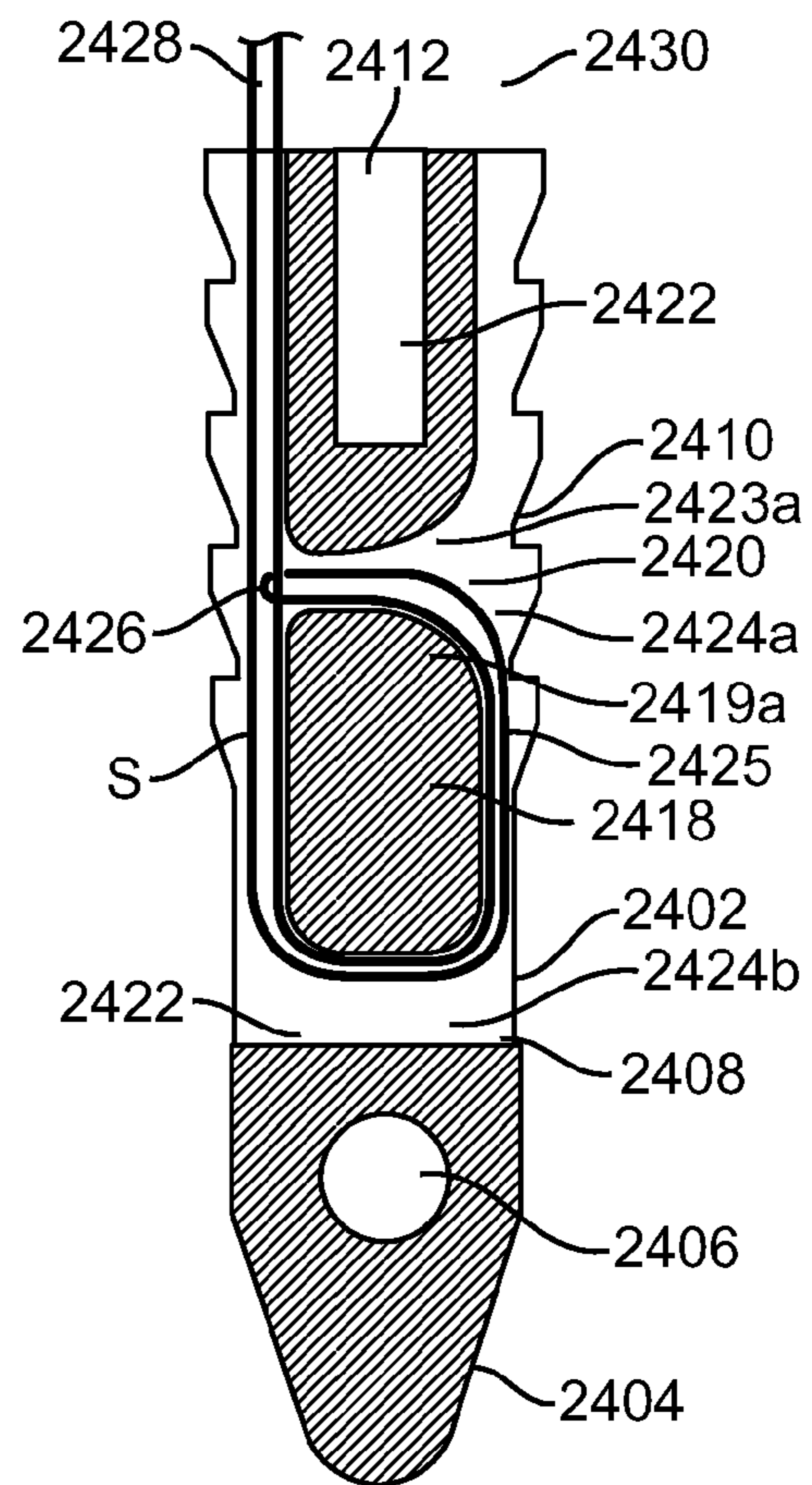
VIEW A-A
