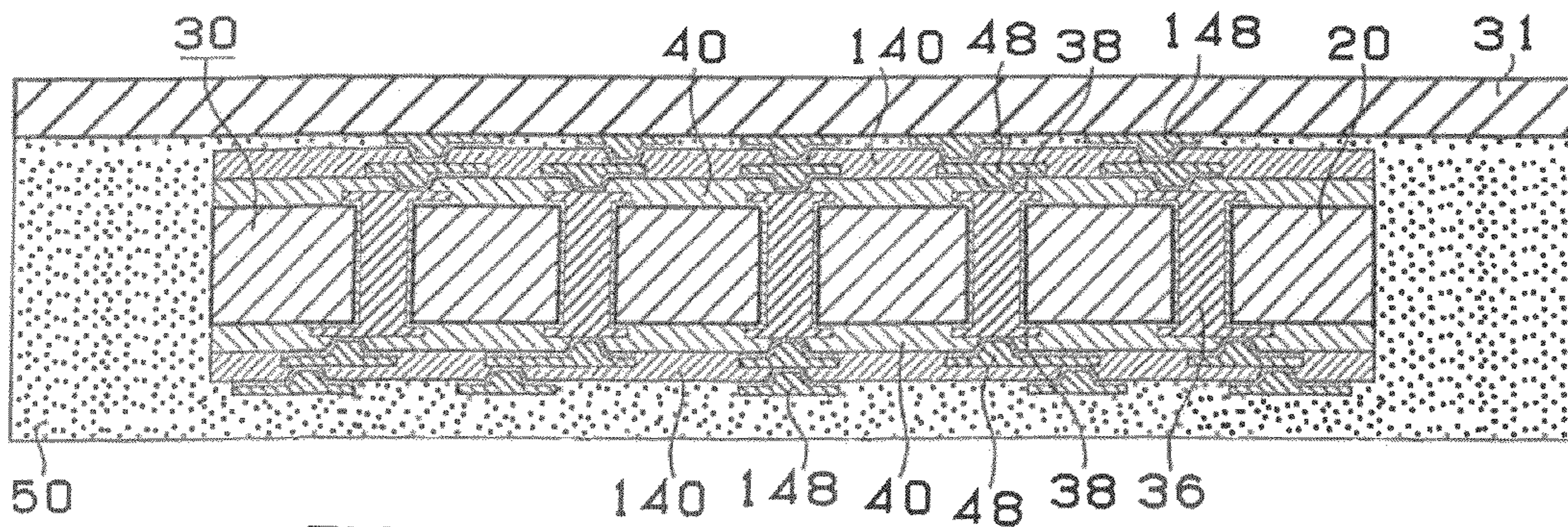
FIG. 5D
