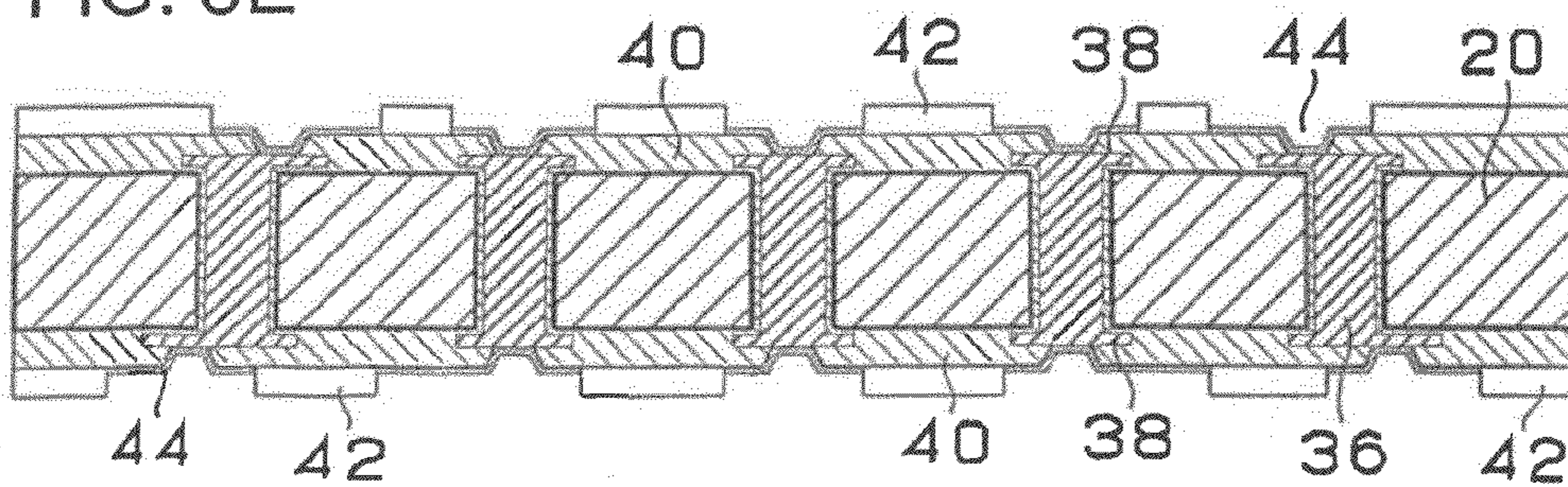
FIG. 3E
