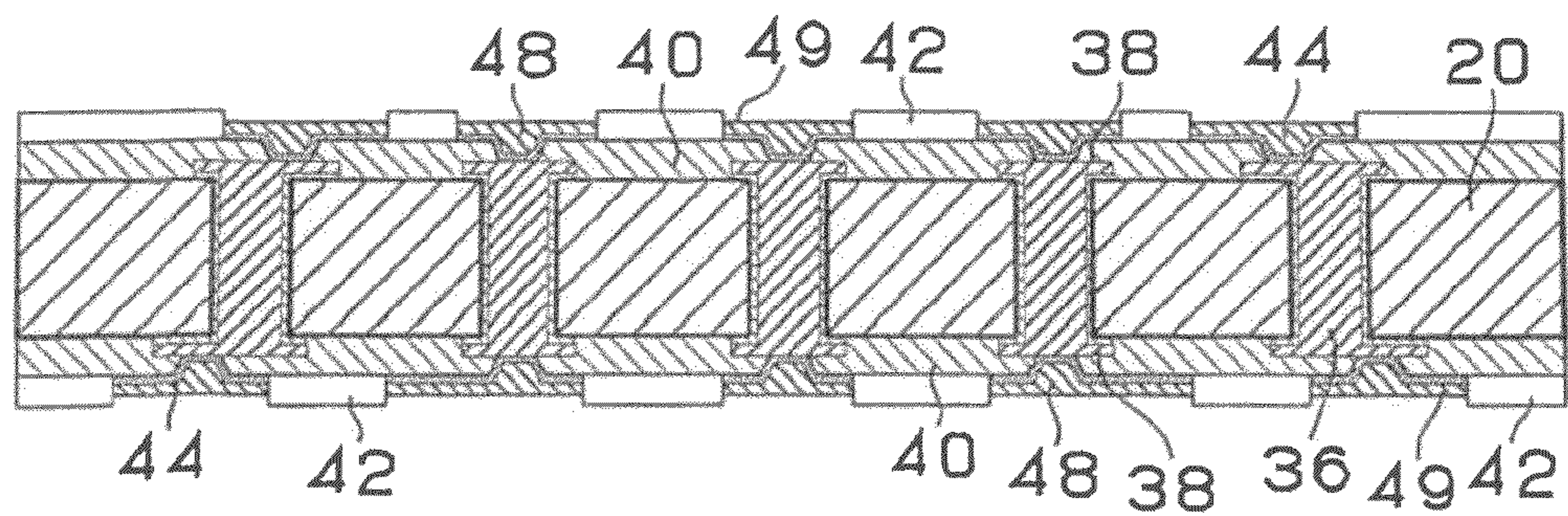
FIG. 4A
