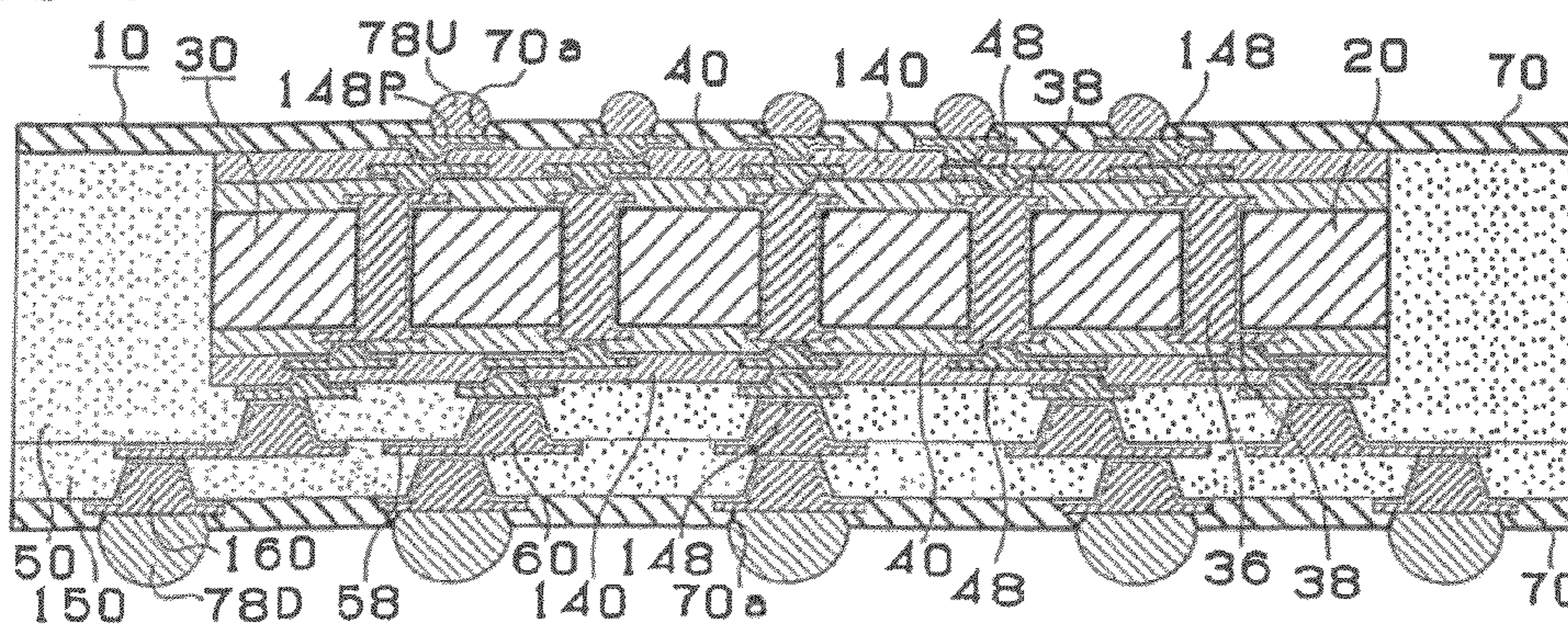
FIG. 7D
