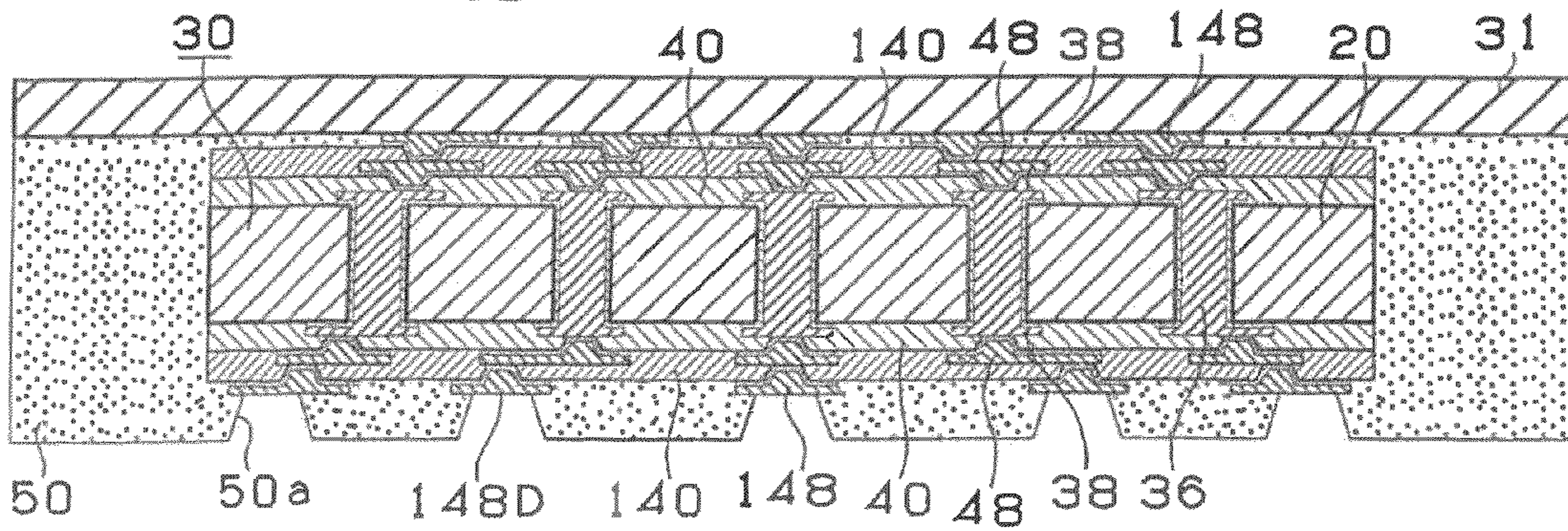
FIG. 5D
