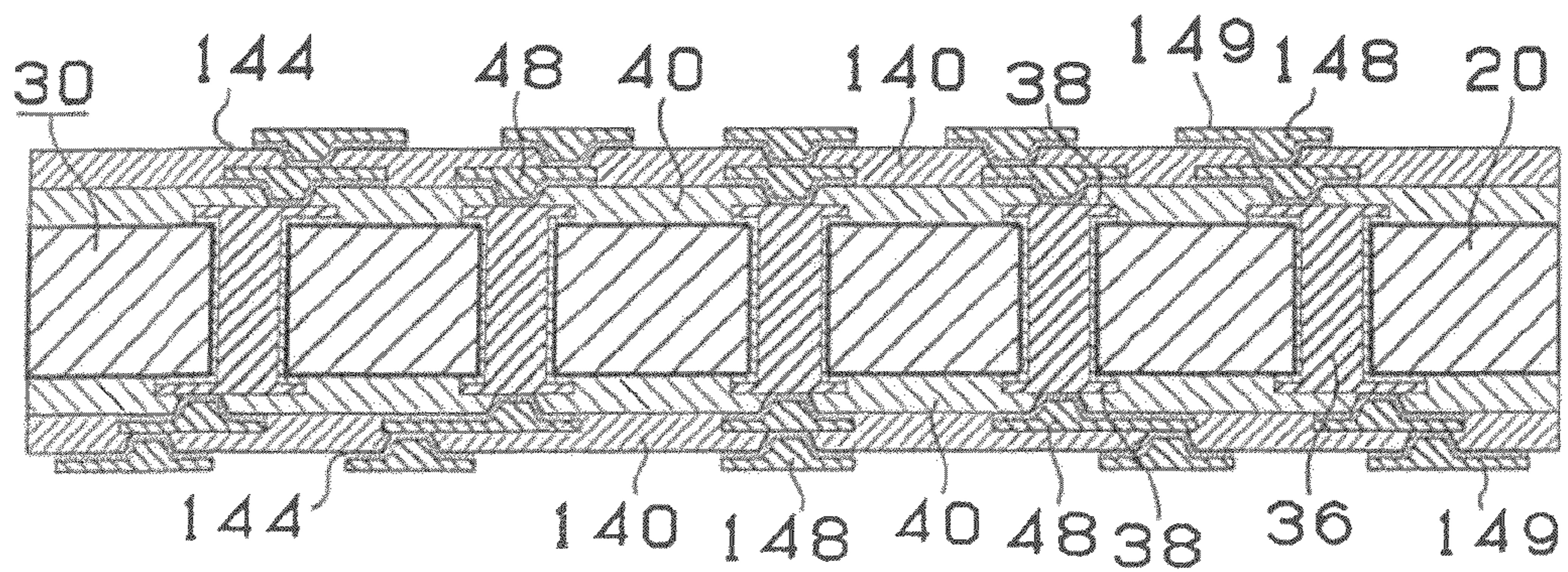
FIG. 4D
