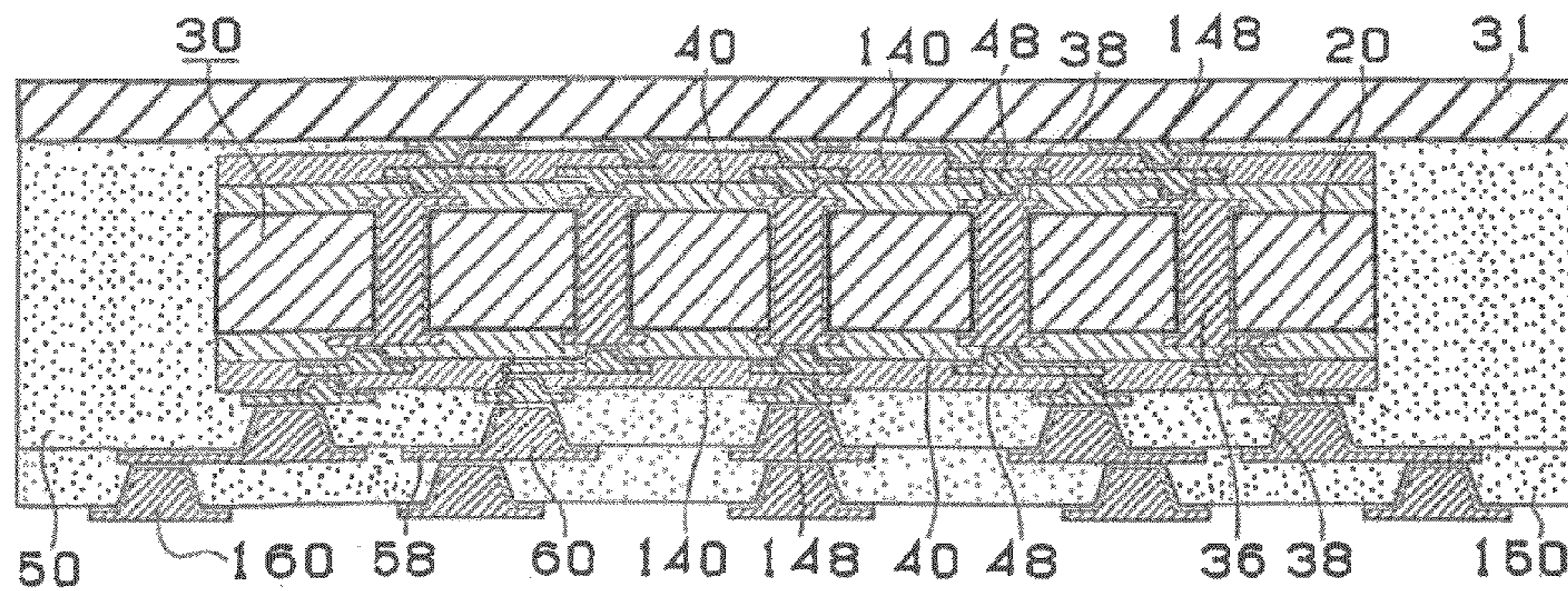
FIG. 7B
