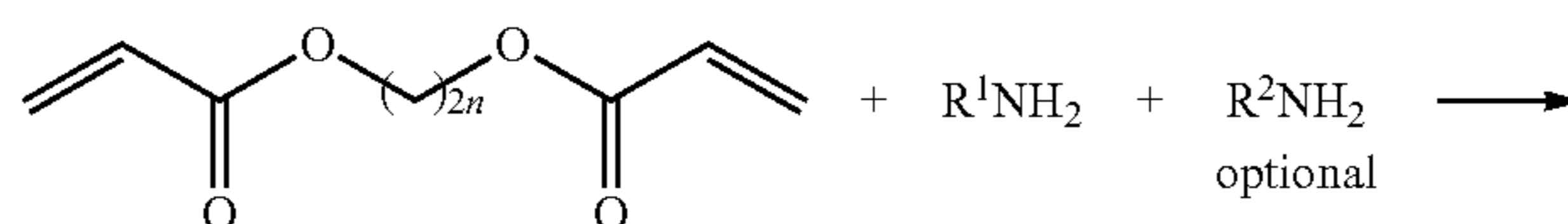
A. Scheme I.
