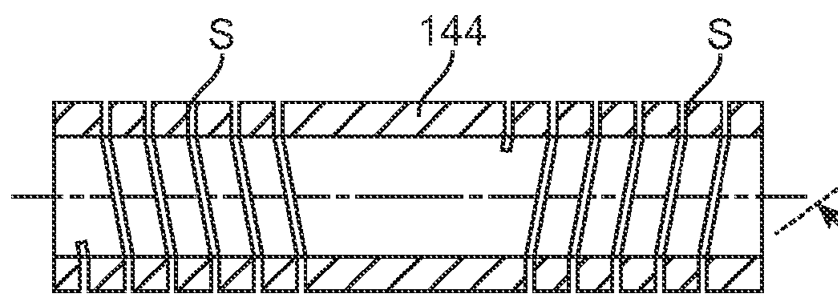
section A-A
