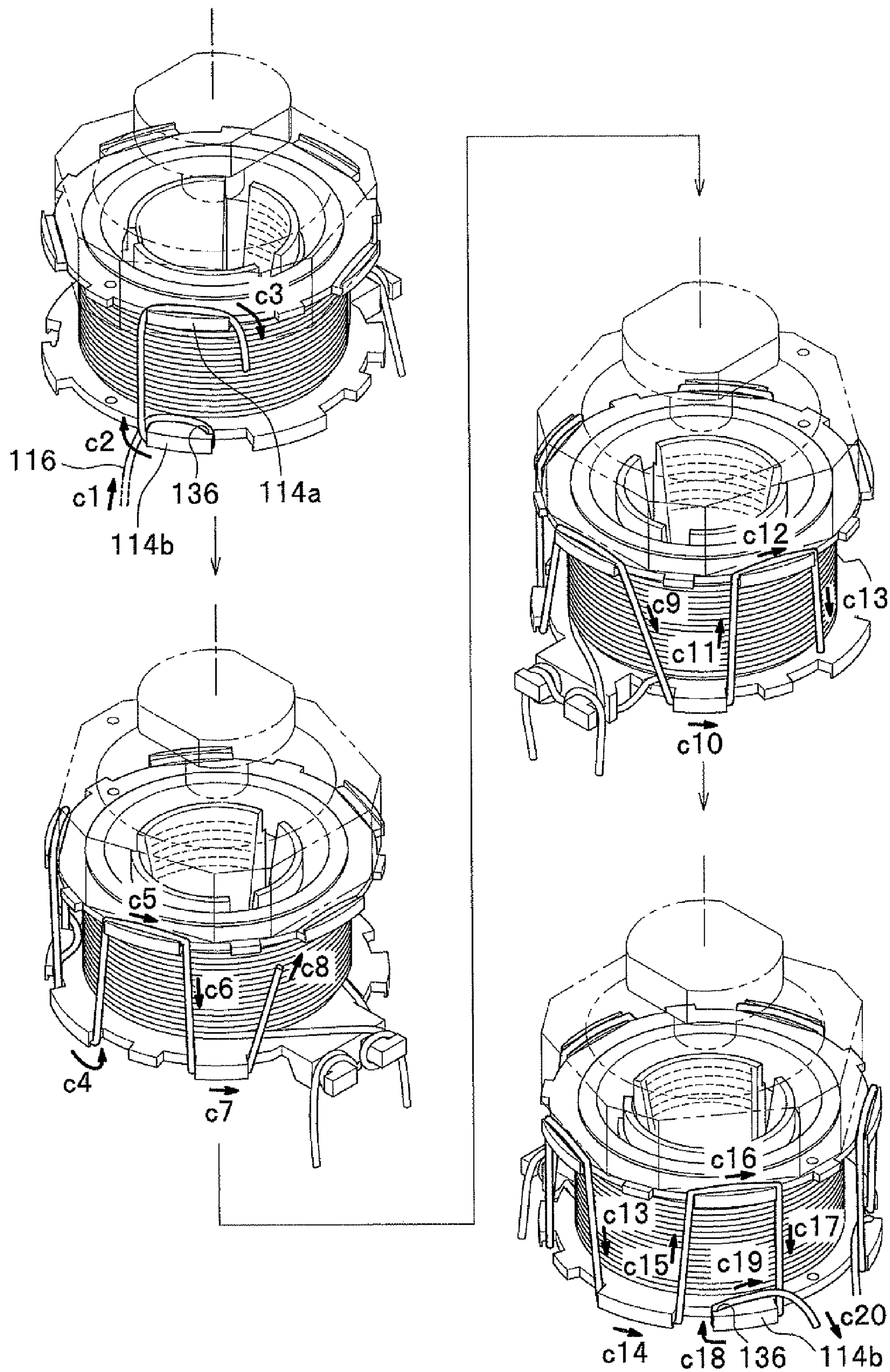
FIG.22
