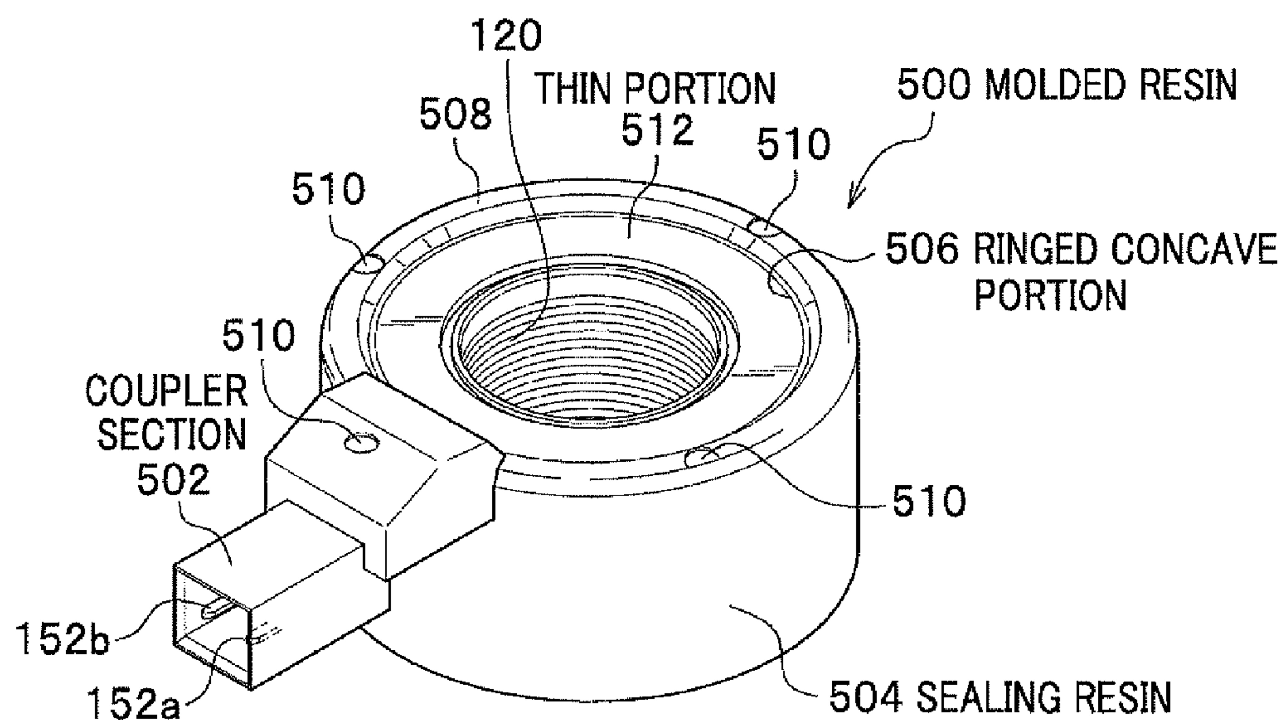
FIG. 29B
