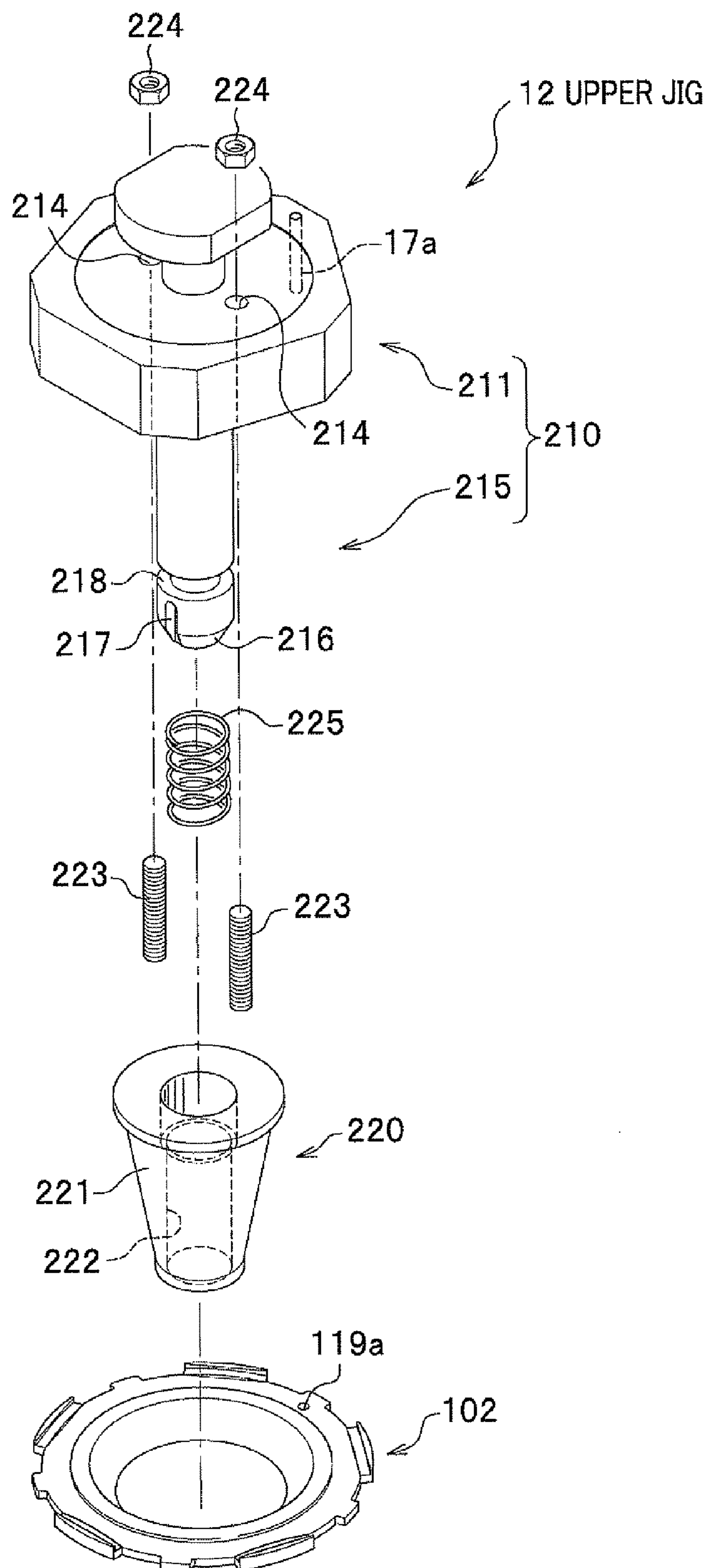
FIG. 10
