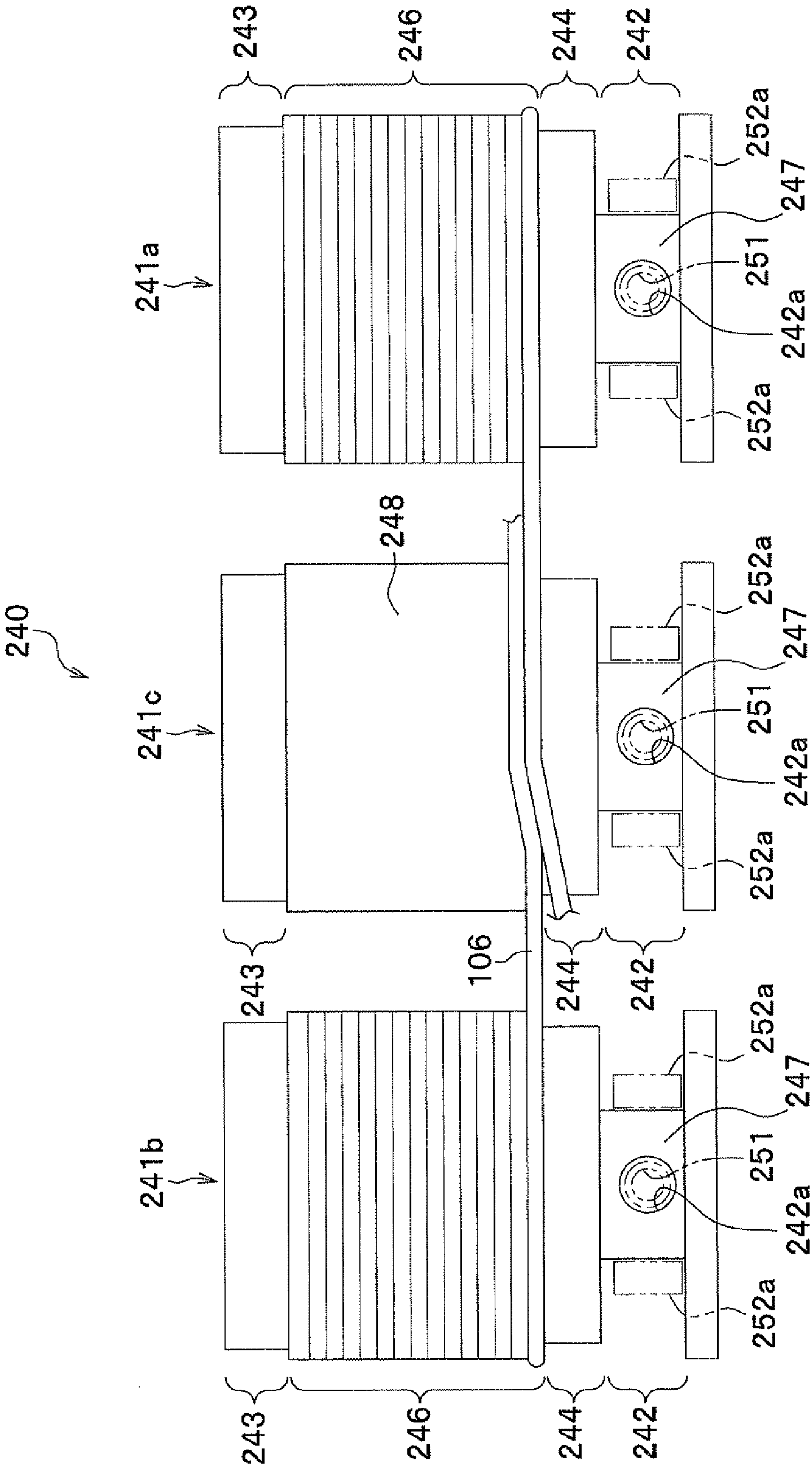
FIG.18
