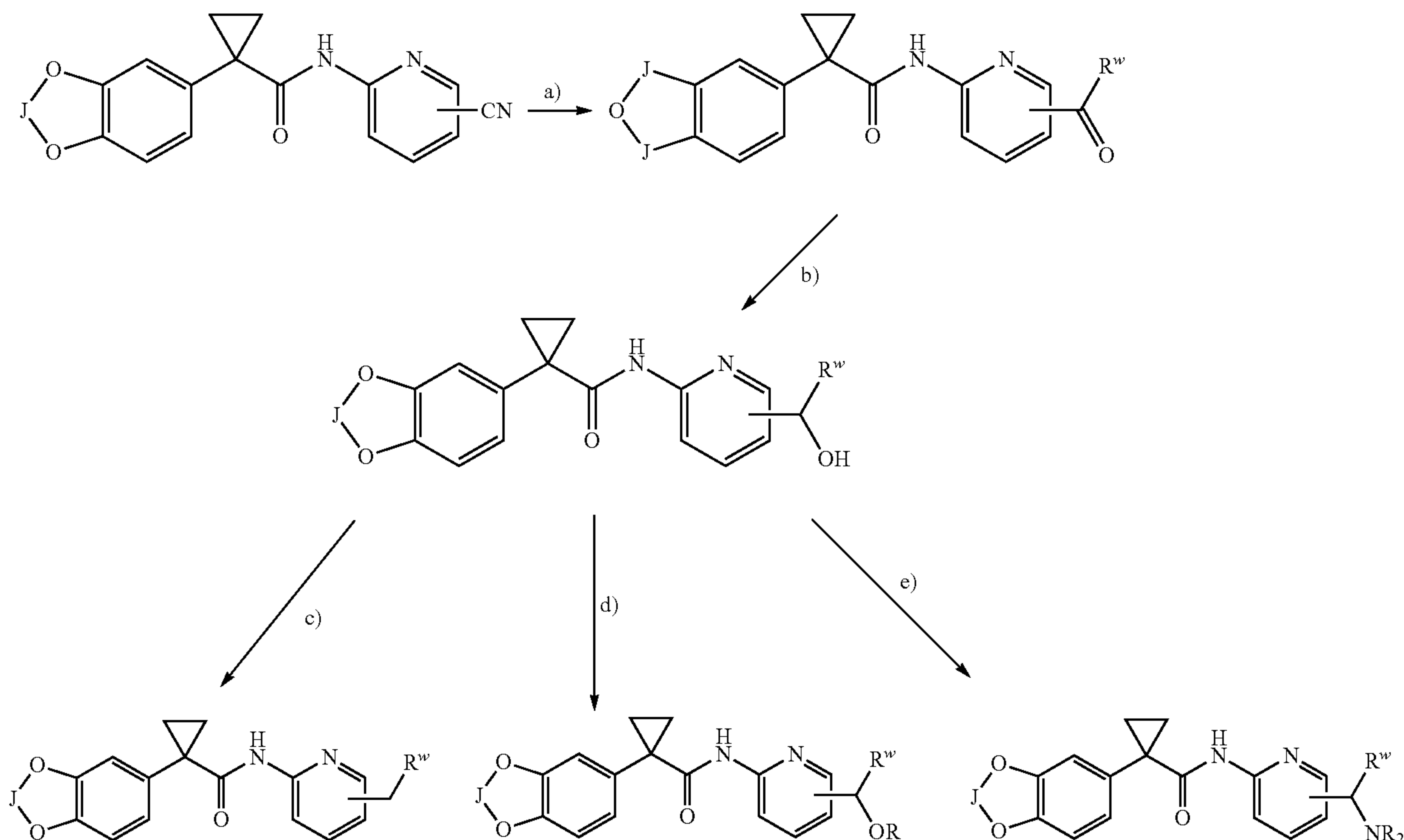
Scheme IVb
