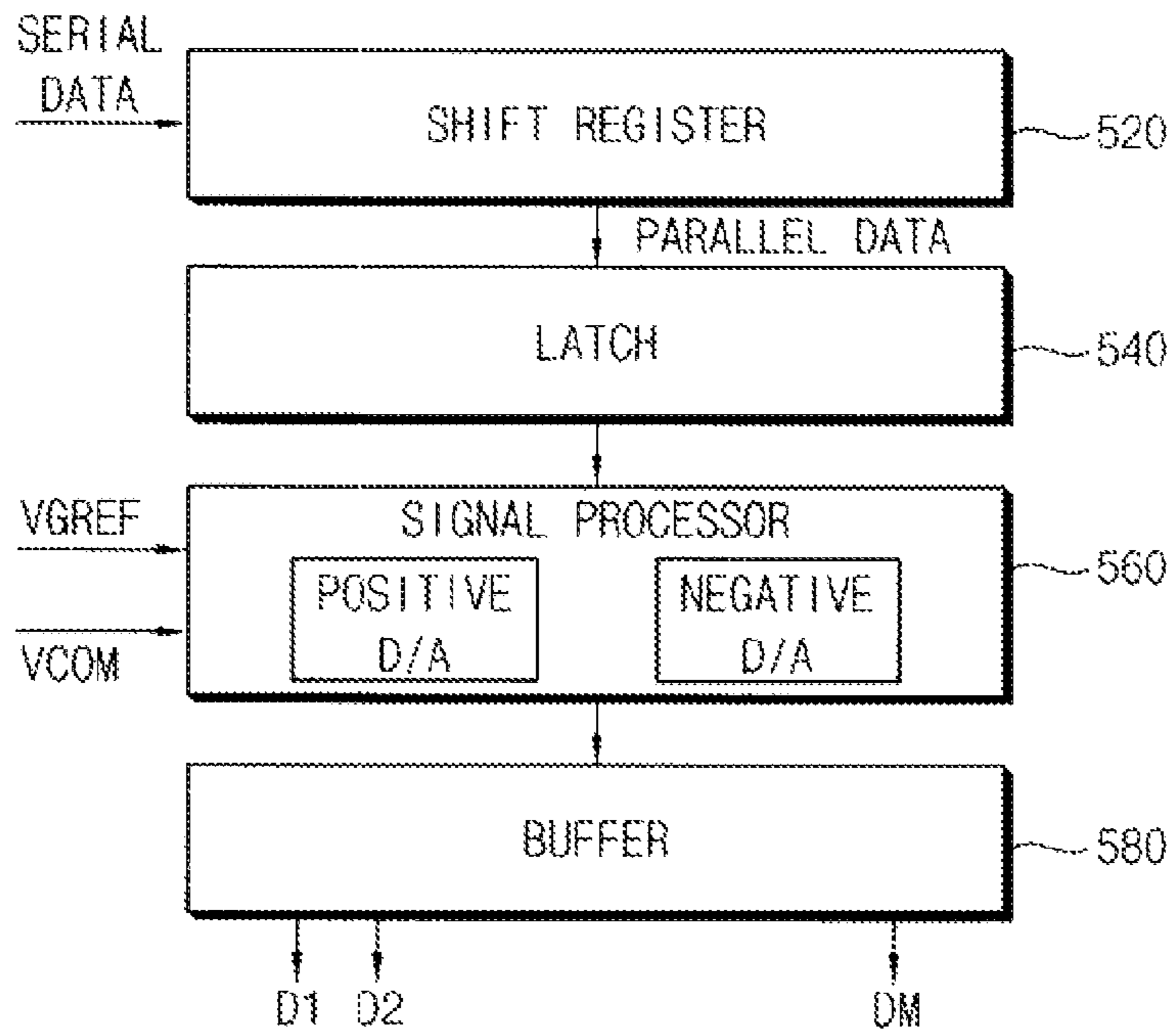
FIG. 4 500
