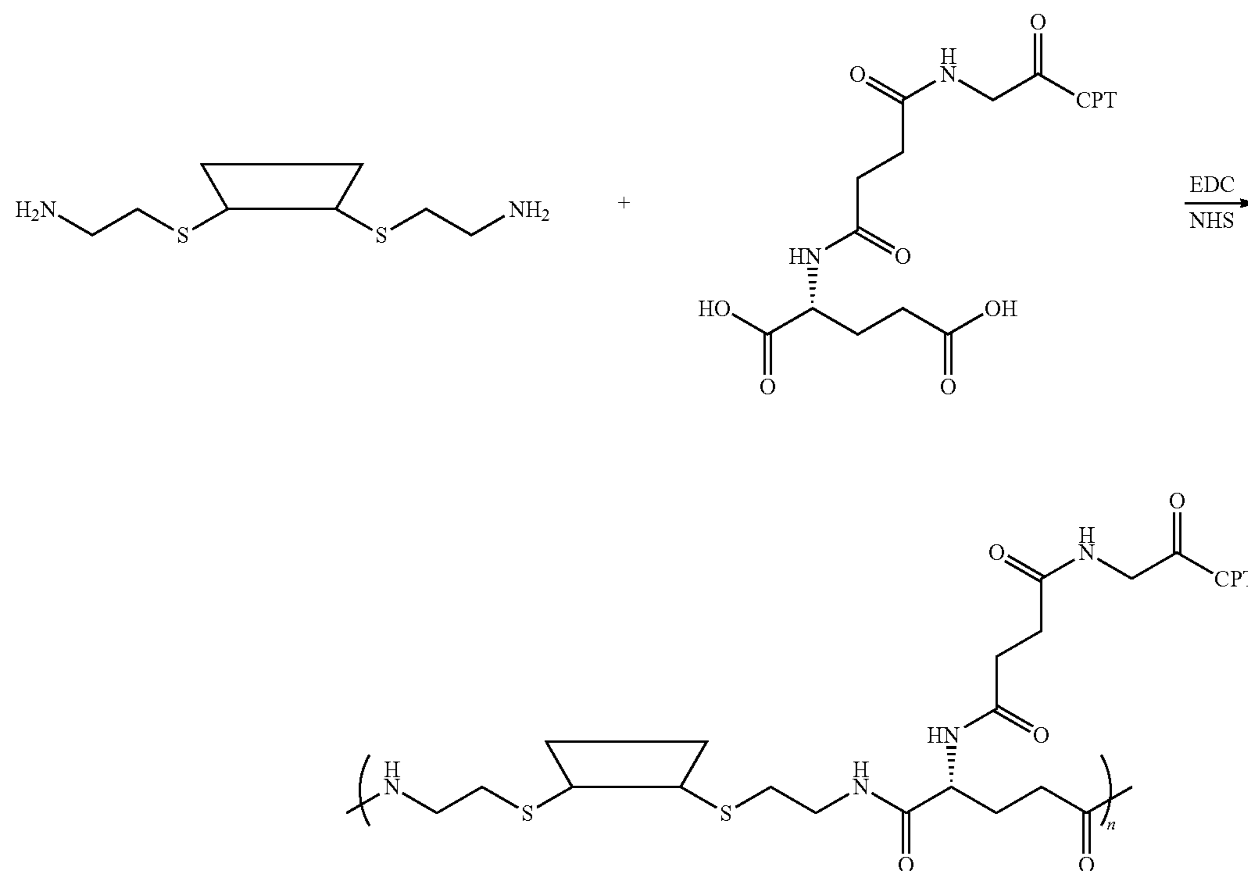
Scheme VI
