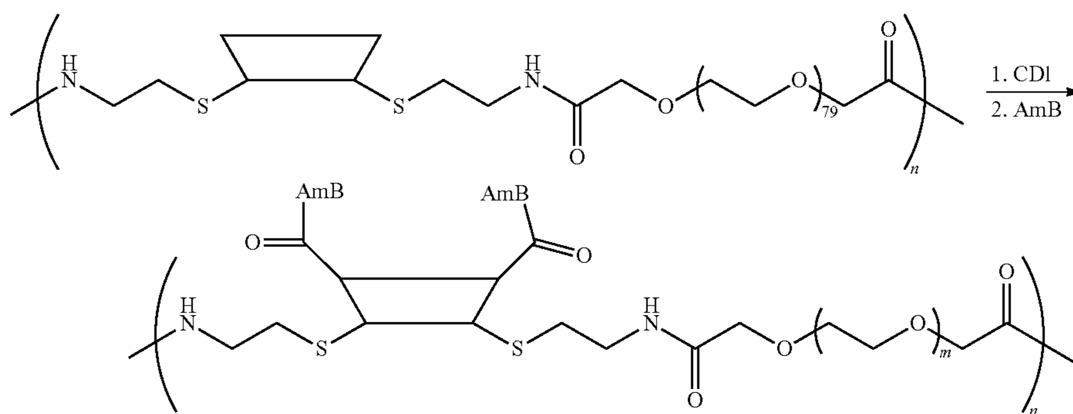
Scheme LII
