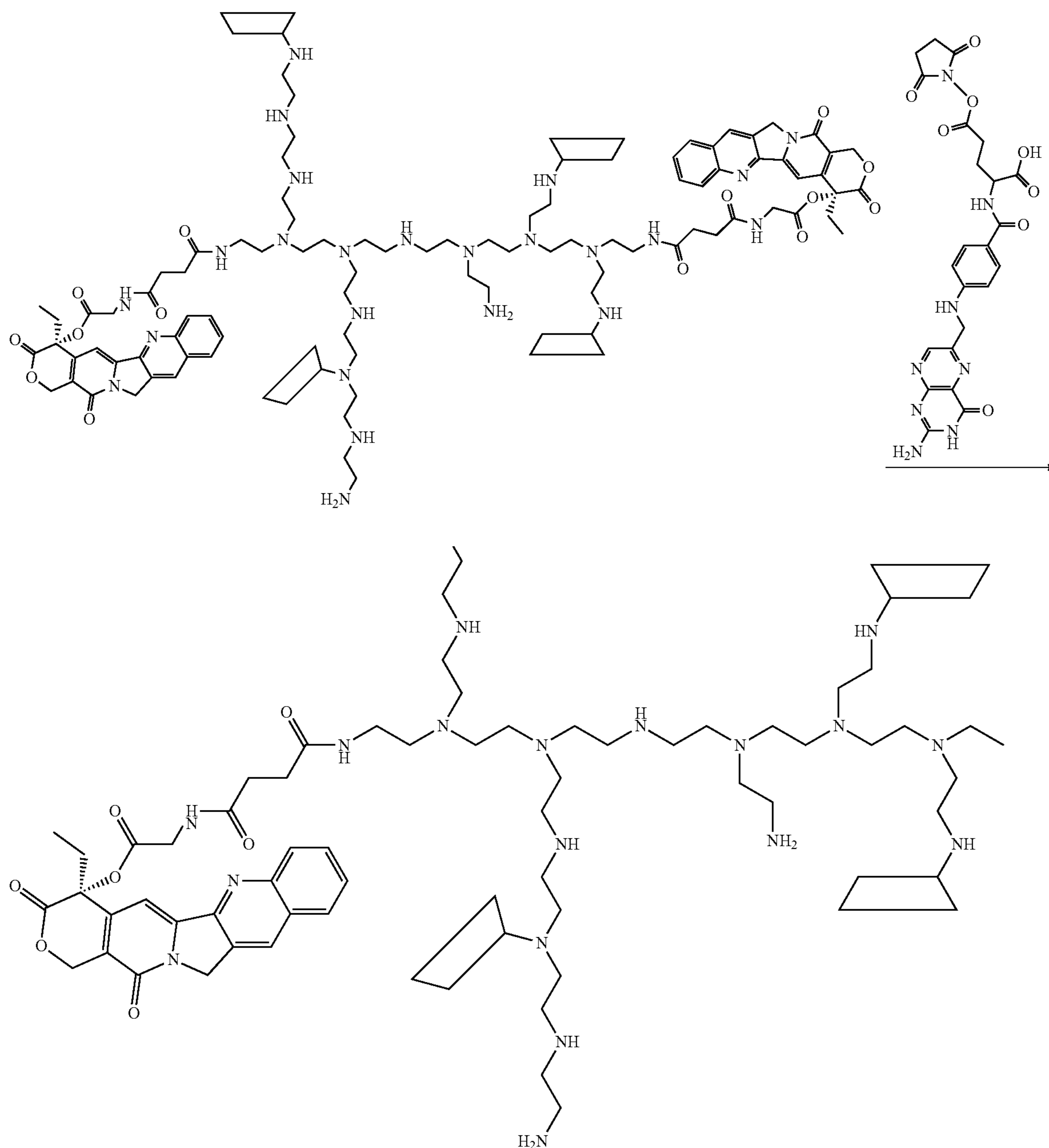
Scheme LI
