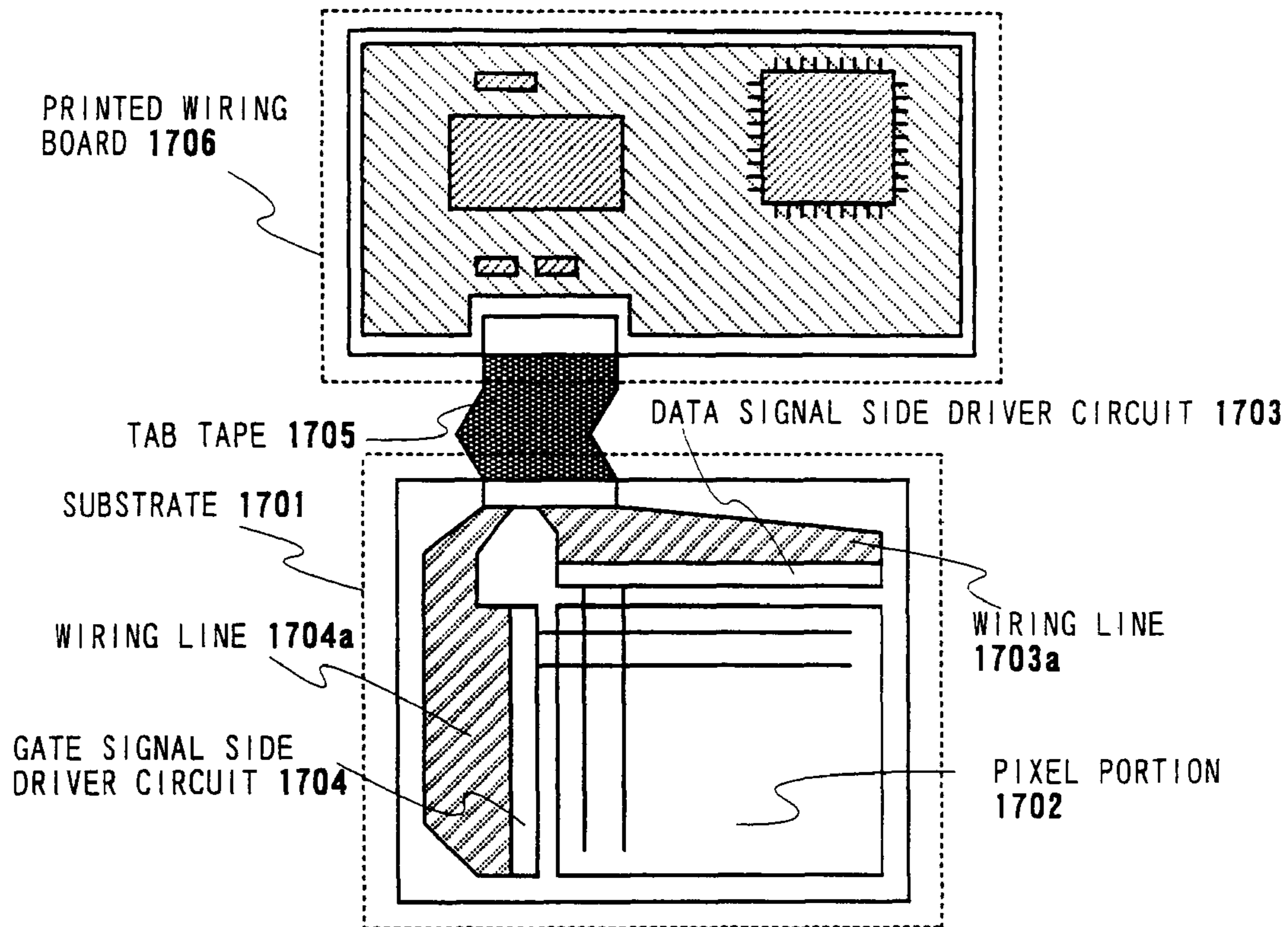
FIG. 17A
