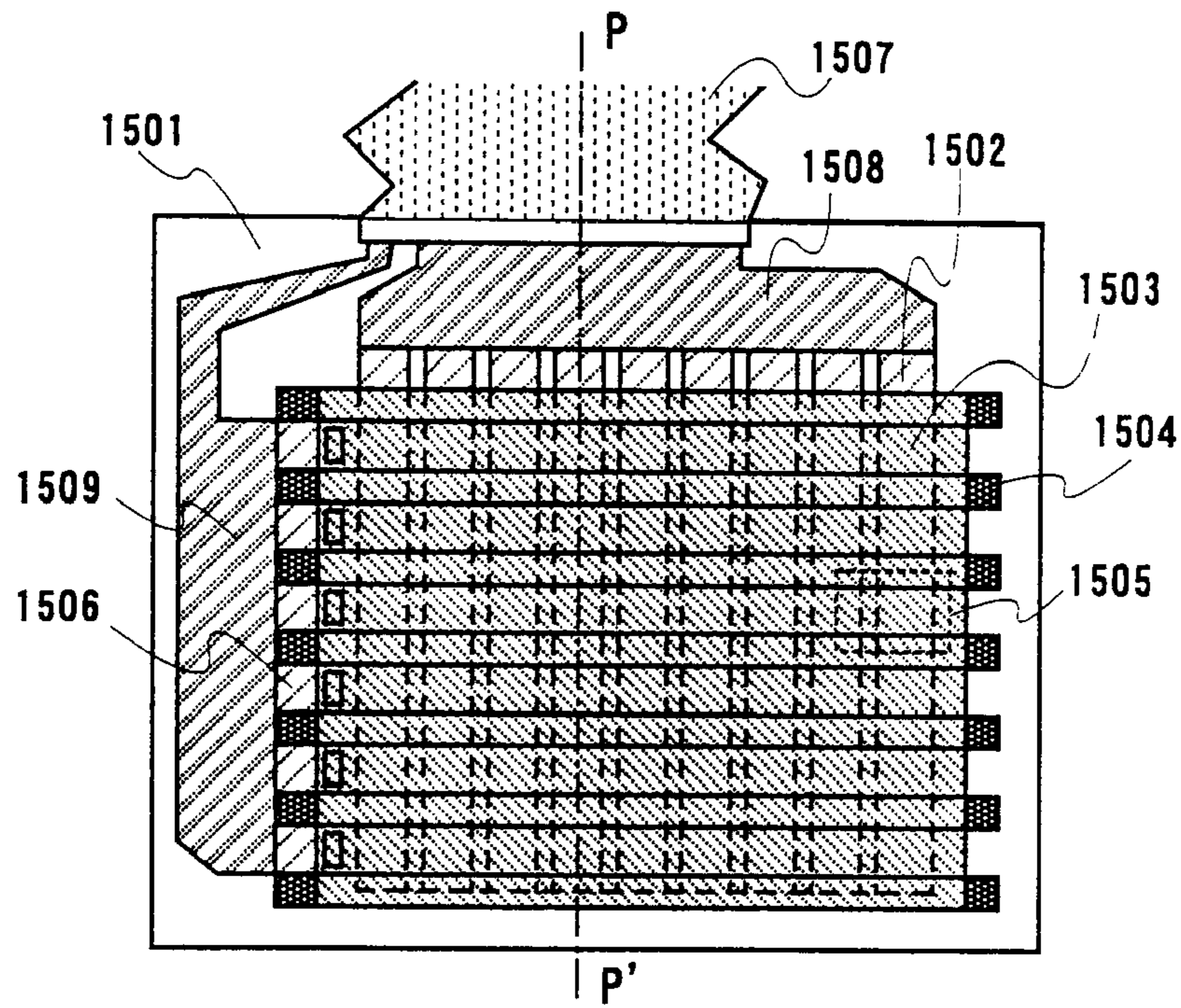
FIG. 15A
