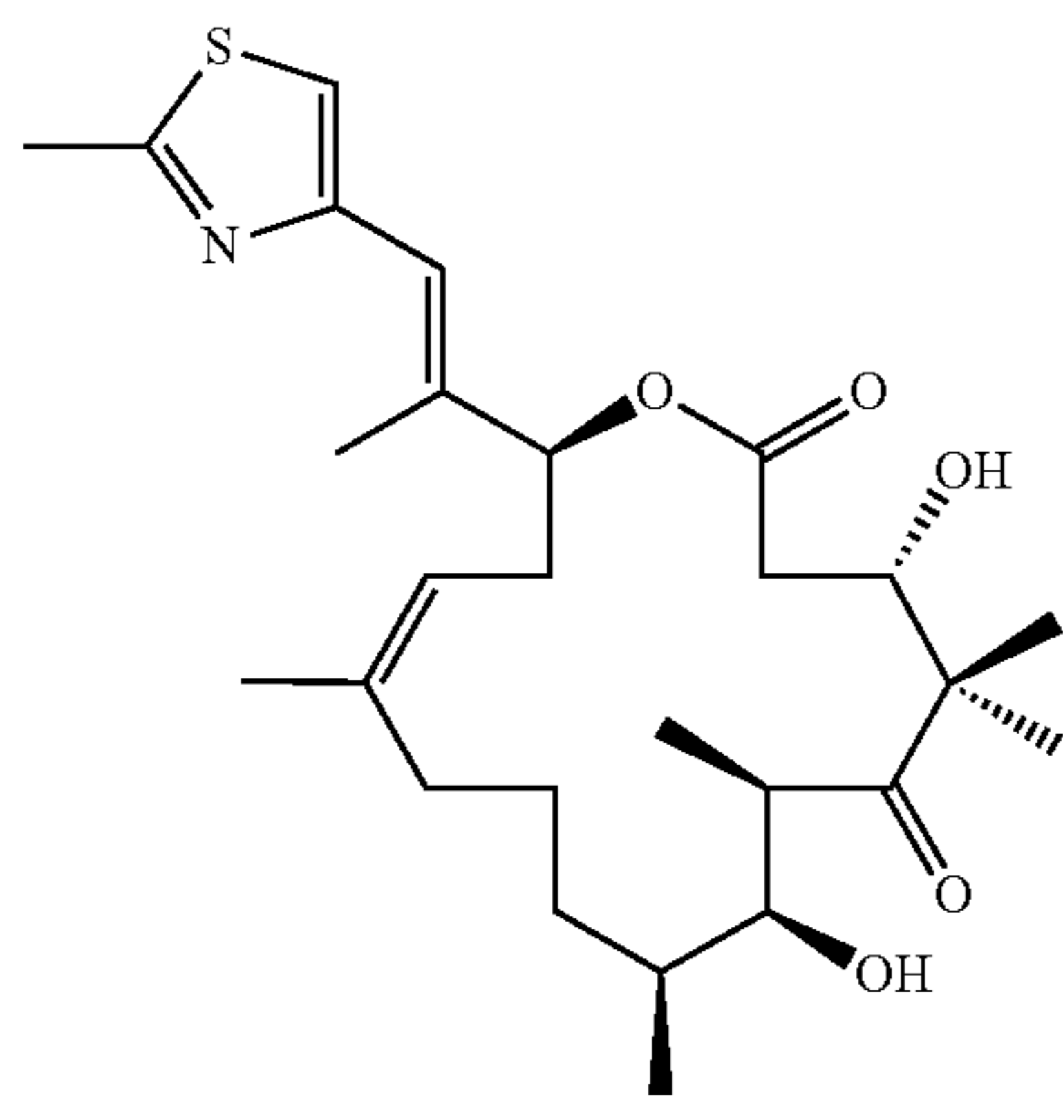
dEpoB (1)
