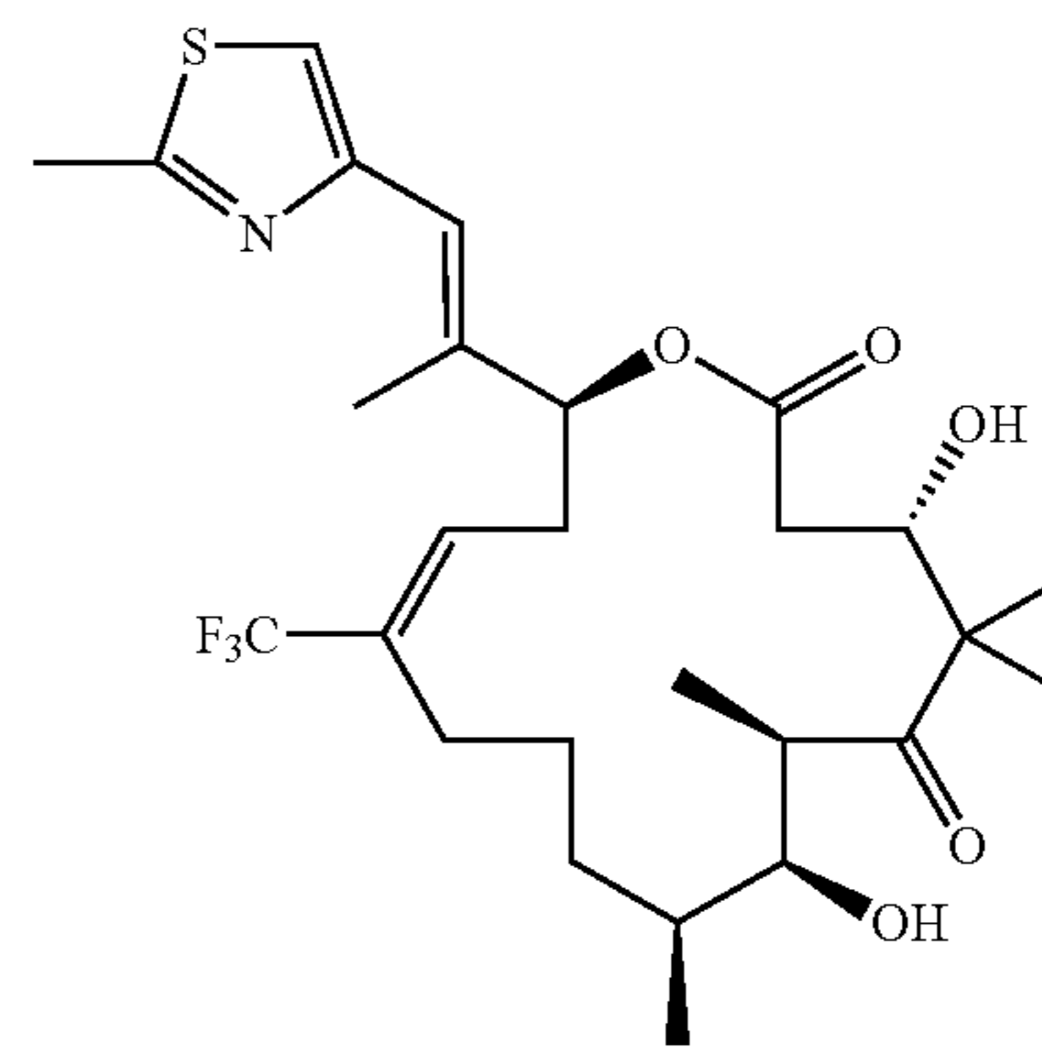
26-F 3 -[16]dEpoB
