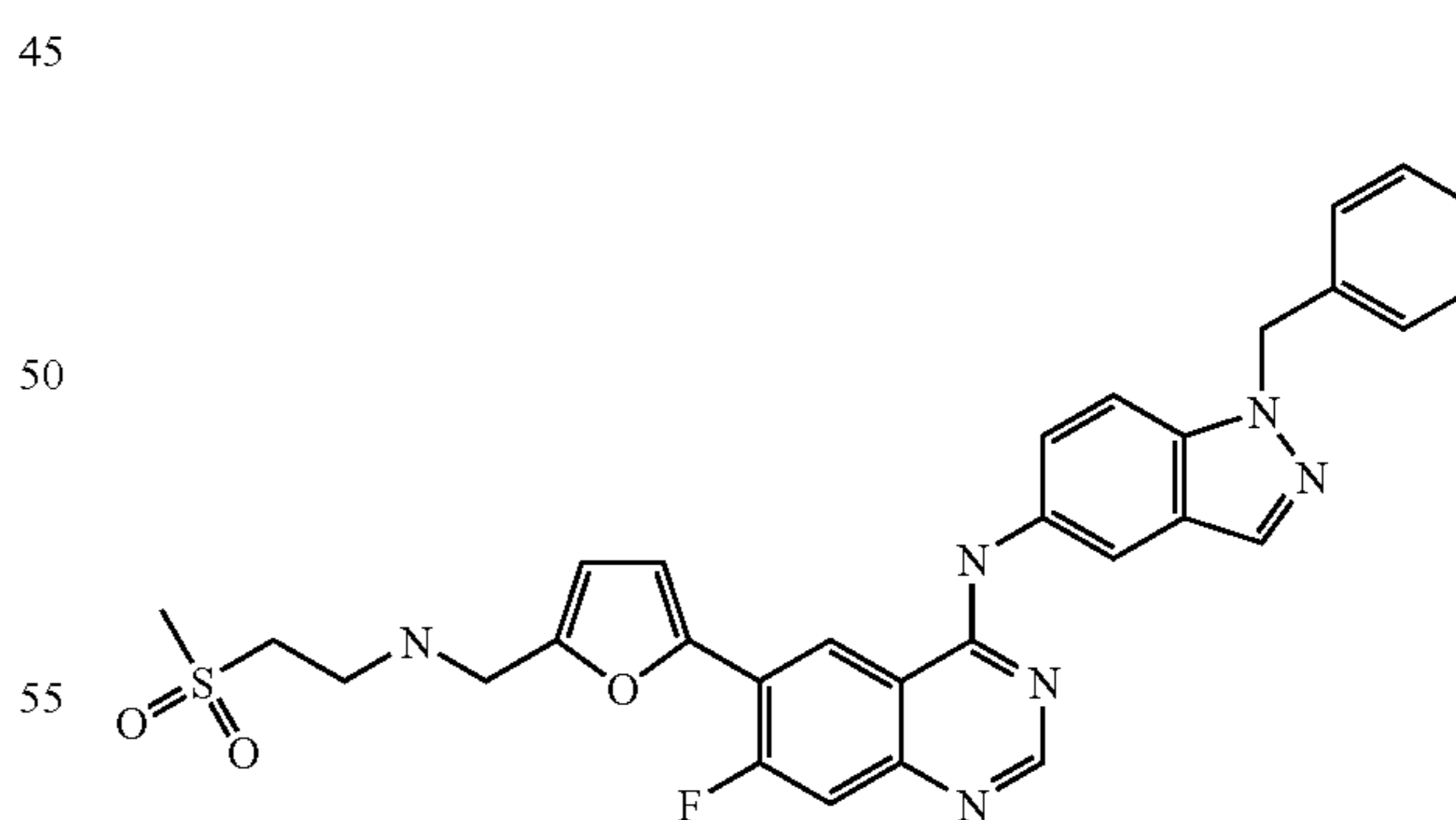
N-(1-Benzyl-1H-indazol-5-yl)-7-fluoro-6-[5-({[2-(methanesulphonyl)ethyl]amino}methyl)-2-furyl]-4-quinazolinamine
