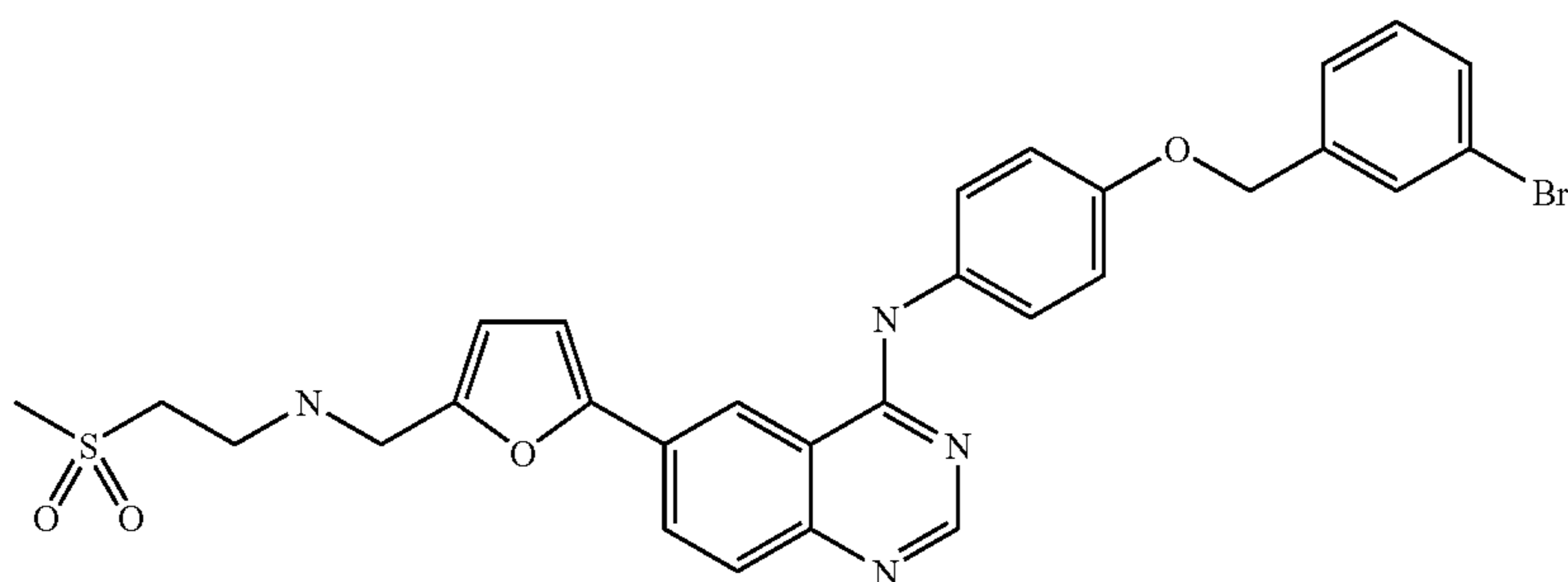
N-{4-[(3-bromobenzyl)oxy]phenyl}-6-[5-({[2-(methanesulphonyl)ethyl]amino}methyl)-2-furyl]-4-quinazolinamine
