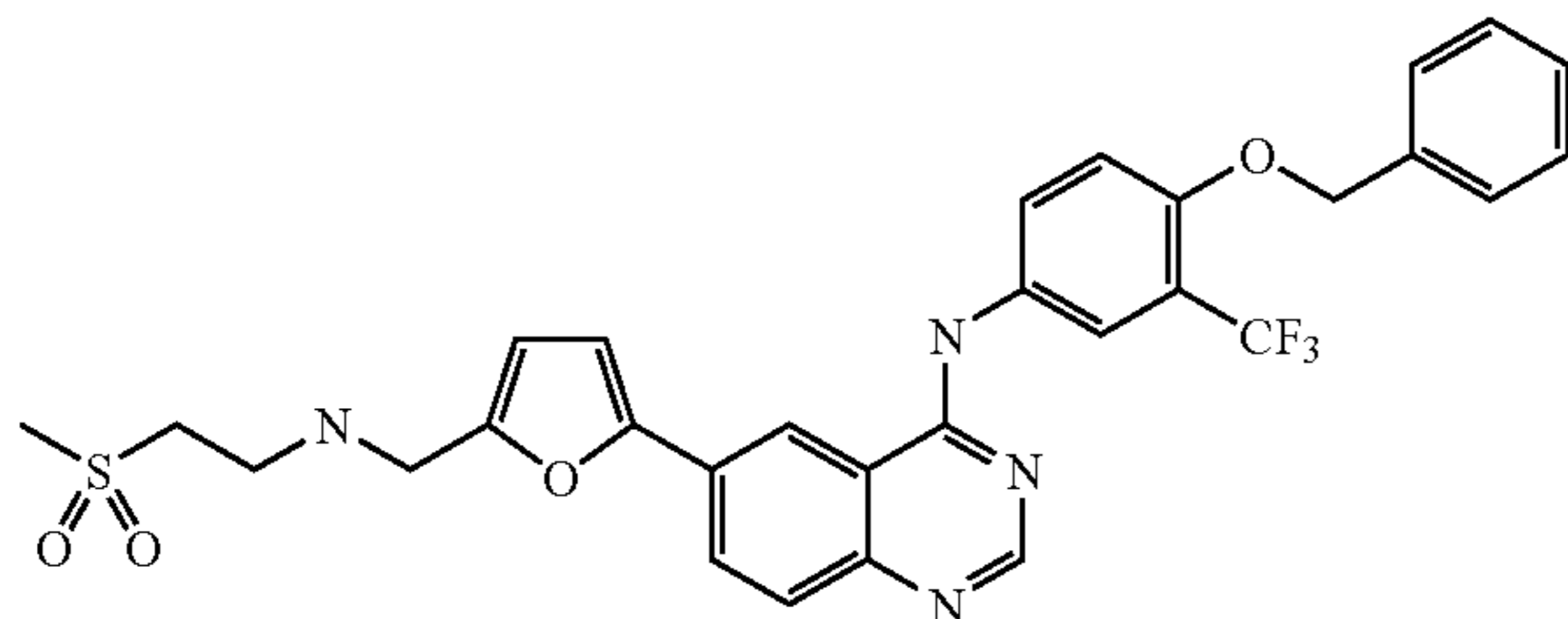
N-(3-Trifluoromethyl-4-benzyloxyphenyl)-6-[5-({[2-(methanesulphonyl)ethyl]amino}methyl)-4-furyl]-4-quinazolinamine
