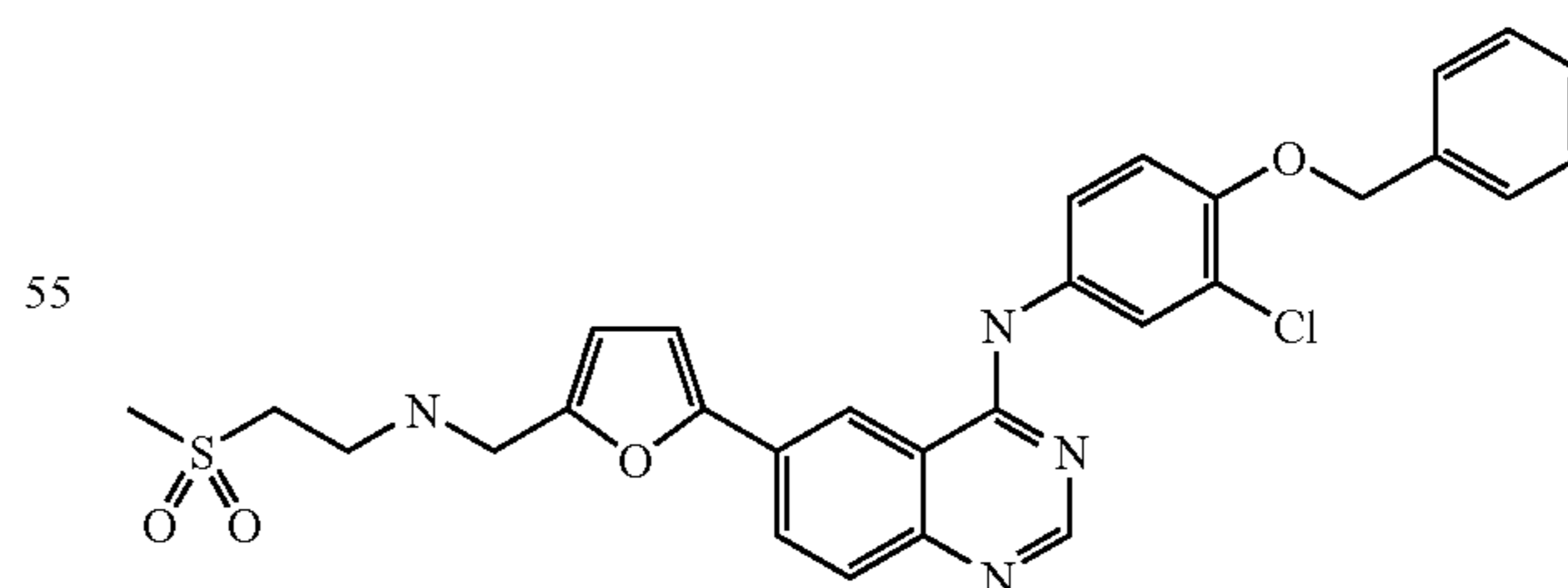
N-(3-Chloro-4-benzyloxyphenyl)-6-[5-({2-(methanesulphonyl)ethyl}amino)methyl]-4-furyl]-4-quinazolinamine
