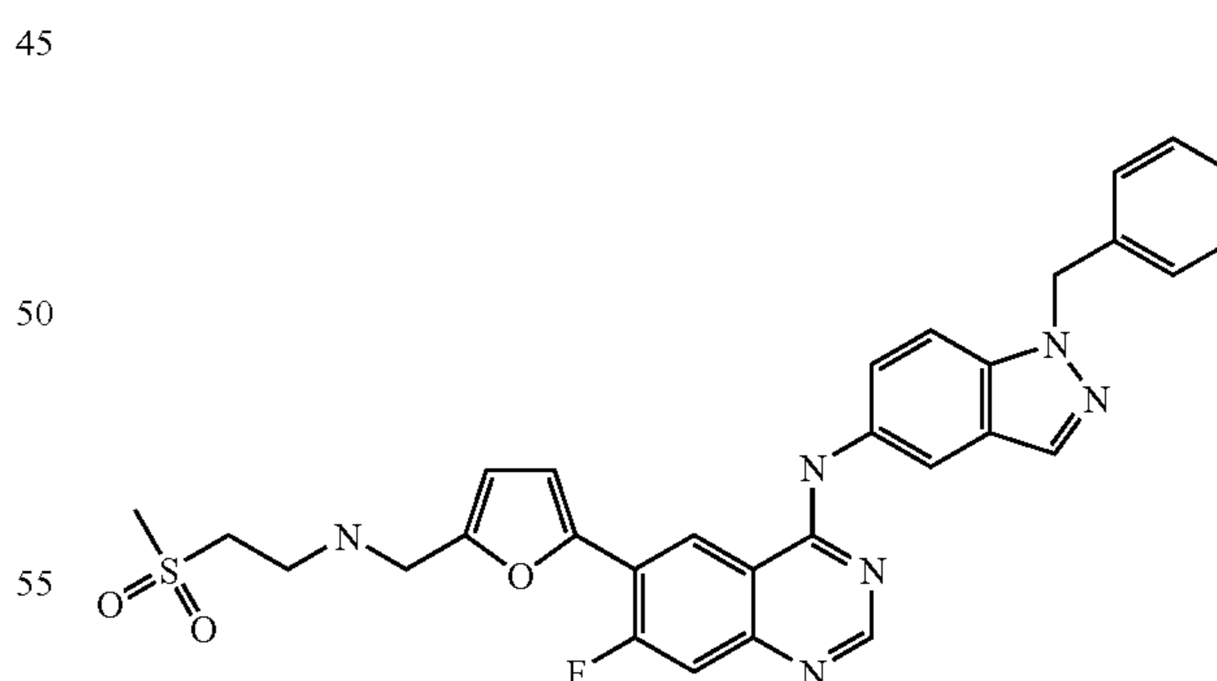
N-(1-Benzyl-1H-indazol-5-yl)-7-fluoro-6-[5-({[2-(methanesulphonyl)ethyl]amino}methyl)-2-furyl]-4-quinazolinamine
