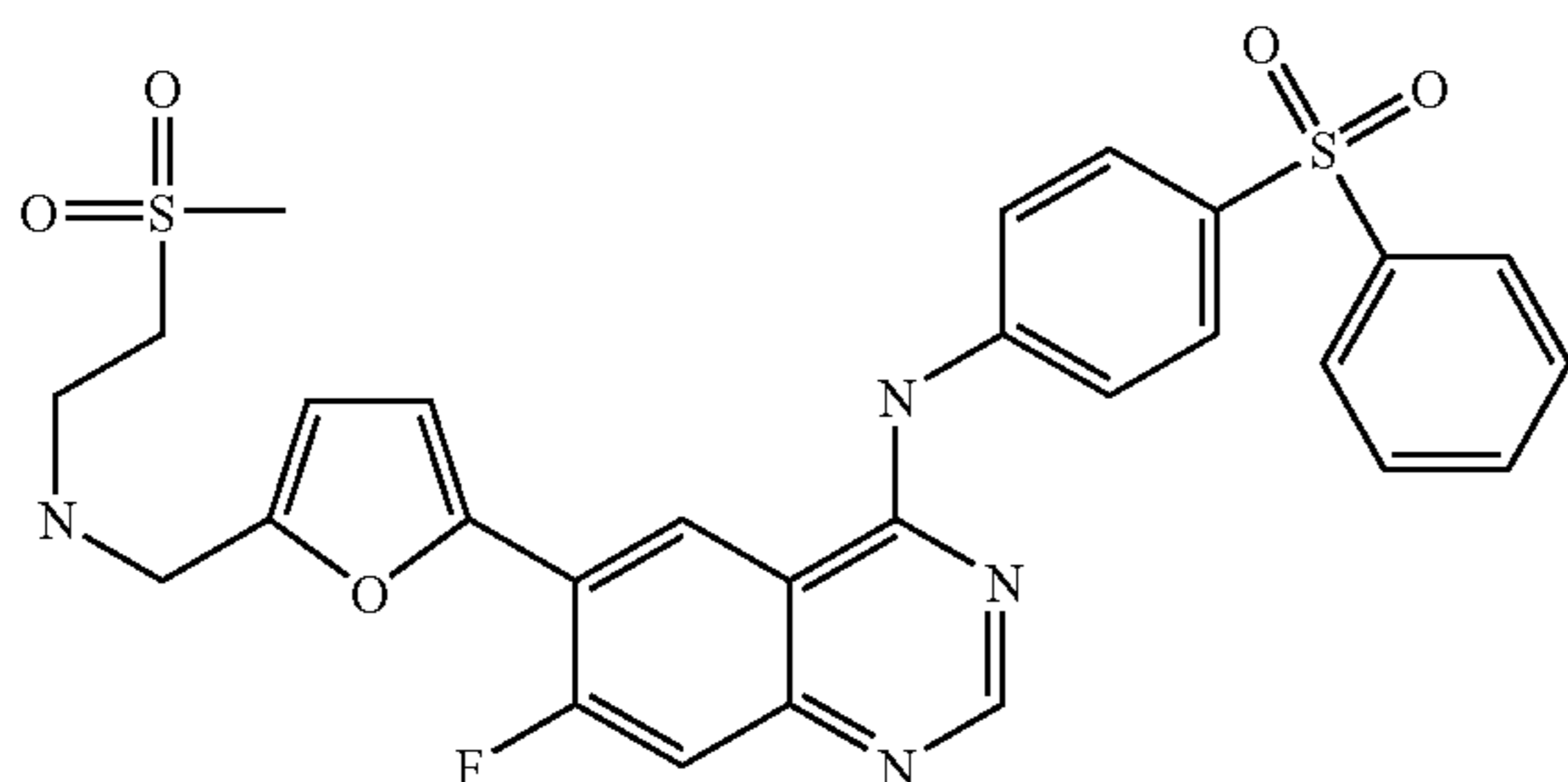
N-[4-(Phenylsulphonyl)phenyl]-7-fluoro-6-[5-({[2-(methanesulphonyl)ethyl]amino}methyl)-2-furyl]-4-quinazolinamine
