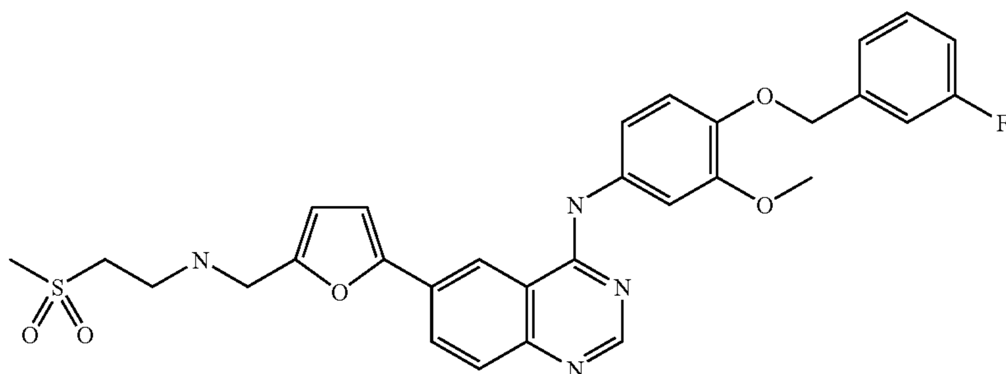
N-{4-[(3-fluorobenzyl)oxy]-3-methoxyphenyl}-6-[5-({[2-(methanesulphonyl)ethyl]amino}methyl)-2-furyl]-4-quinazolinamine
