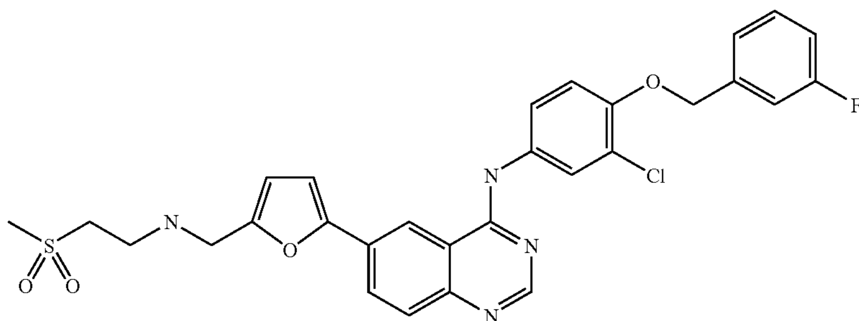
N-{3-Chloro-4-[(3-fluorobenzyl)oxy]phenyl}-6-[[2-(methanesulphonyl)ethyl]amino]methyl-2-furyl]-4-quinazolinamine
