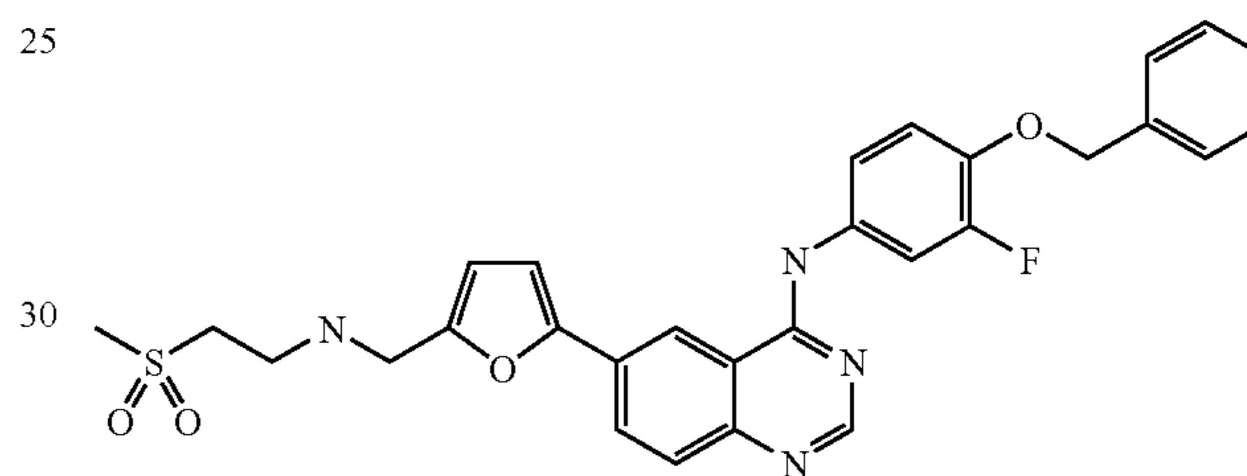
N-(3-Fluoro-4-benzyloxyphenyl)-6-[5-({2-(methanesulphonyl)ethyl}amino)methyl]-4-furyl]-4-quinazolinamine
