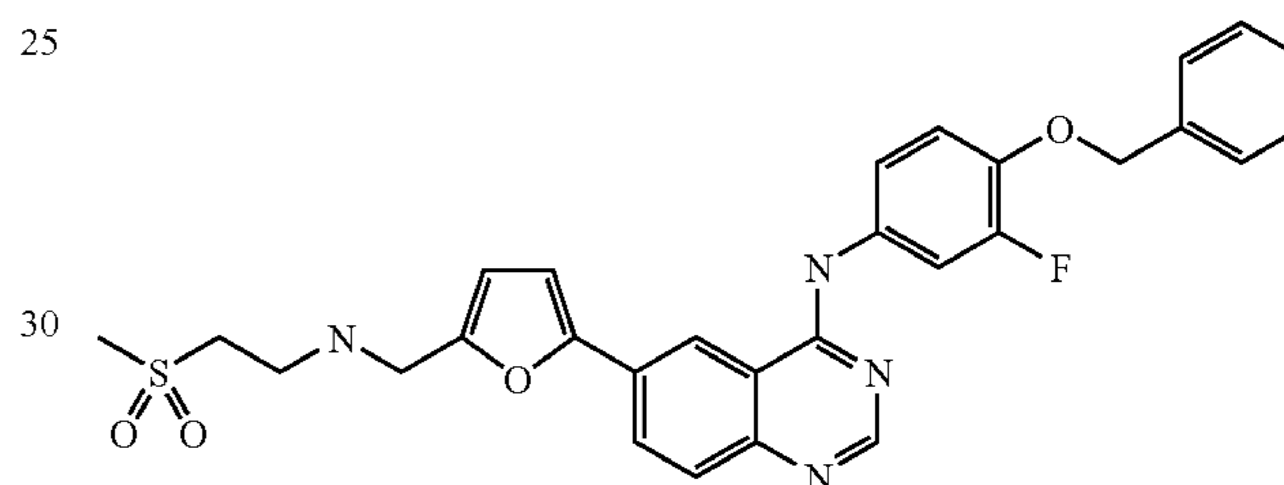
N-(3-Fluoro-4-benzyloxyphenyl)-6-[5-({2-(methanesulphonyl)ethyl}amino)methyl]-4-furyl]-4-quinazolinamine
