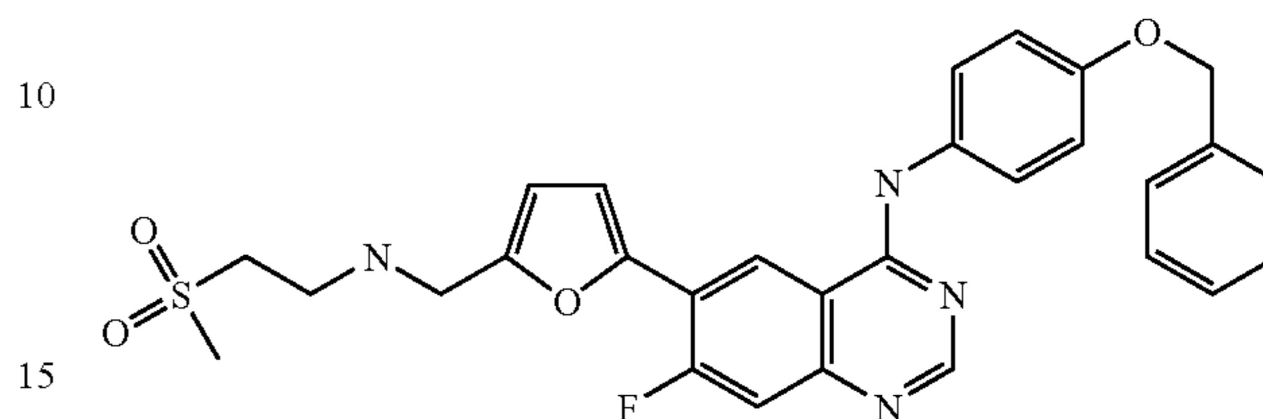
N-[4-(Benzyloxy)phenyl]-7-fluoro-6-[5-({[2-(methanesulphonyl)ethyl]amino}methyl)-2-furyl]-4-quinazolinamine
