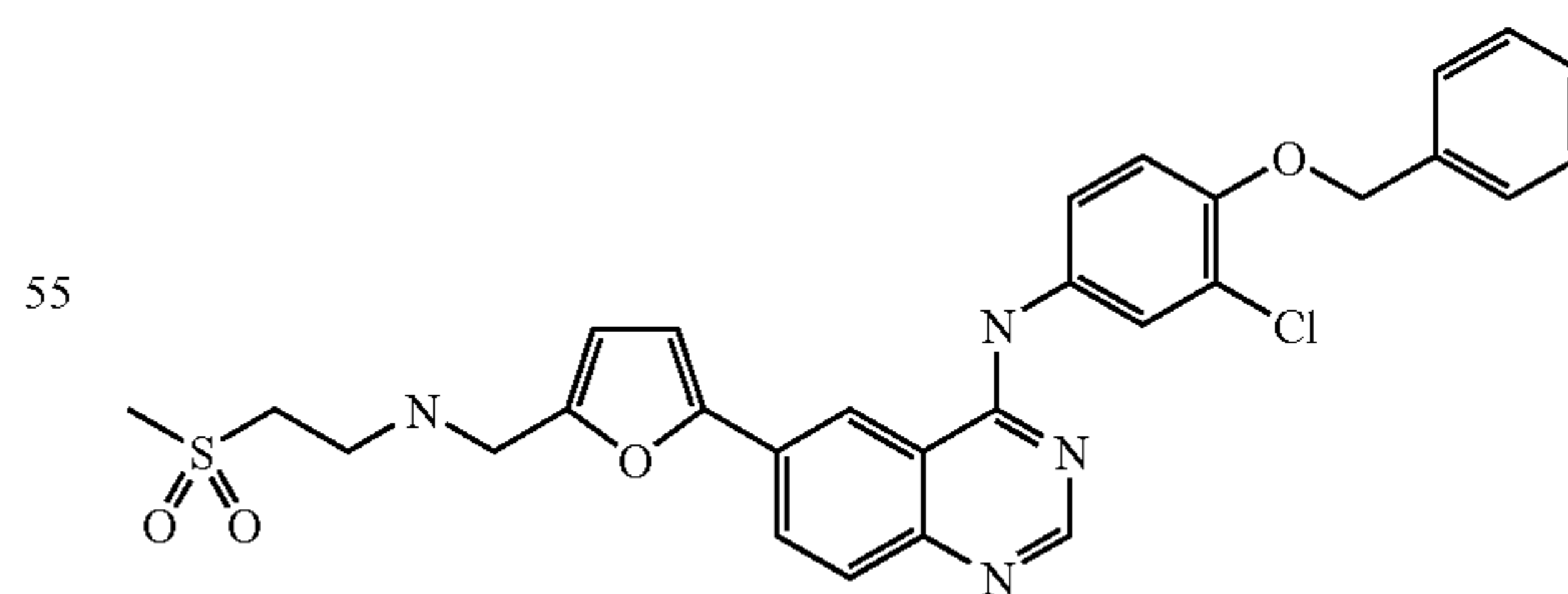
N-(3-Chloro-4-benzyloxyphenyl)-6-[5-({2-(methanesulphonyl)ethyl}amino)methyl]-4-furyl]-4-quinazolinamine
