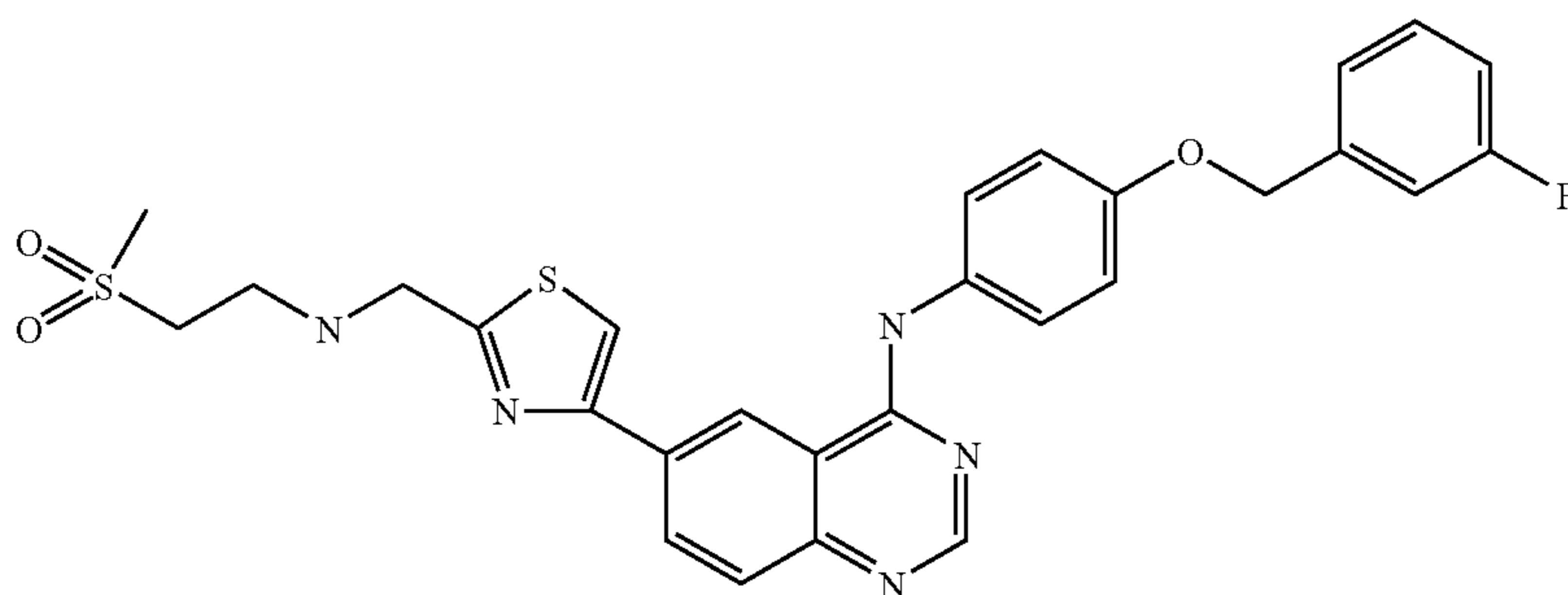
N-{4-[(3-fluorobenzyl)oxy]phenyl}-6-[2-({[2-(methanesulphonyl)ethyl]amino}methyl)-1,3-thiazol-4-yl]-4-quinazolinamine
