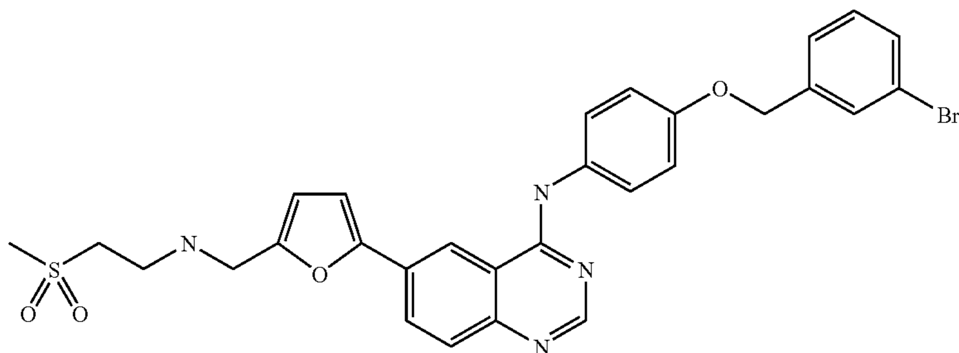
N-{4-[(3-bromobenzyl)oxy]phenyl}-6-[5-({[2-(methanesulphonyl)ethyl]amino}methyl)-2-furyl]-4-quinazolinamine
