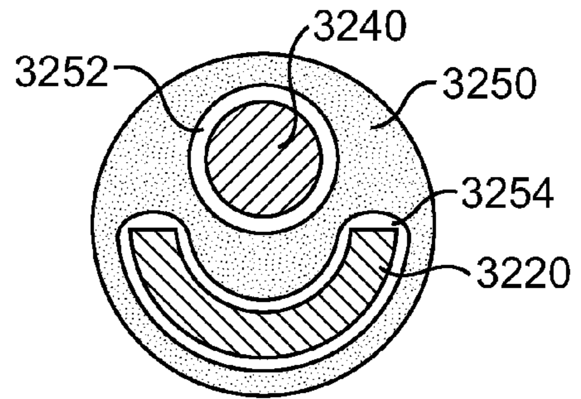
SECTION A-A
