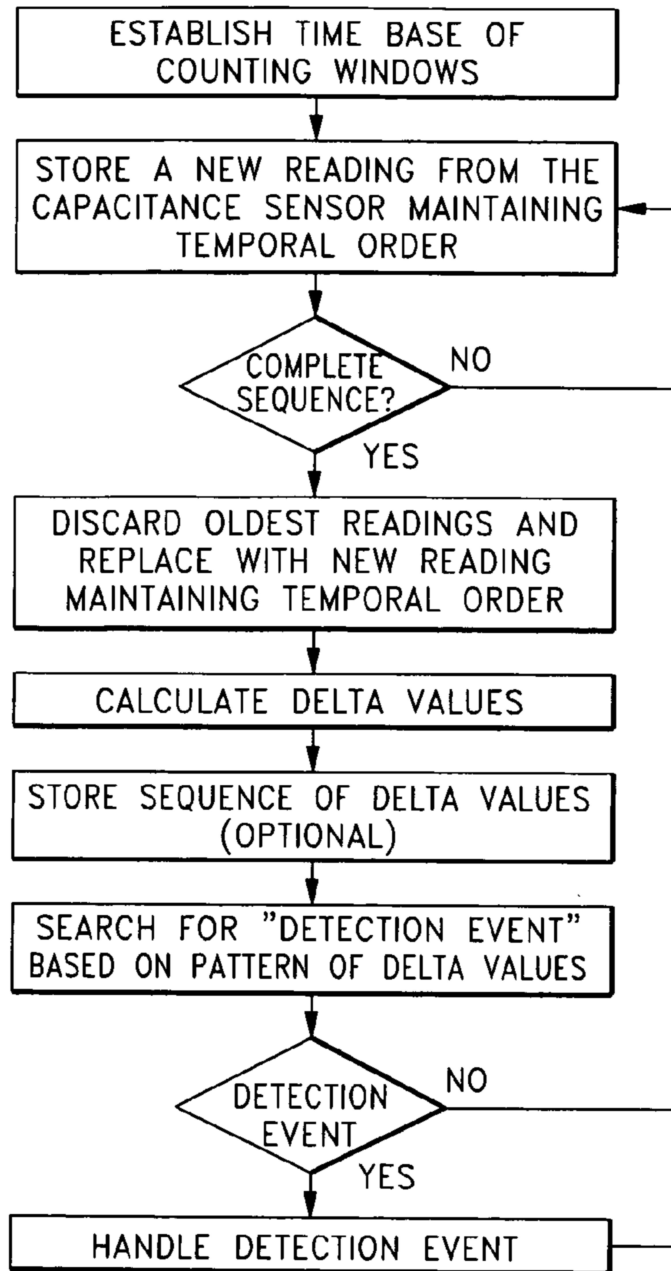
Fig. 18
