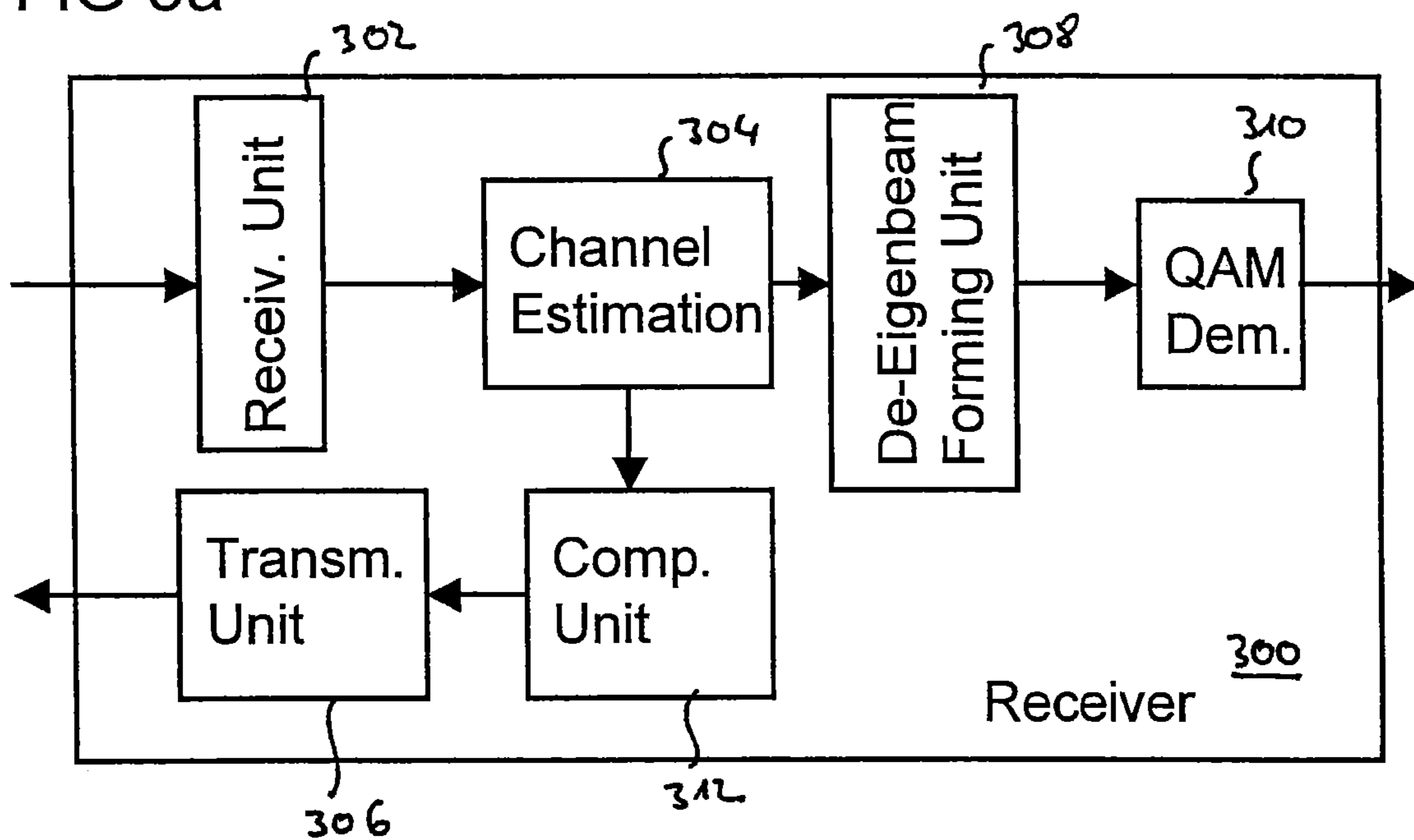
FIG 3a
