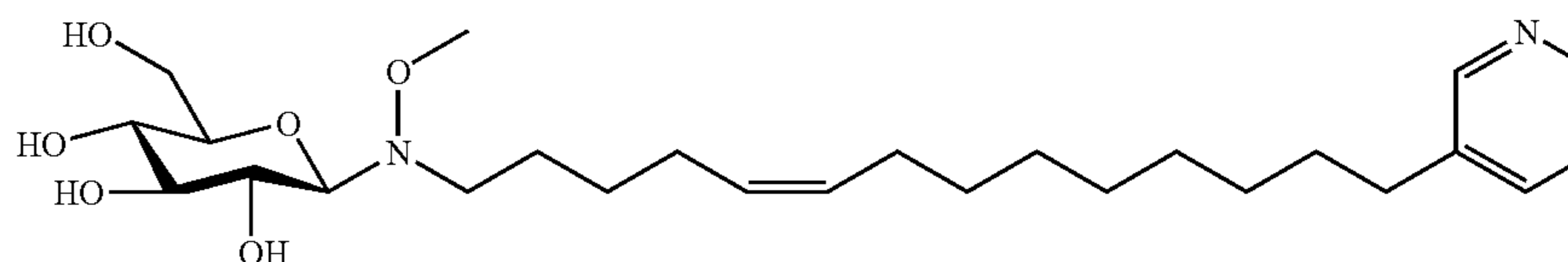
Amphlmedoside E
