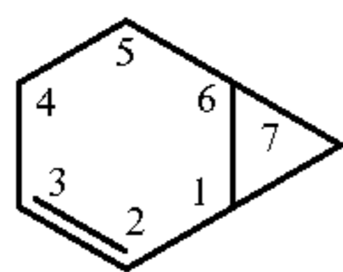
[4.1.0]
