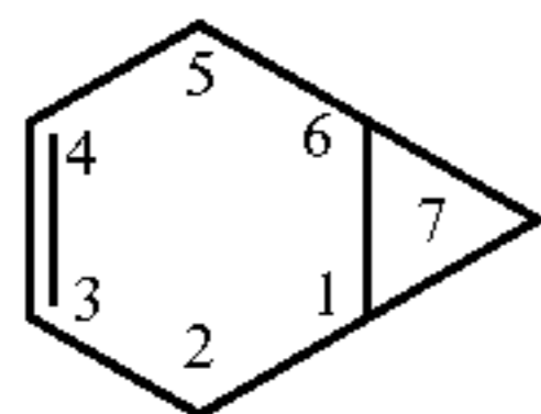
[4.1.0]
