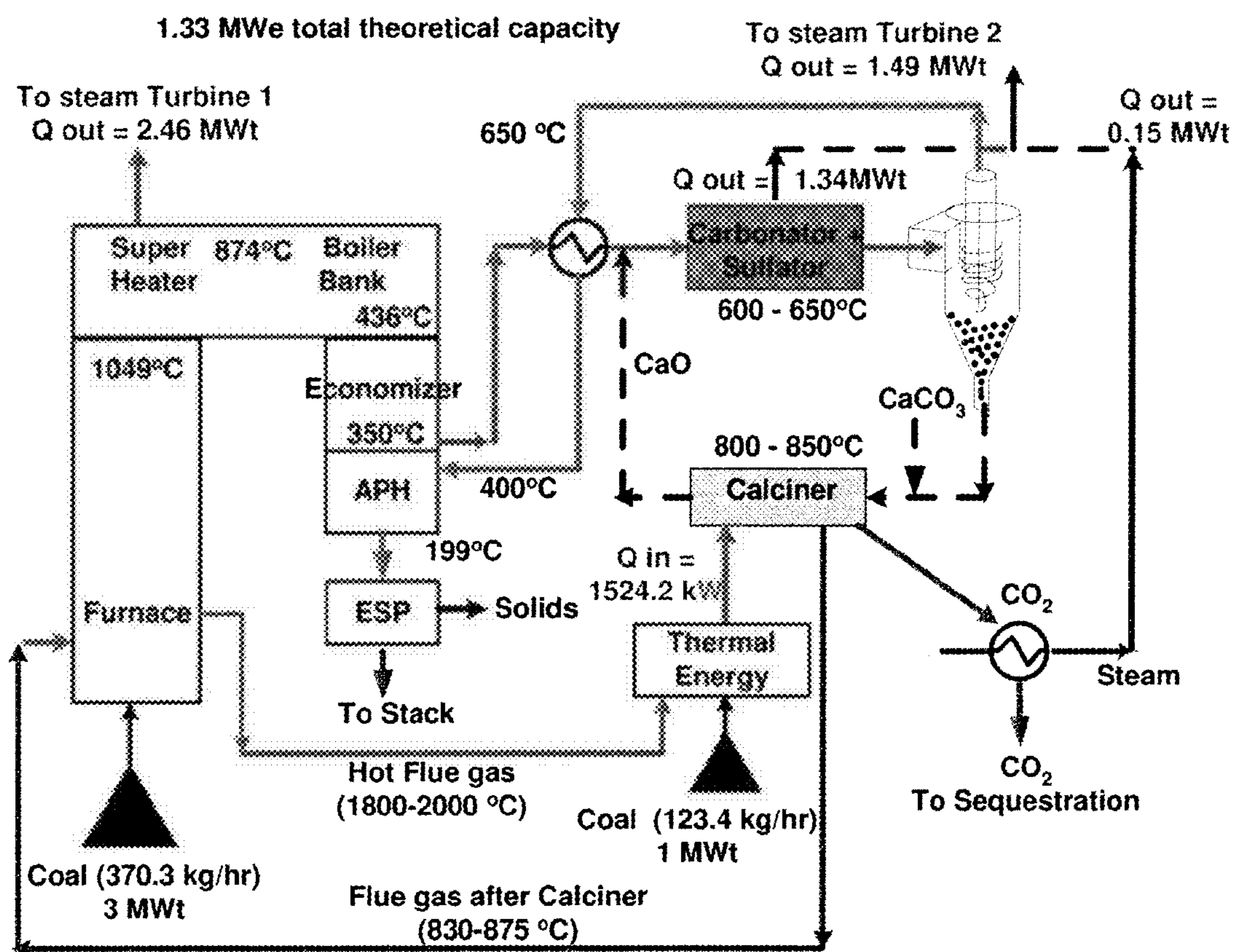
FIG. 29
