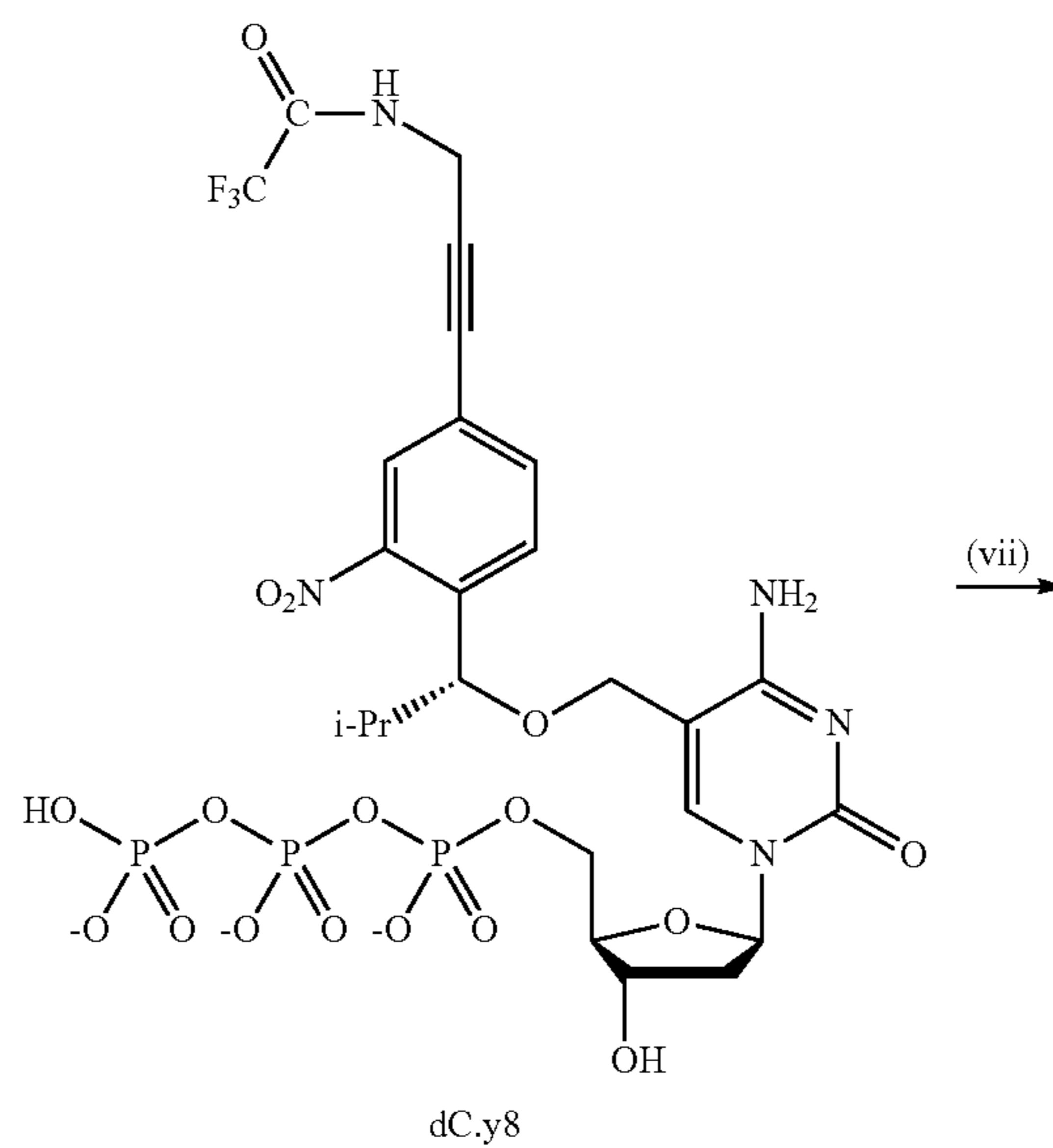
Scheme 16.
