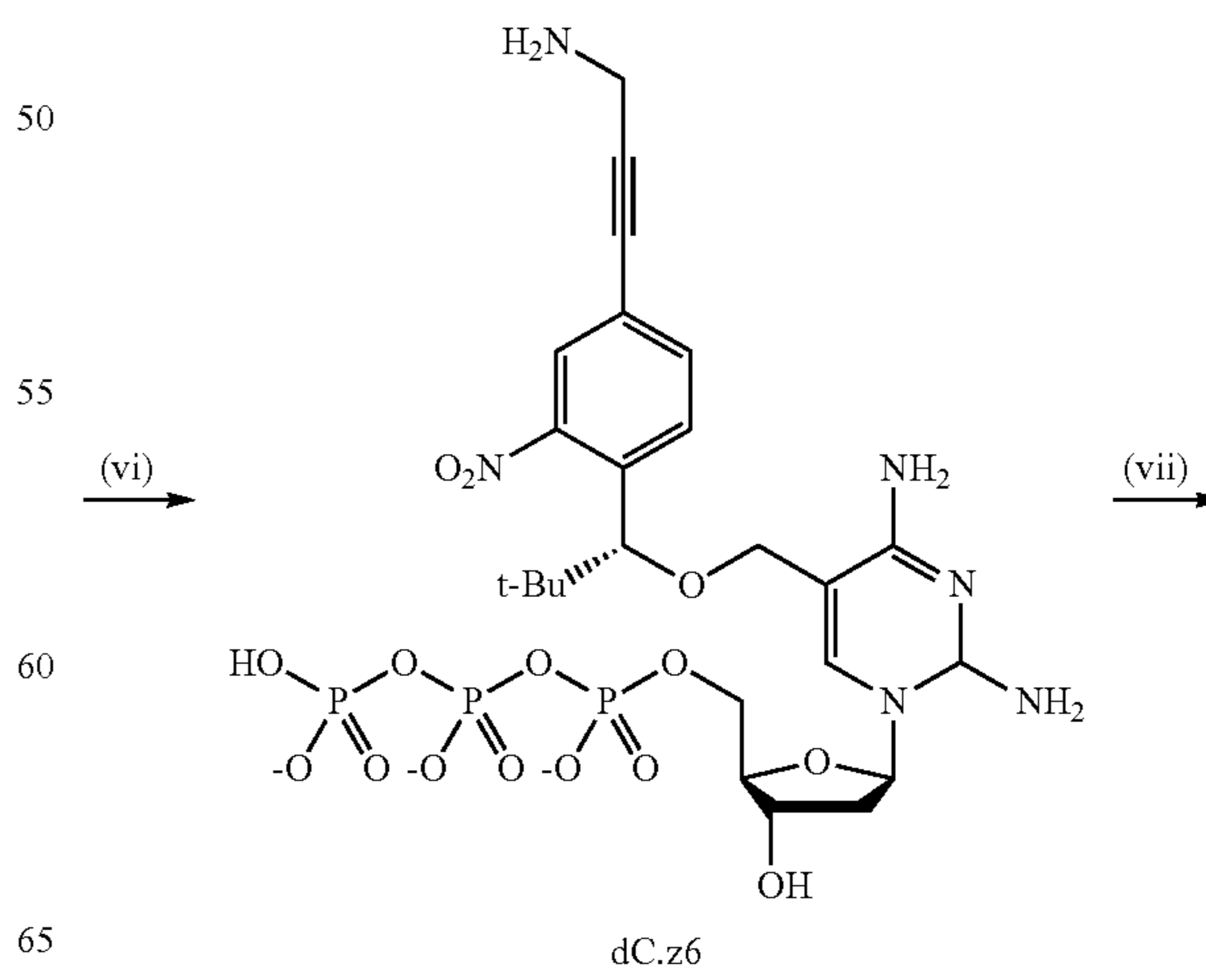
Scheme 18.
