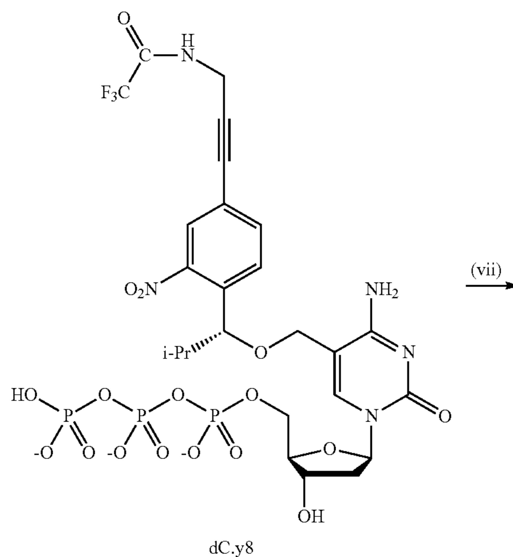
Scheme 16.
