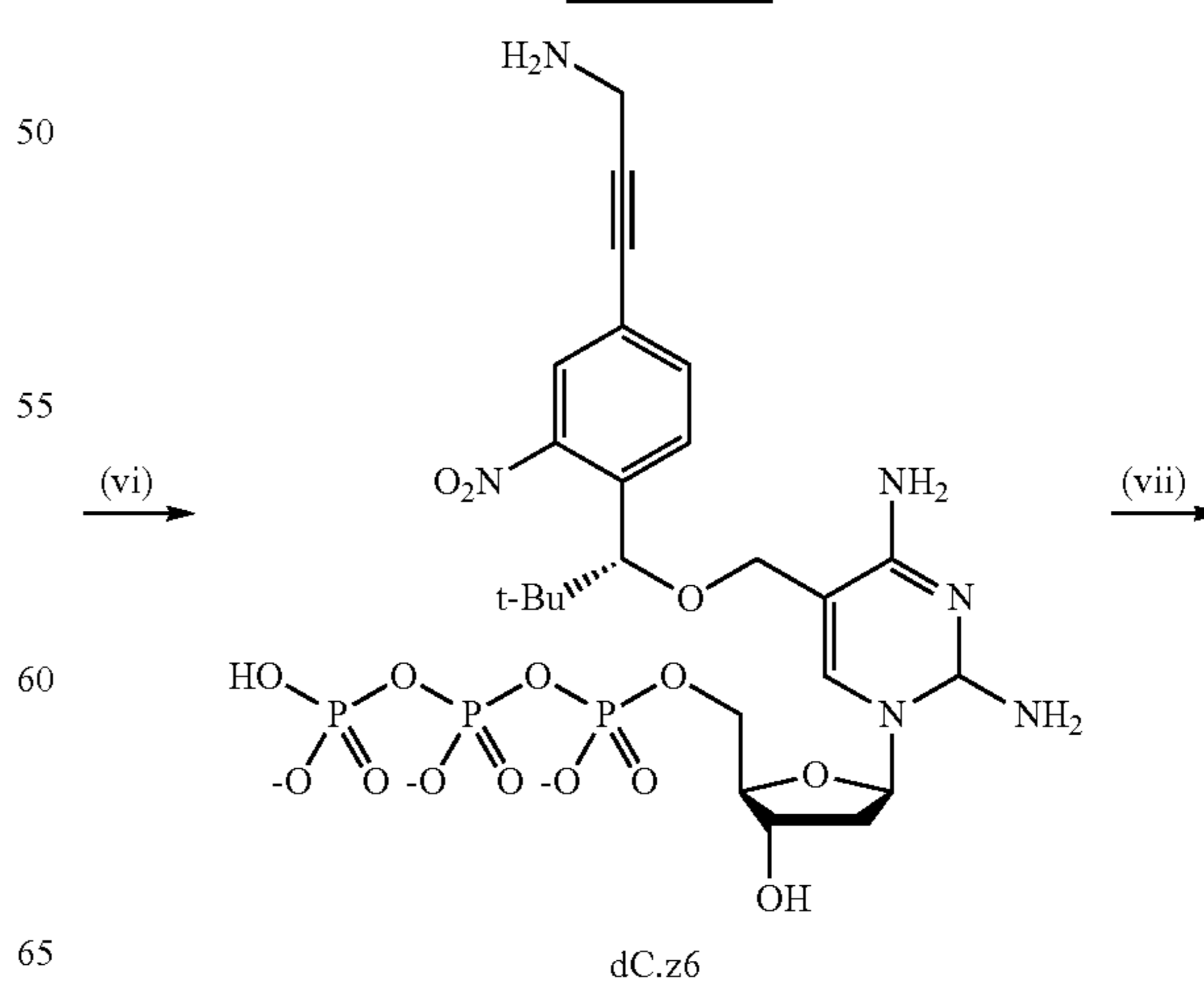
Scheme 18.
