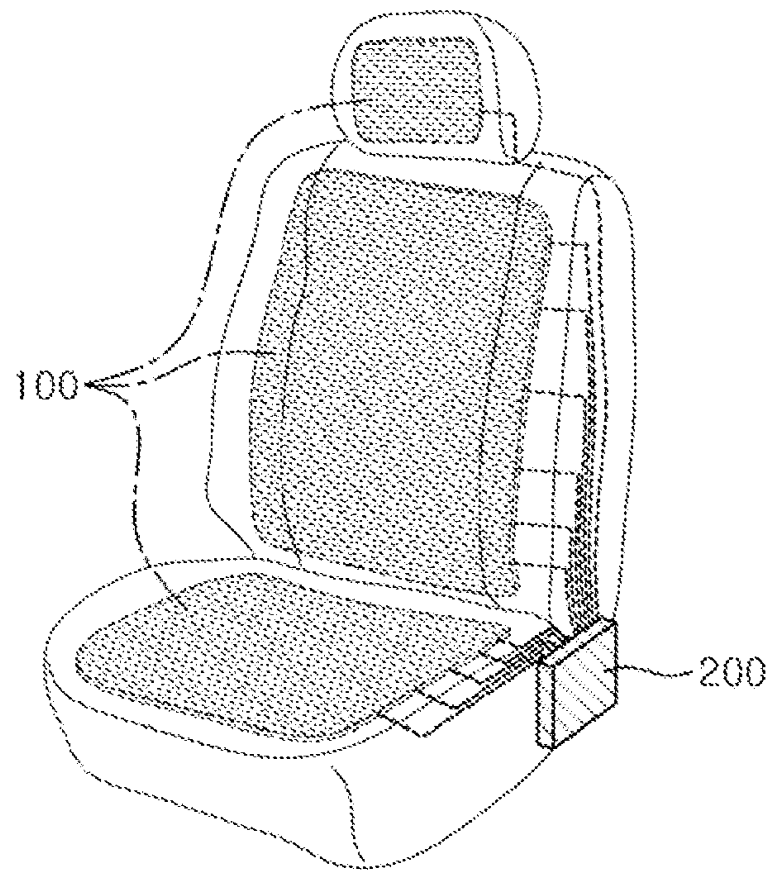
FIG. 2C
