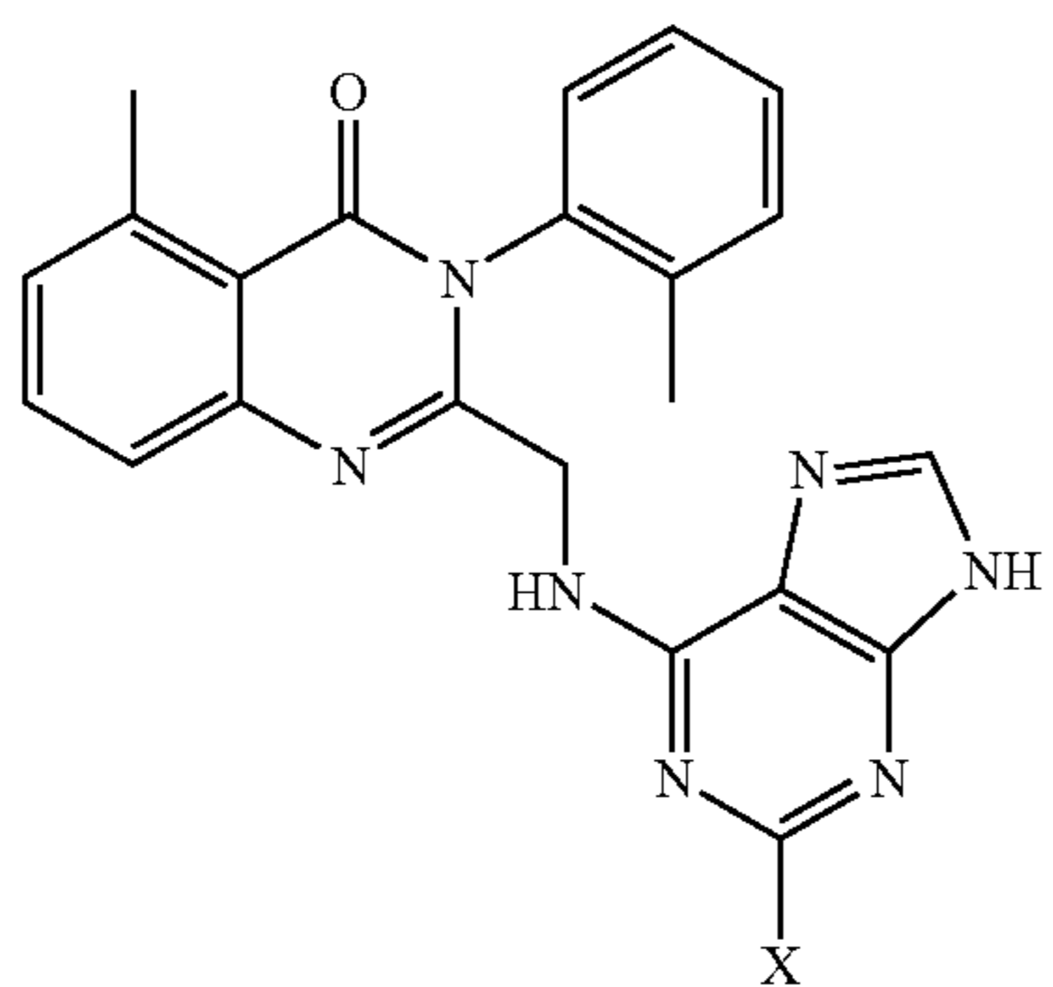
5e
