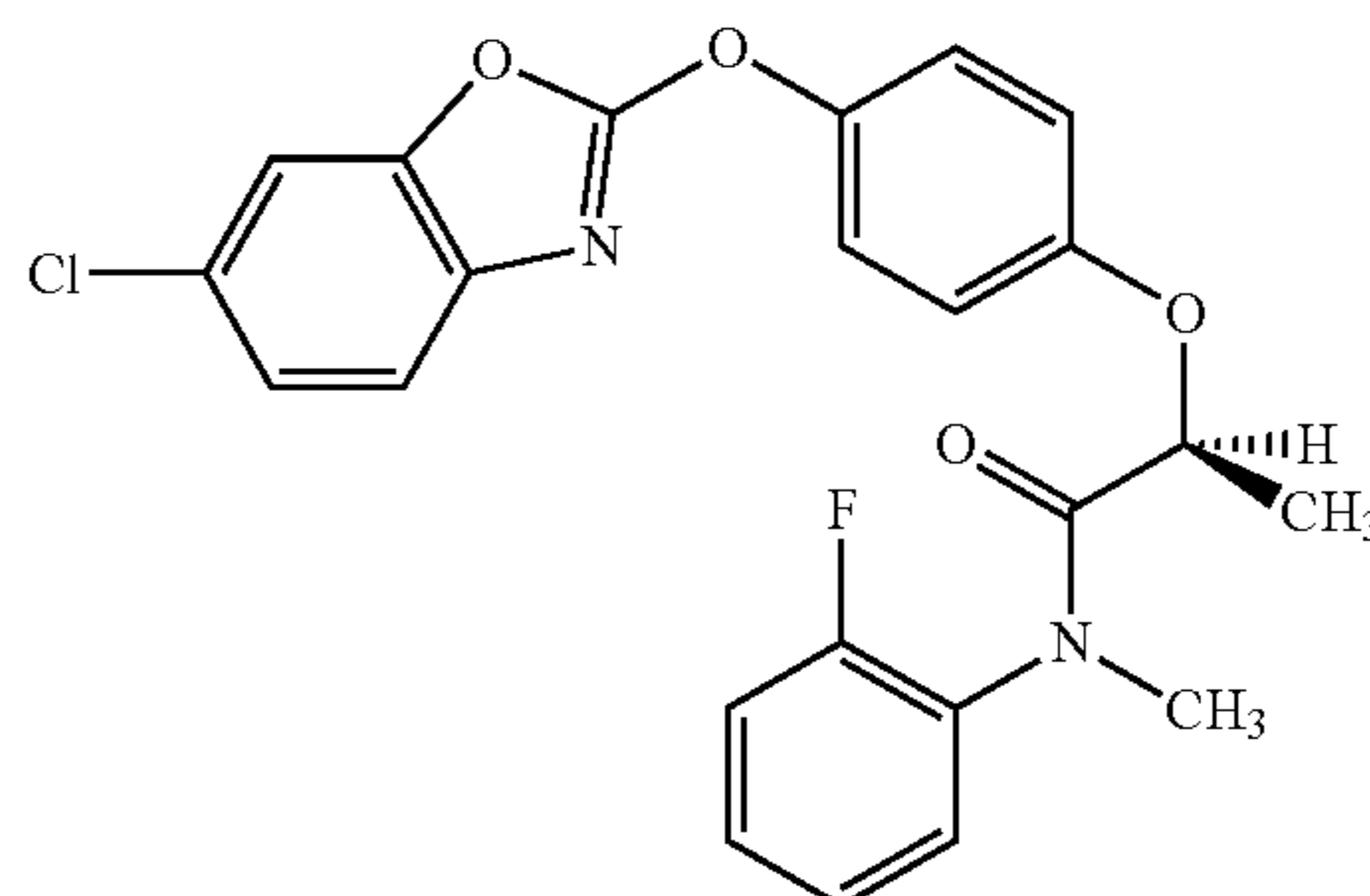
(2S)-2-{4-[(6-chloro-1,3-benzoxazol-2-yl)oxy]phenoxy}-N-(2-fluorophenyl)-N-methylpropanamide
