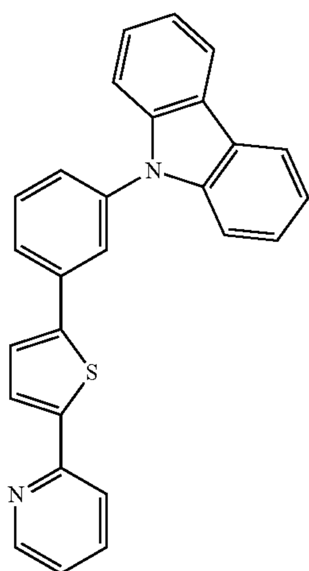
Ligand B
