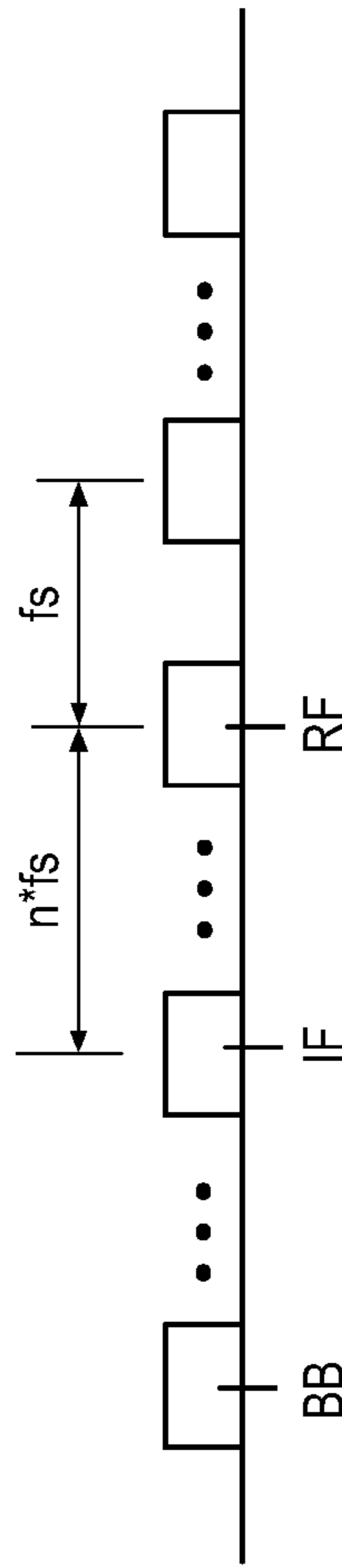
FIG. 113 S&H output 1 426
