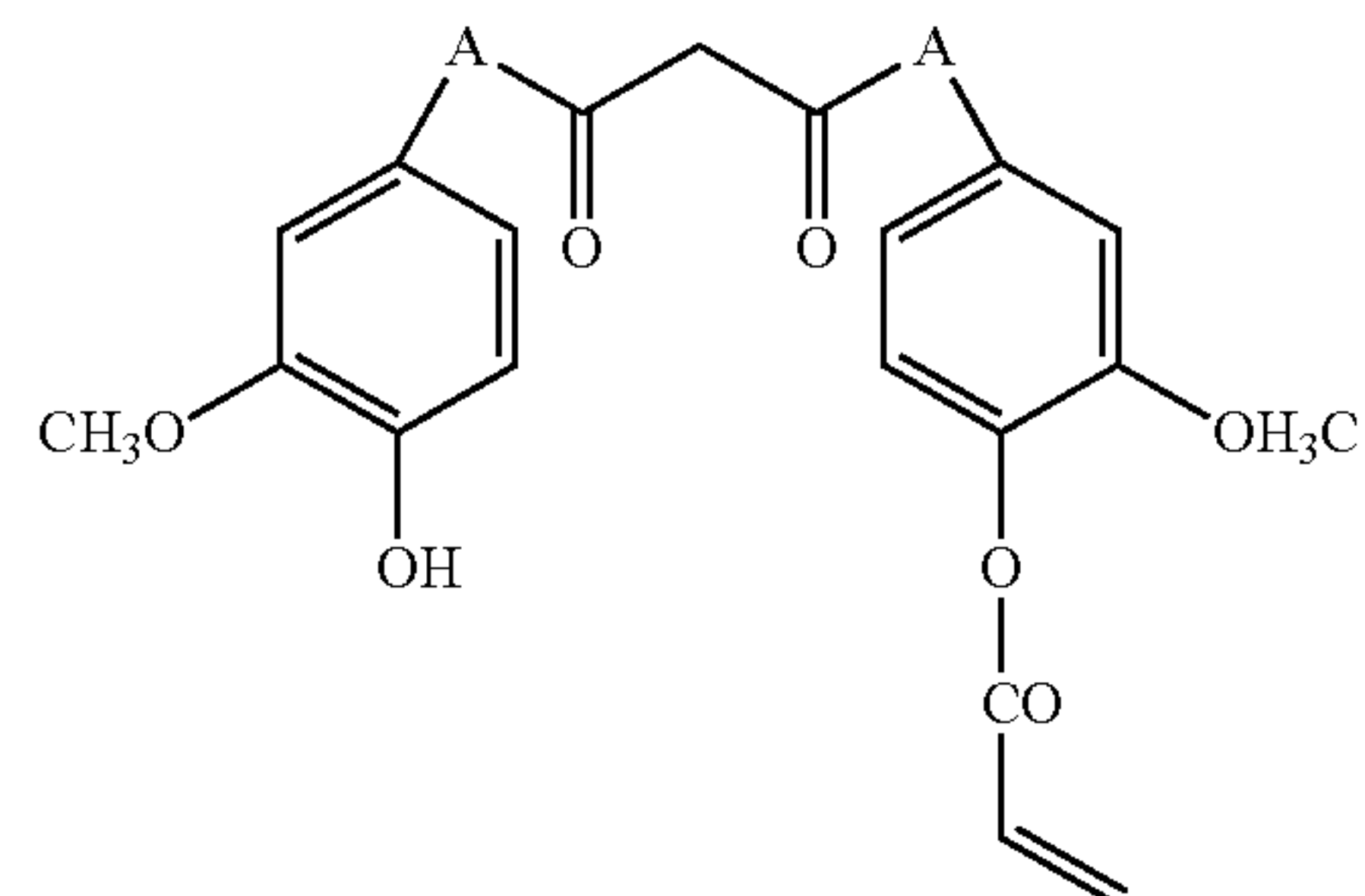
a) Curcumin Acrylate
