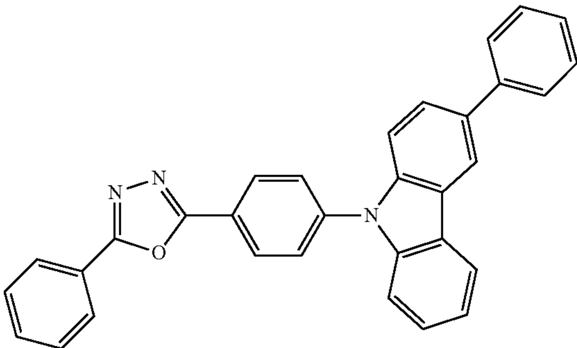
(CO11-II)
