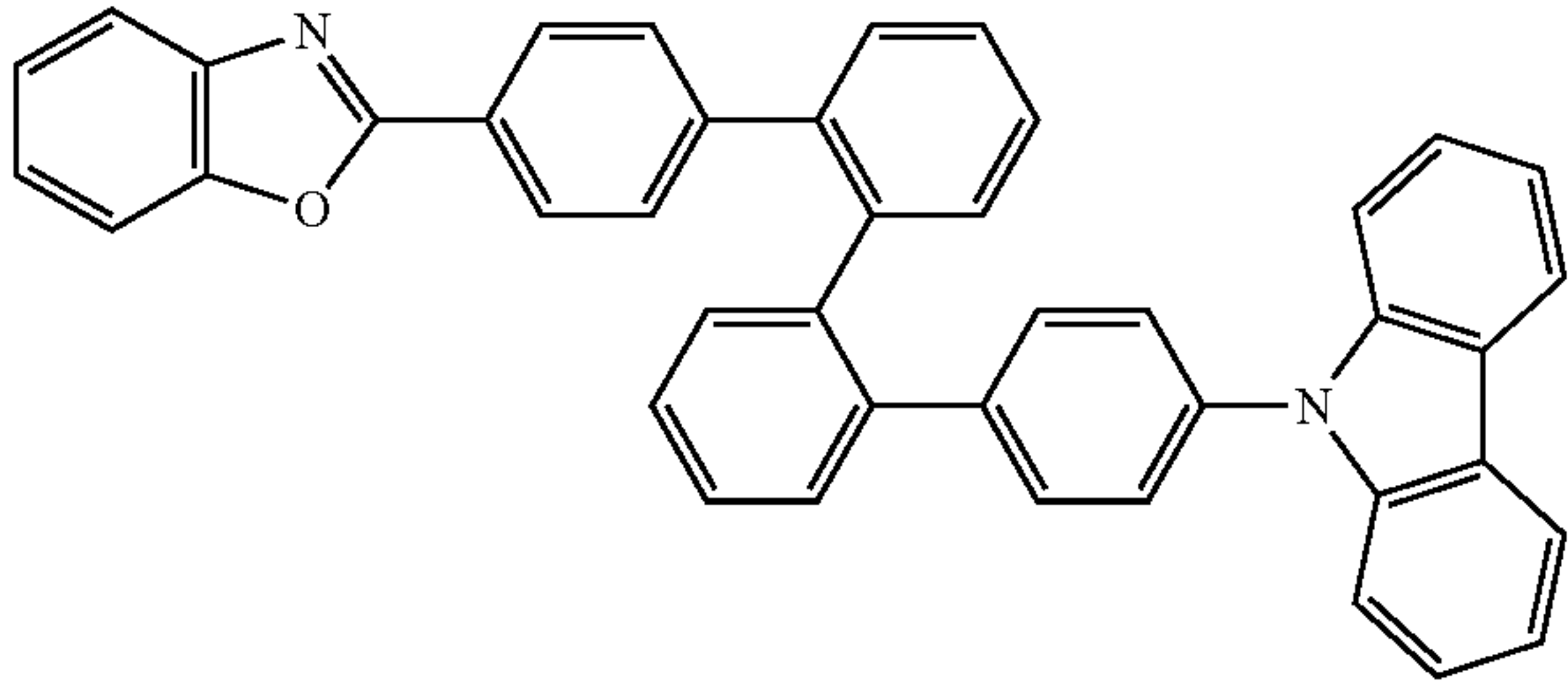
(Z-CzPBOx)
