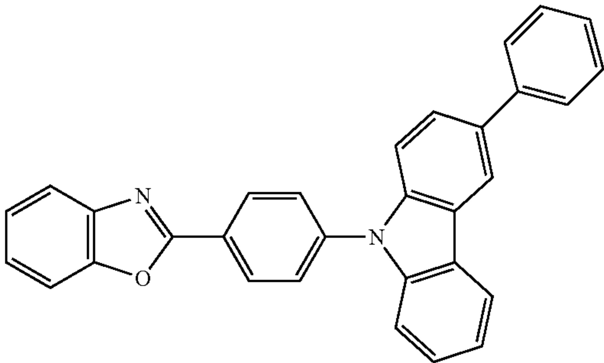
(CzBOx-II)
