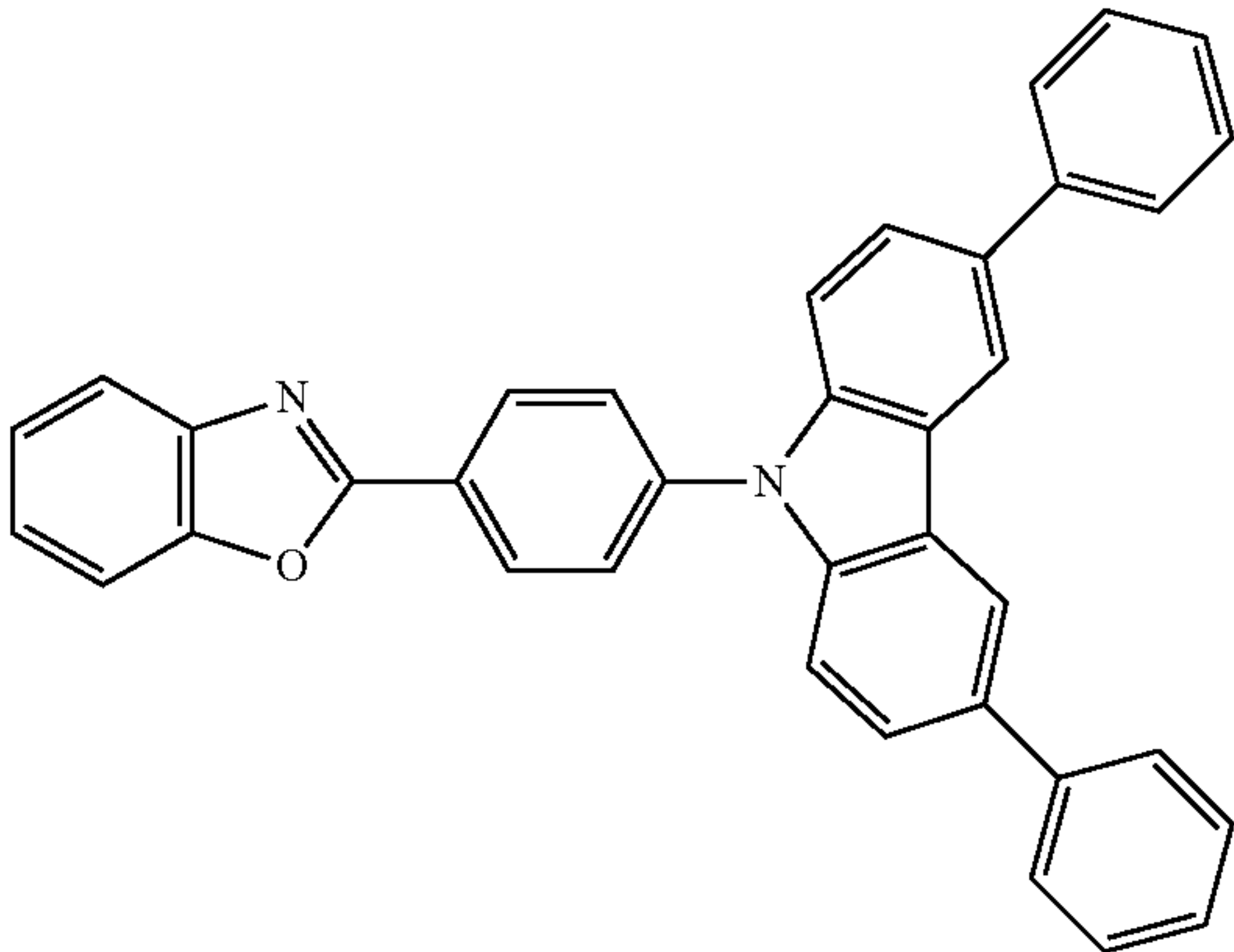
(CzBOx-III)
