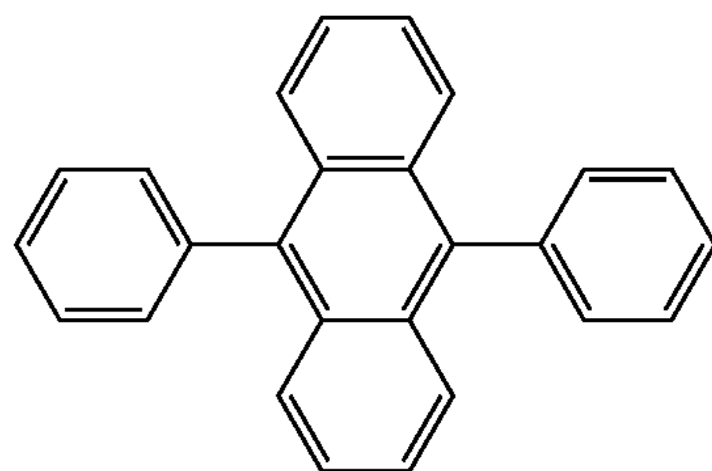
(DPAnth)
