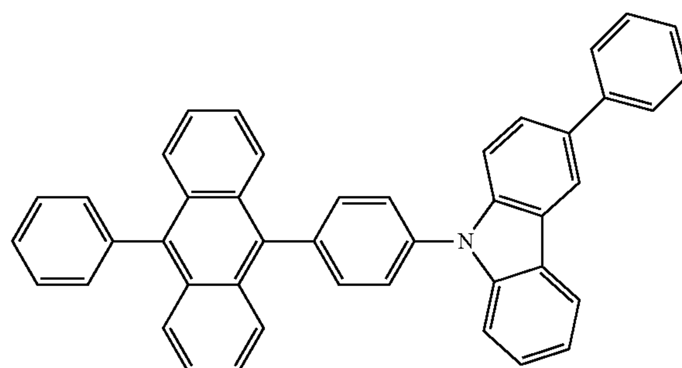
(CzPAP)
