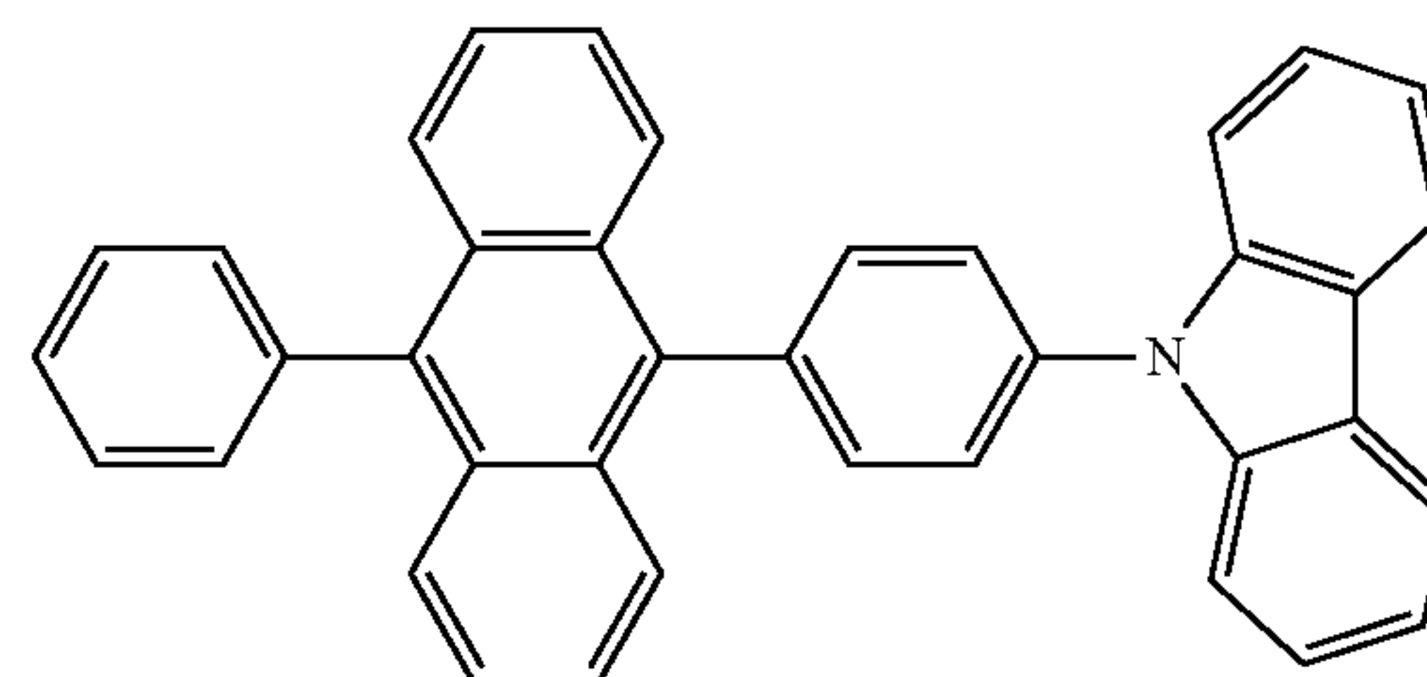
(CzPA)
