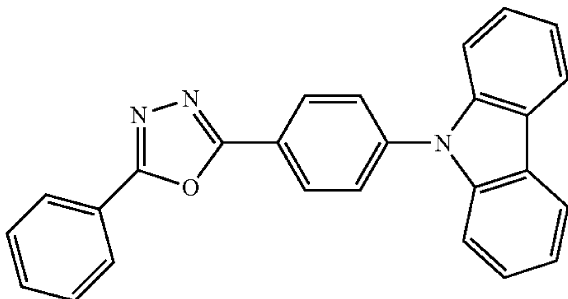
(CO11)
