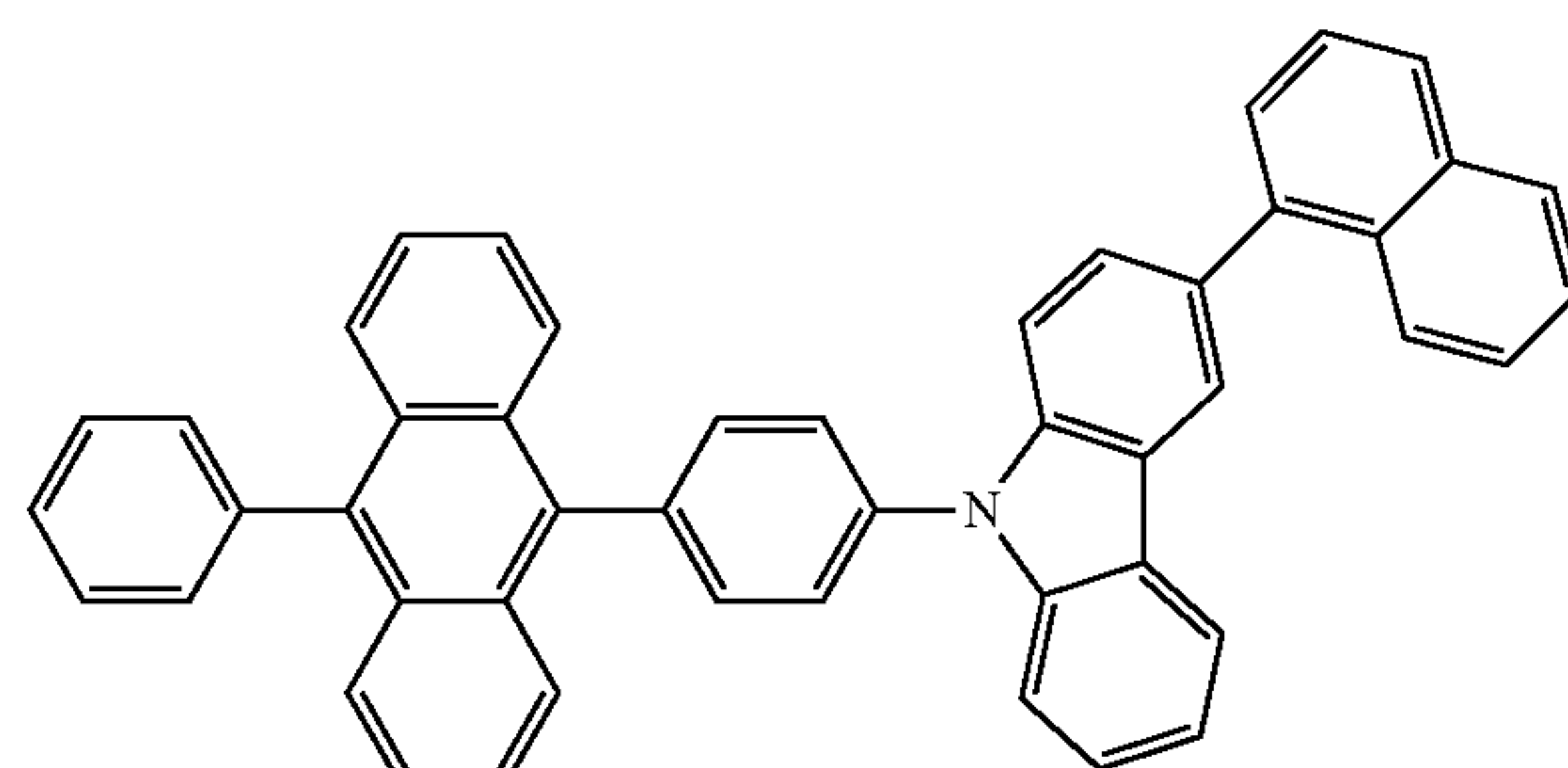
(CzPAαN)
