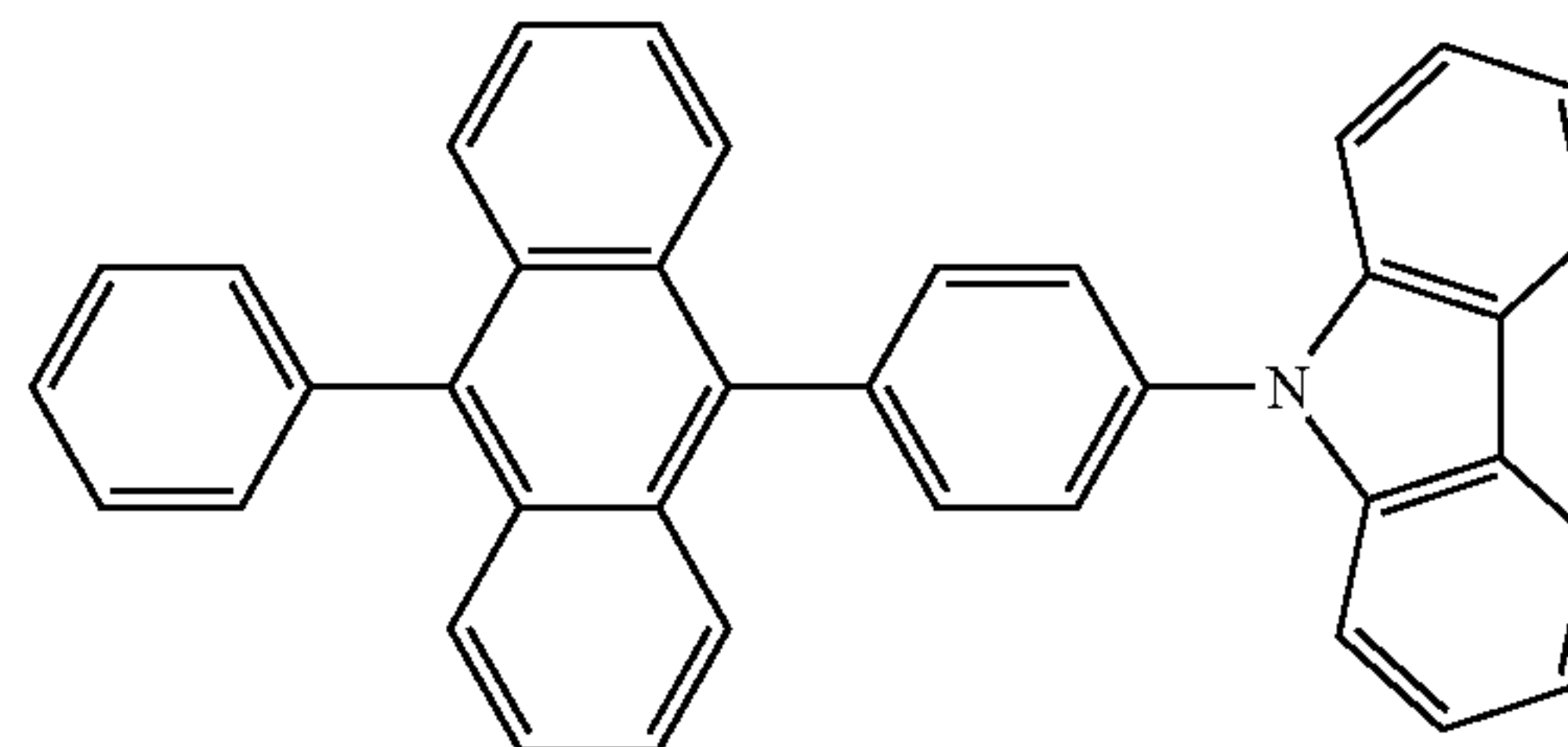
CzPA
