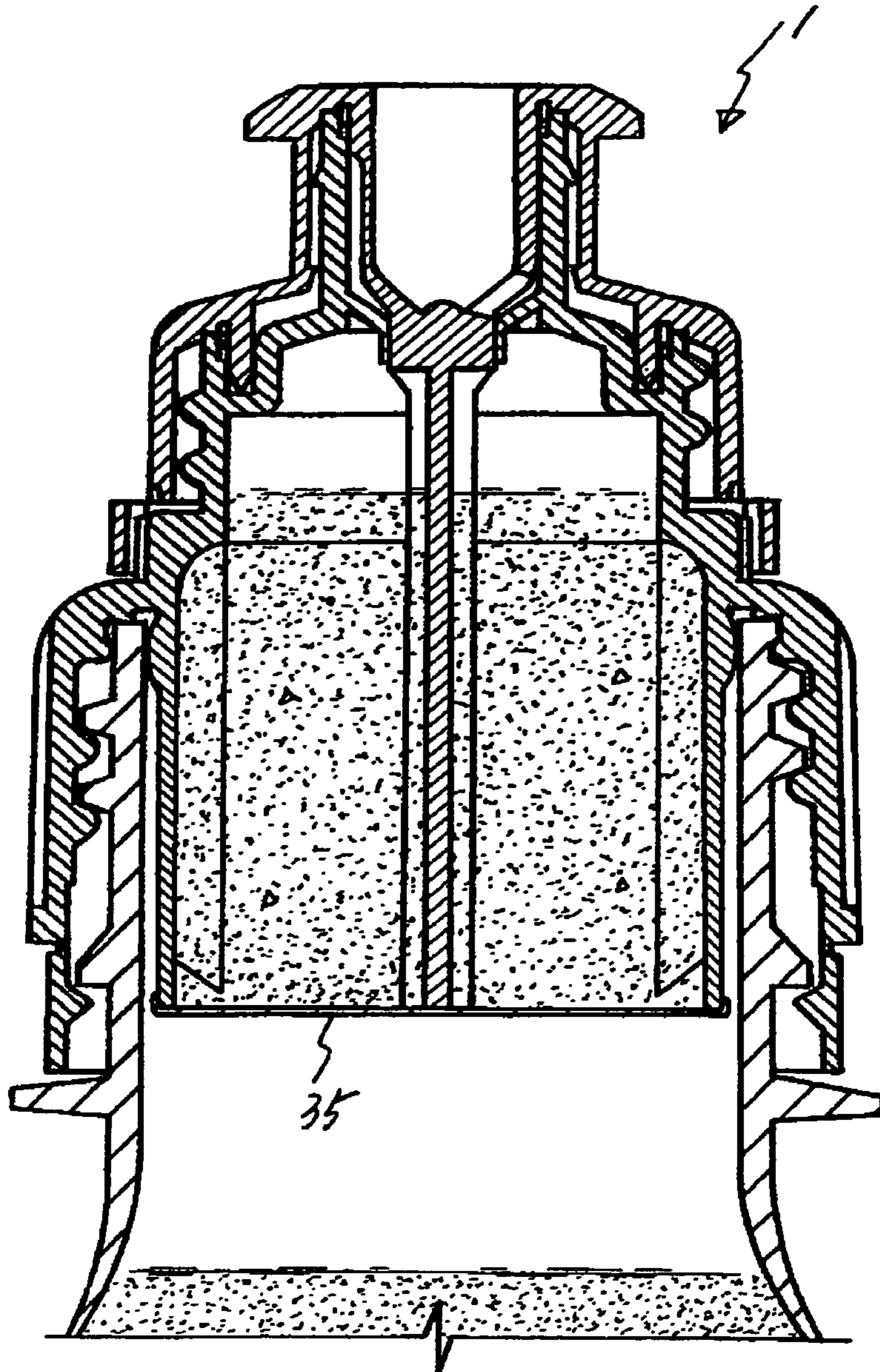
Fig. 6
