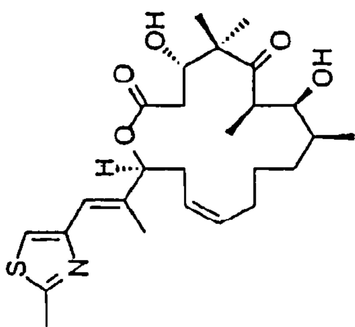
desoxyepothilone A
