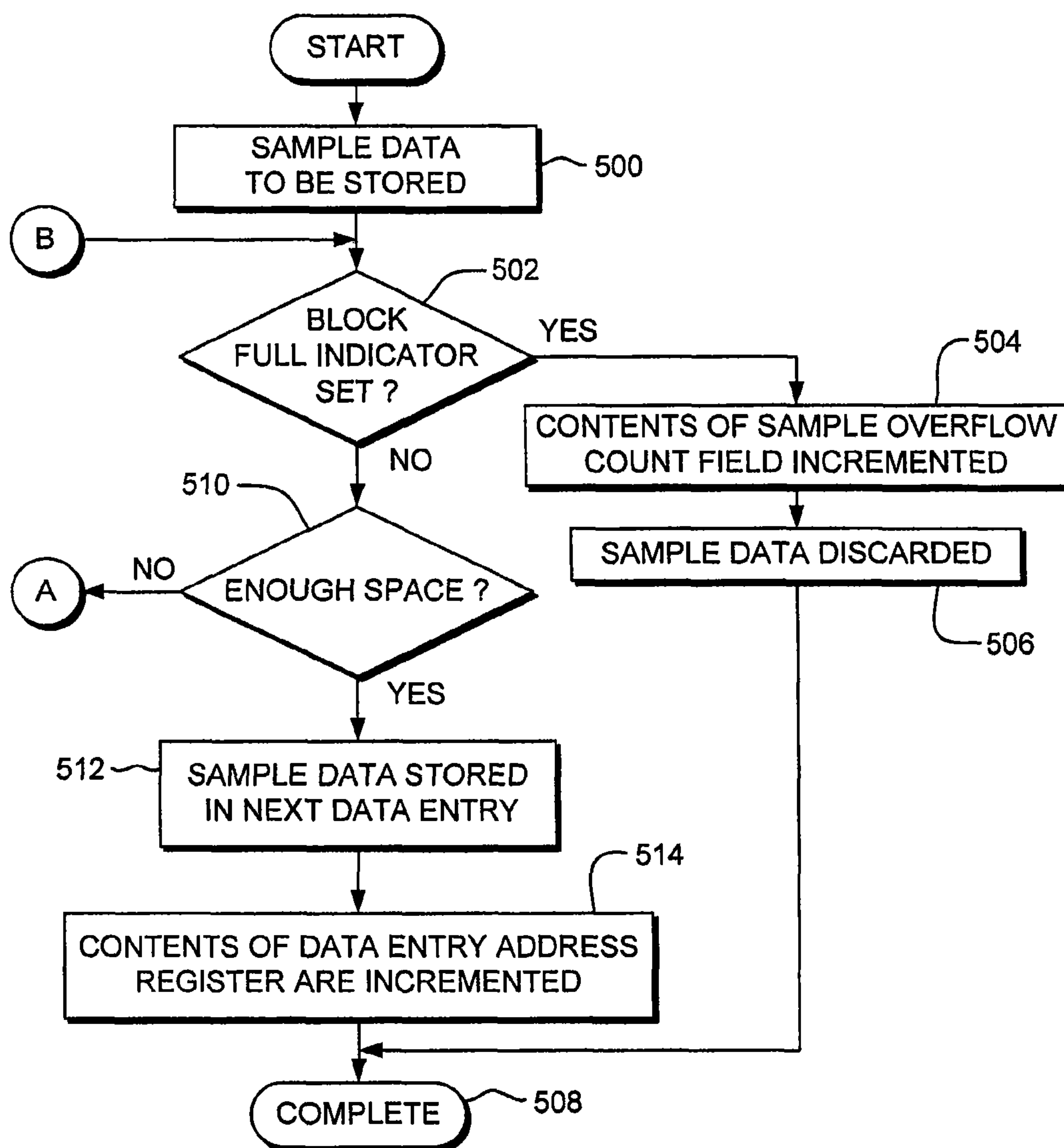
FIG. 5A
