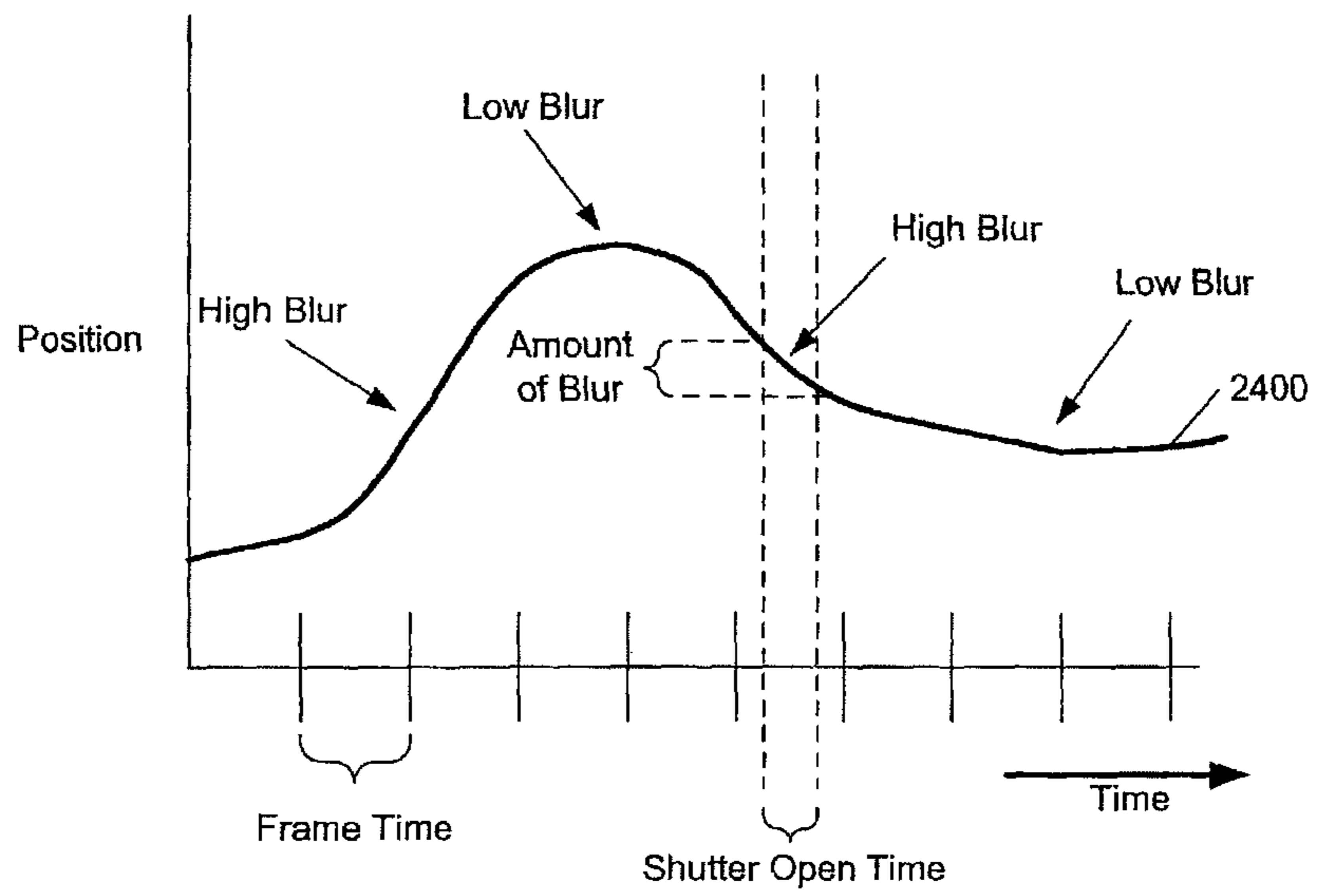
FIG. 24
