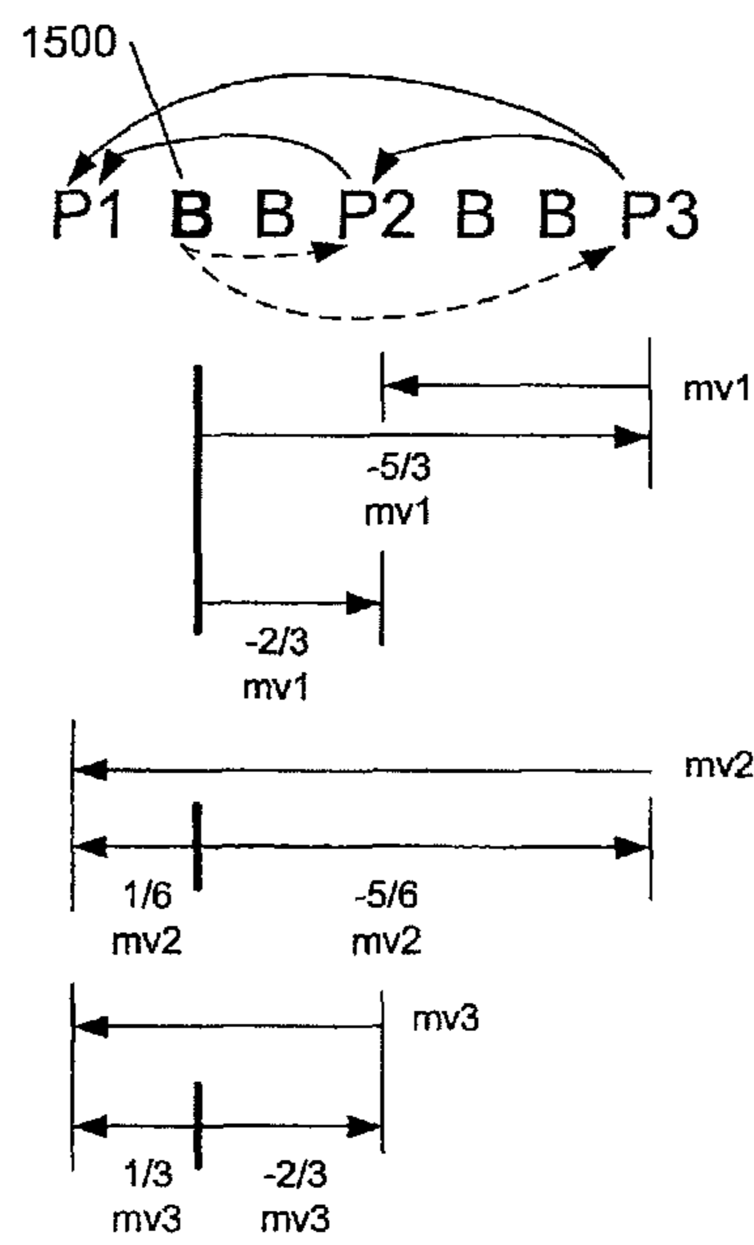
FIG. 15
