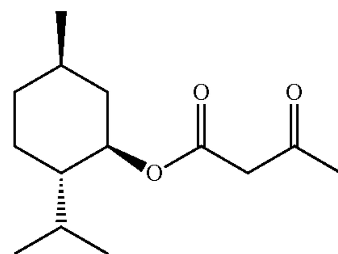
[Chem. 3]
