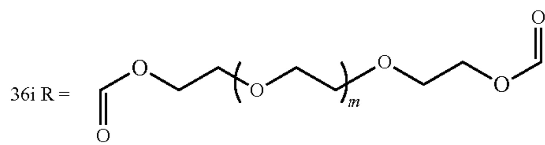
Poly(CDDCys-CB-PEG)
