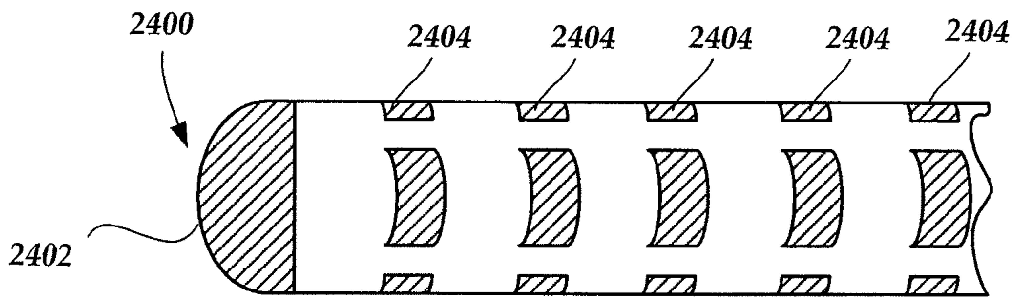
FIG. 23
