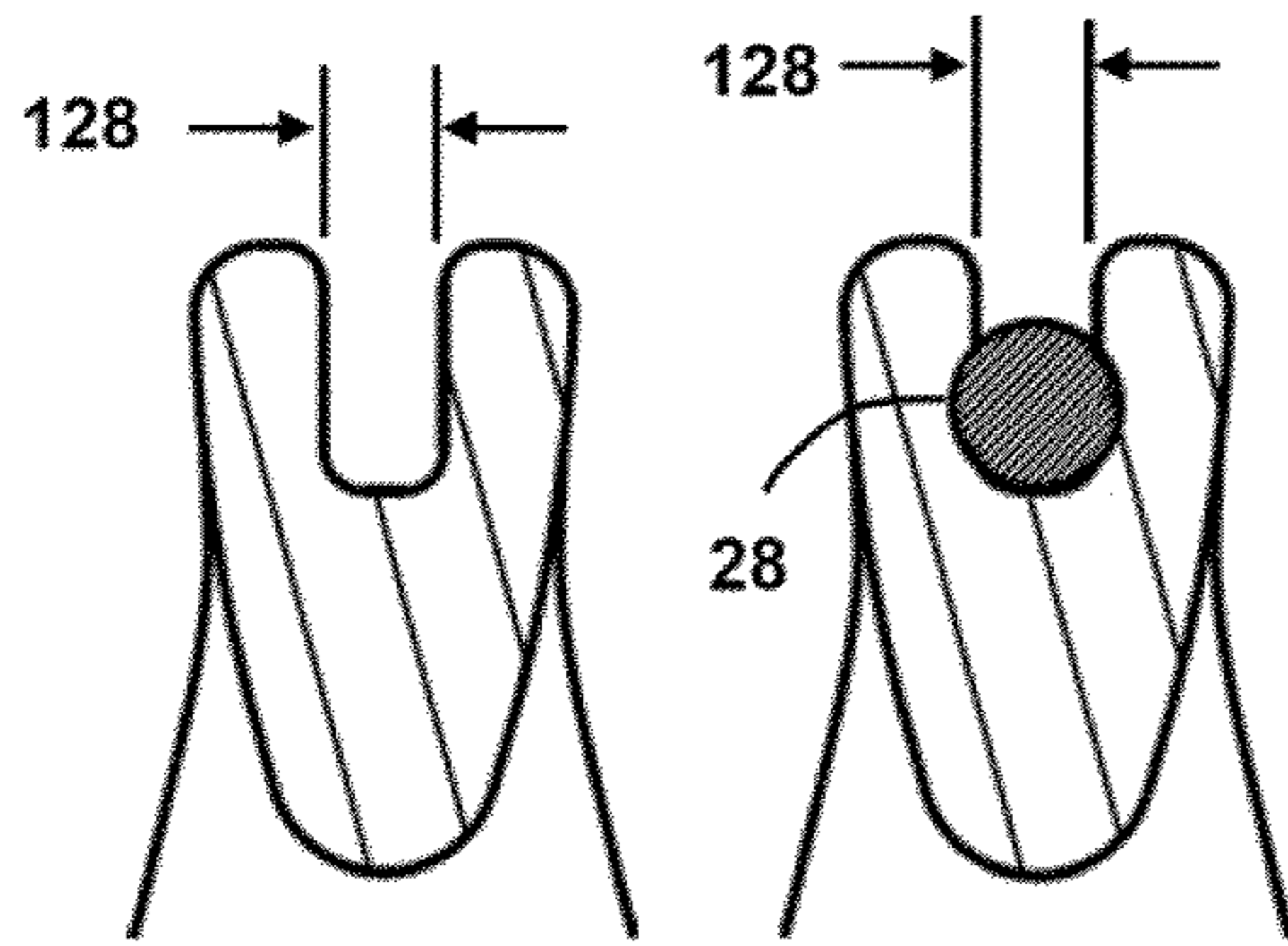
SECTION D-D
