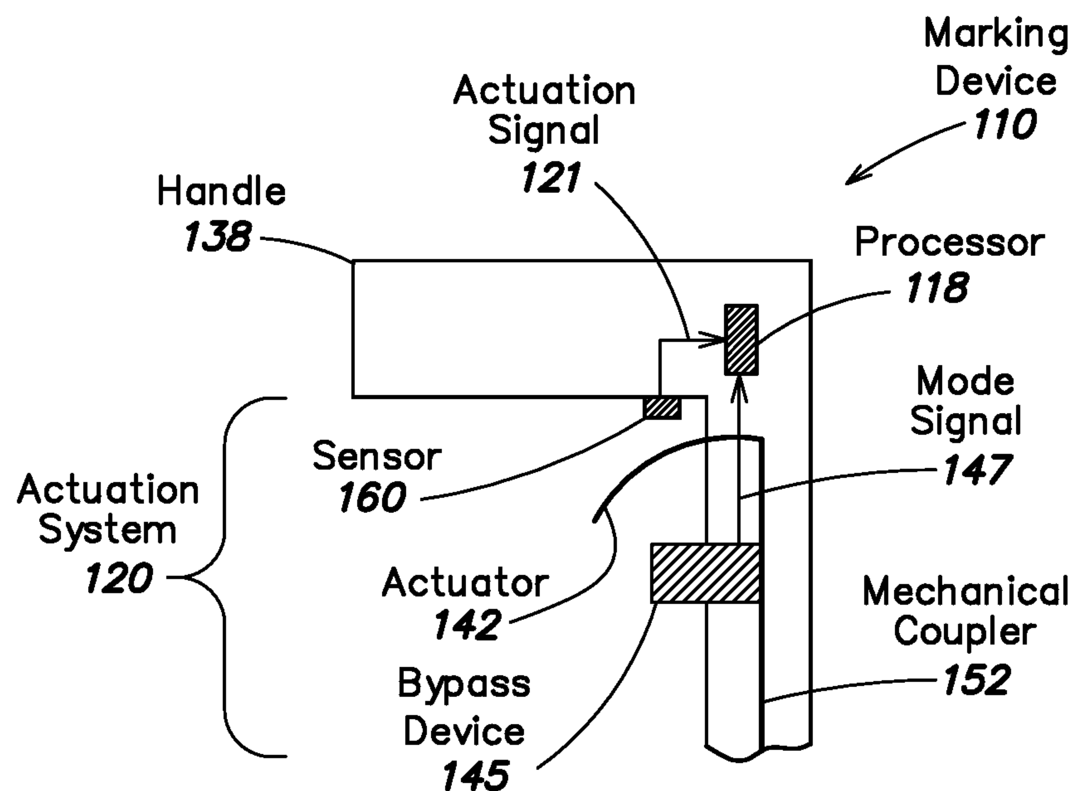
FIG. 11A
