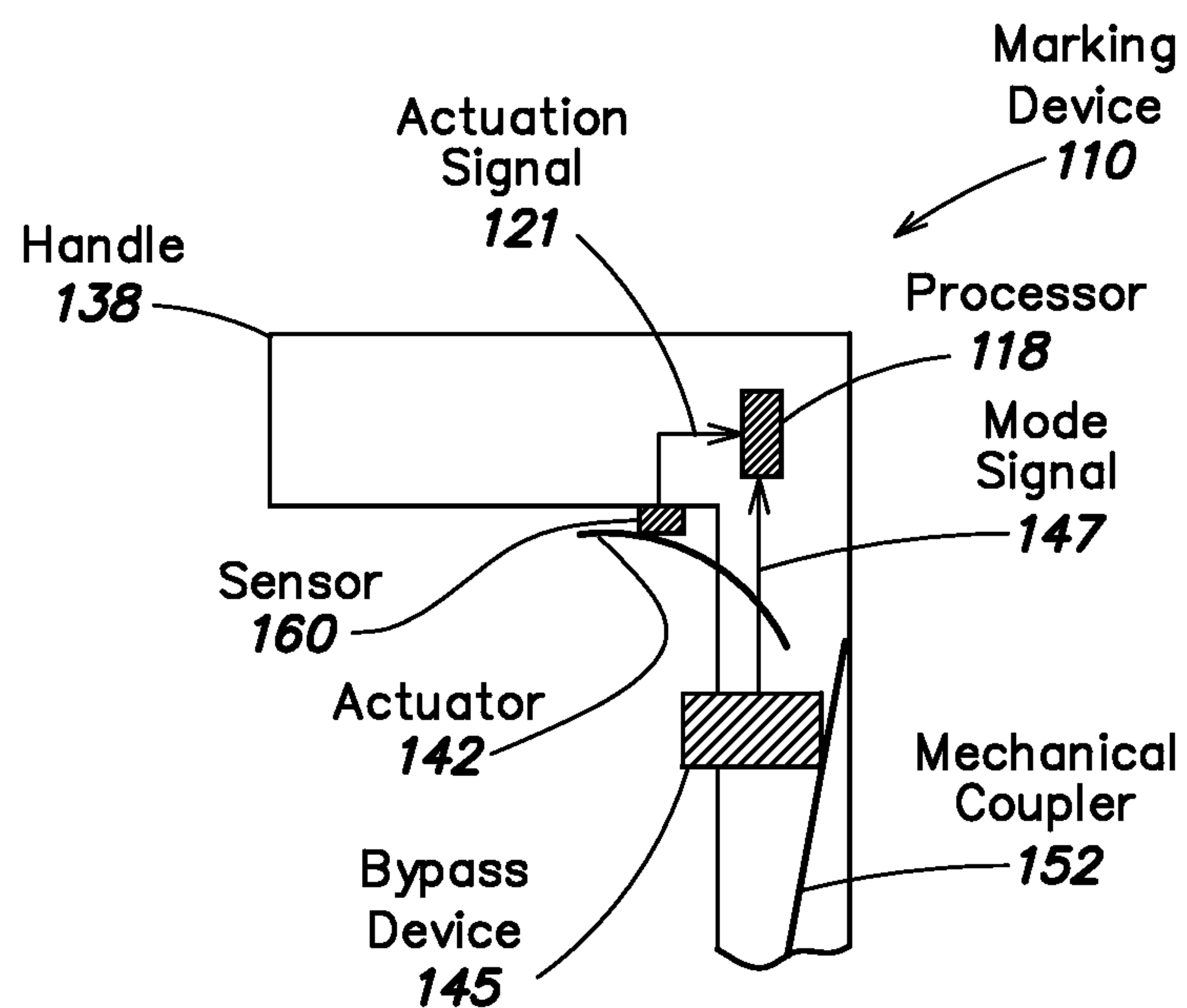
FIG. 11B
