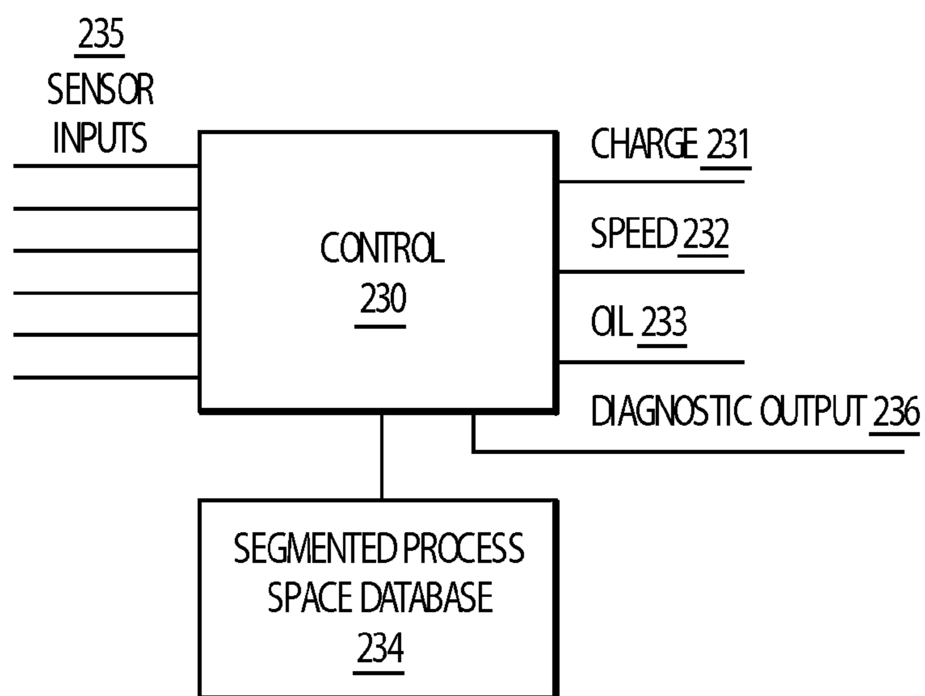
FIG. 7C
