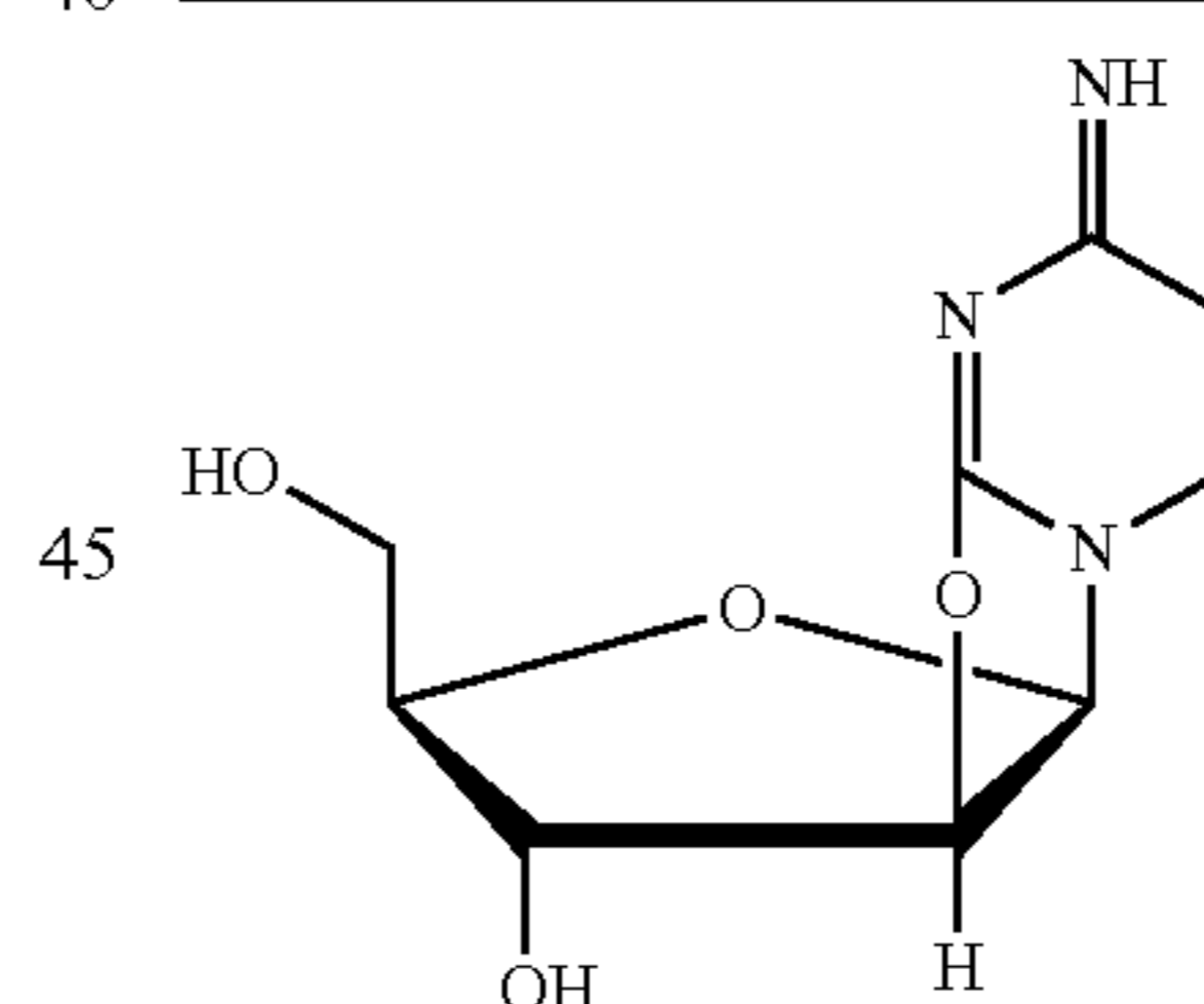
Ancitabine
