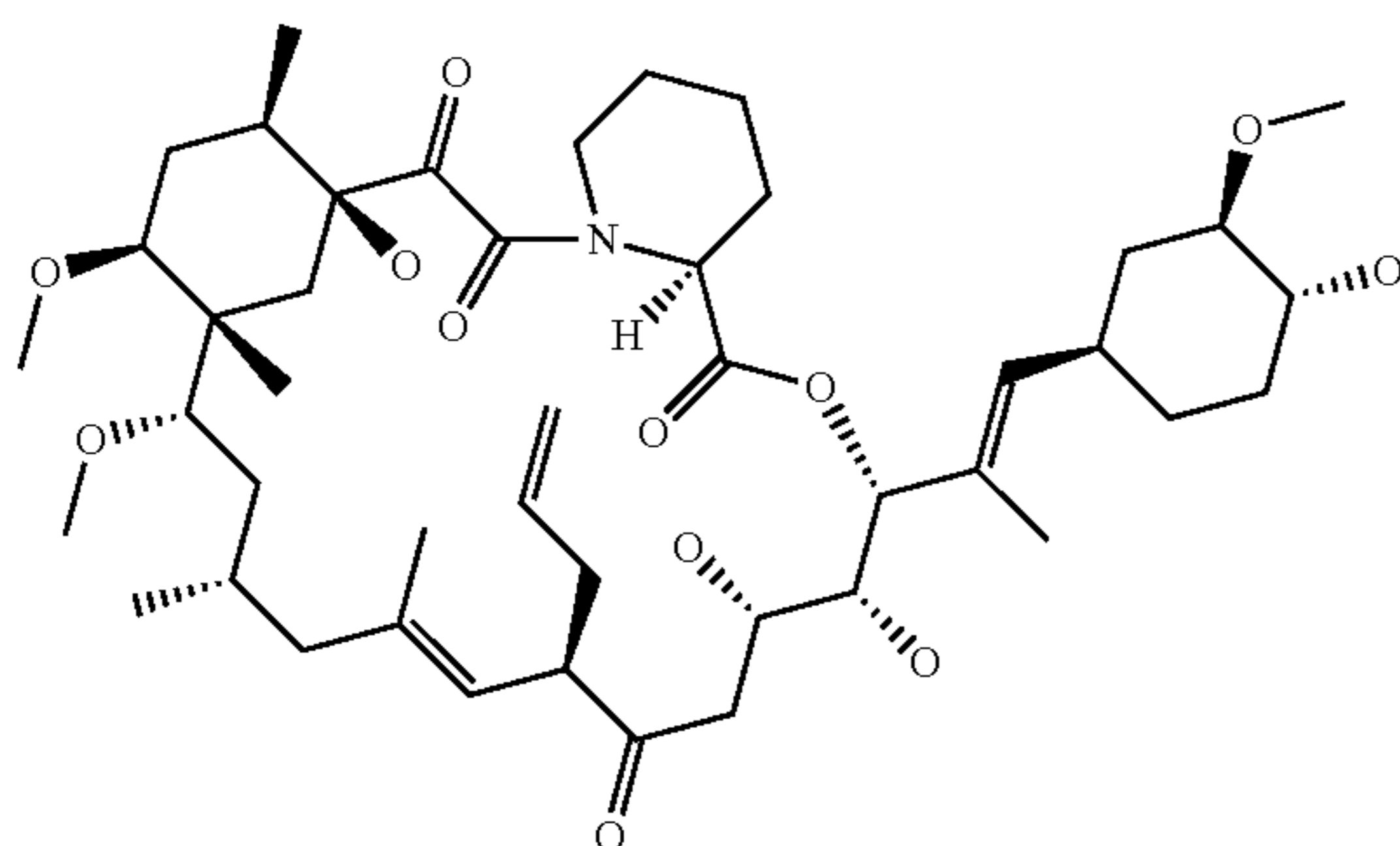
Tacrolimus
