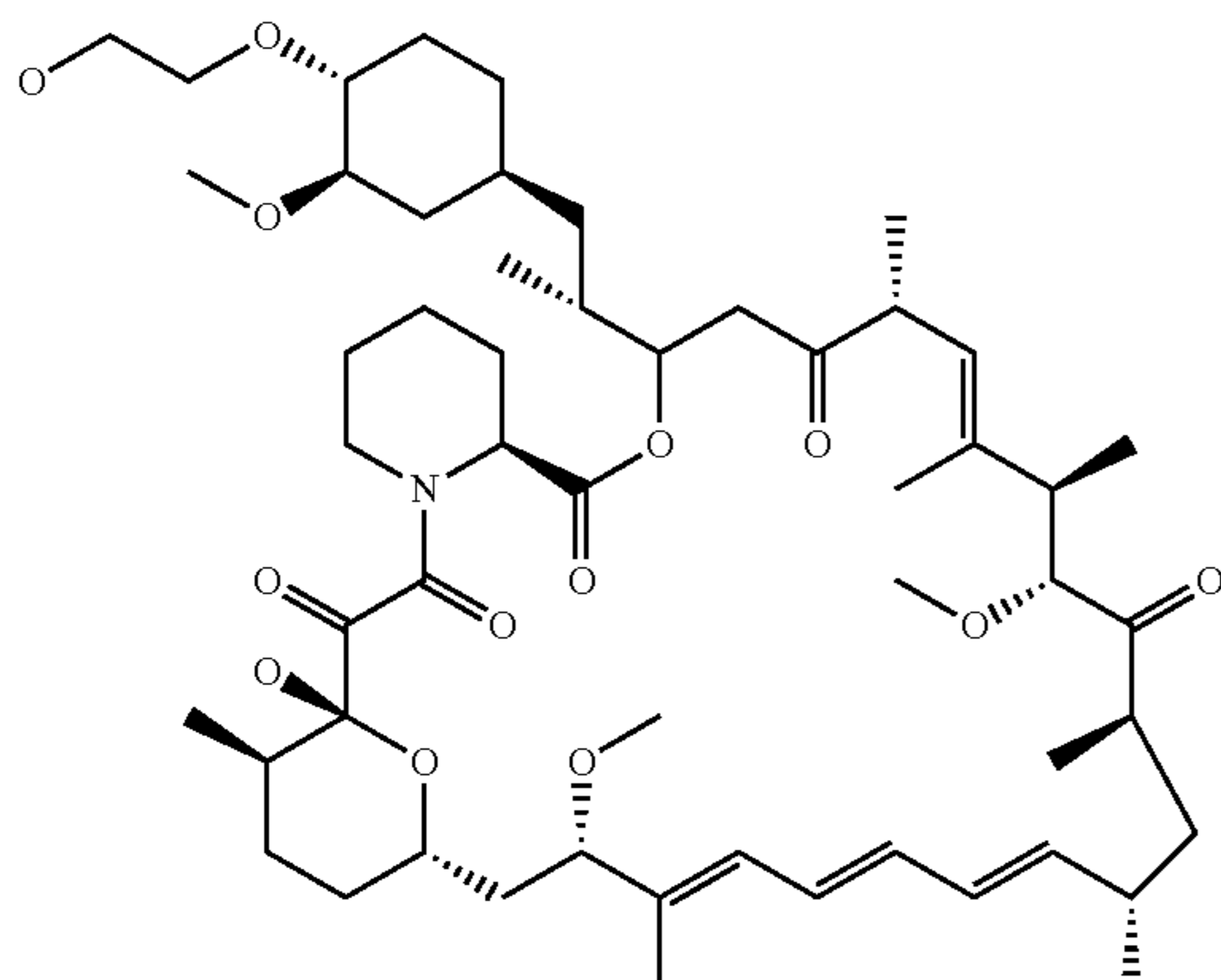
Everolimus
