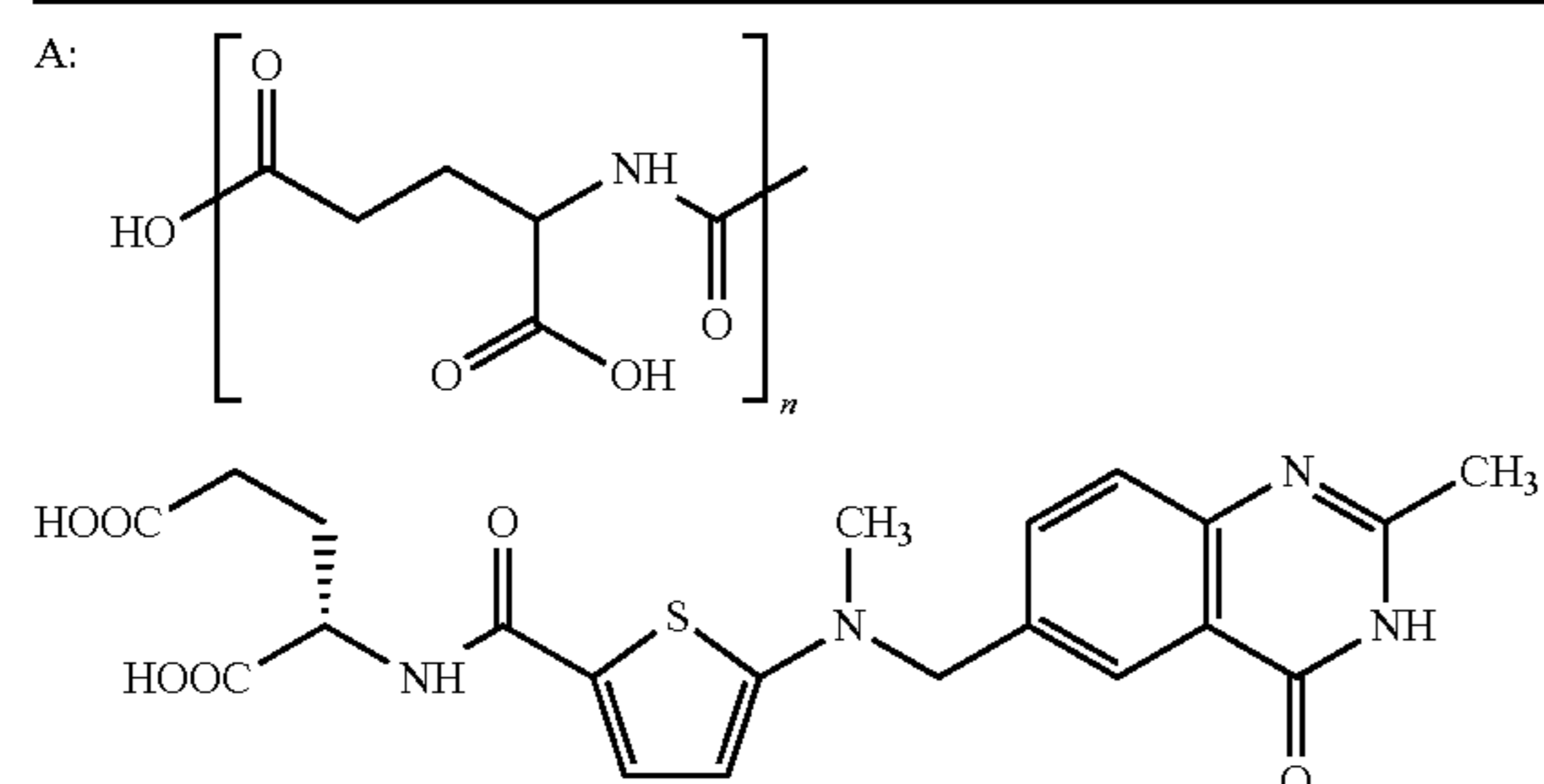
(XXI) Tomudex
