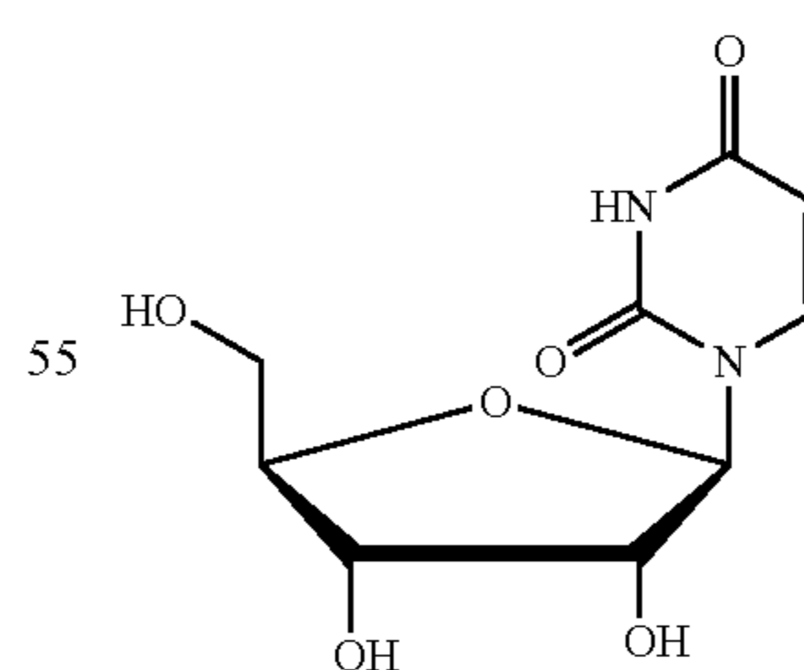
6-Azauridine
