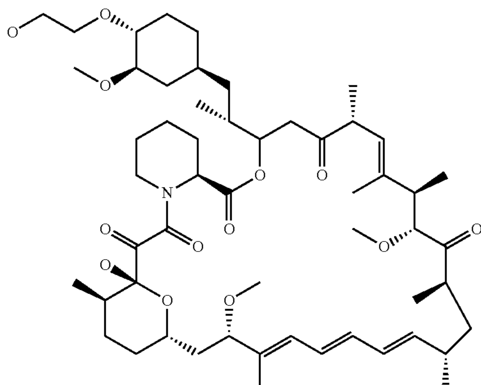
Everolimus
