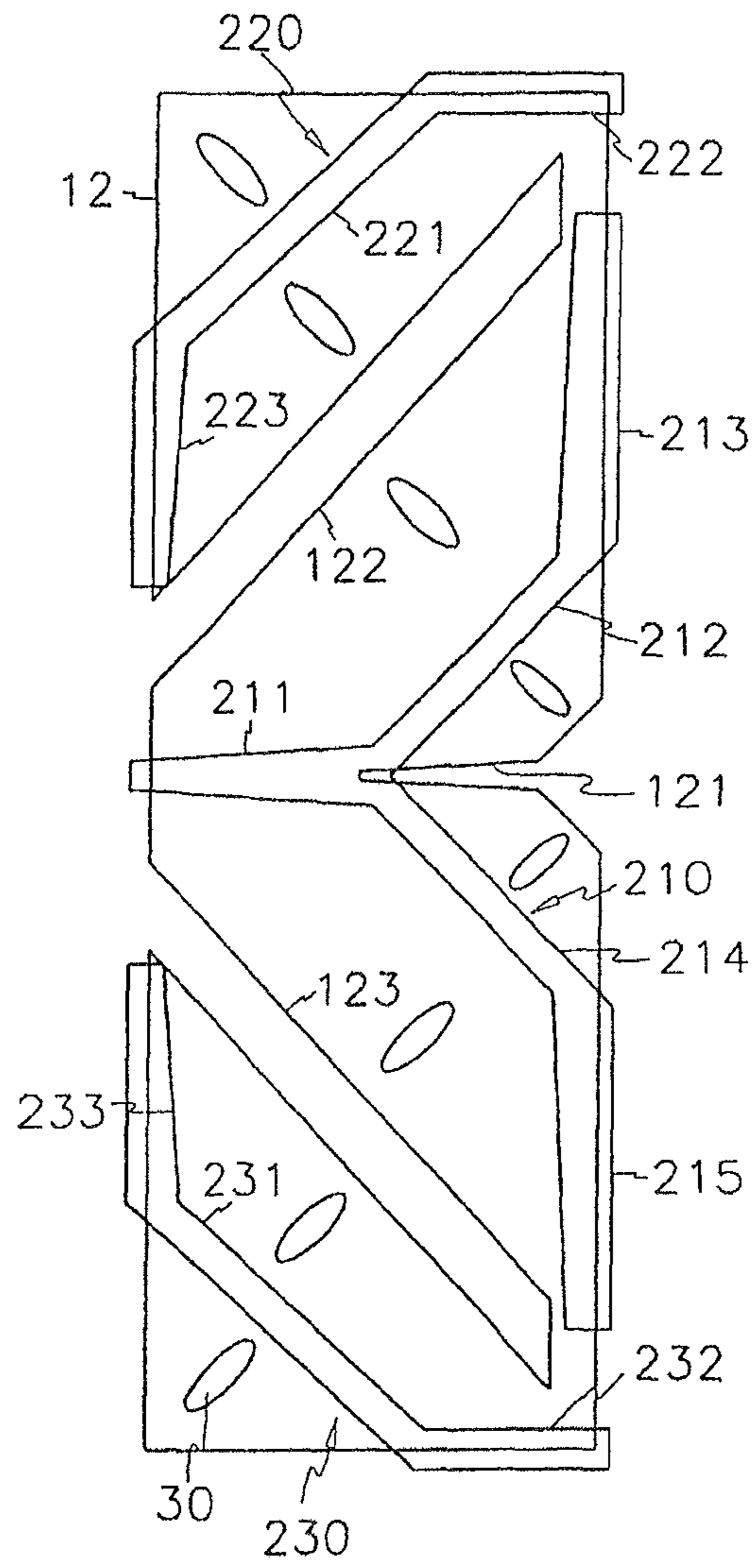
FIG. 4C
